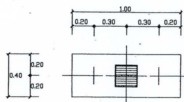
PLAN F2
