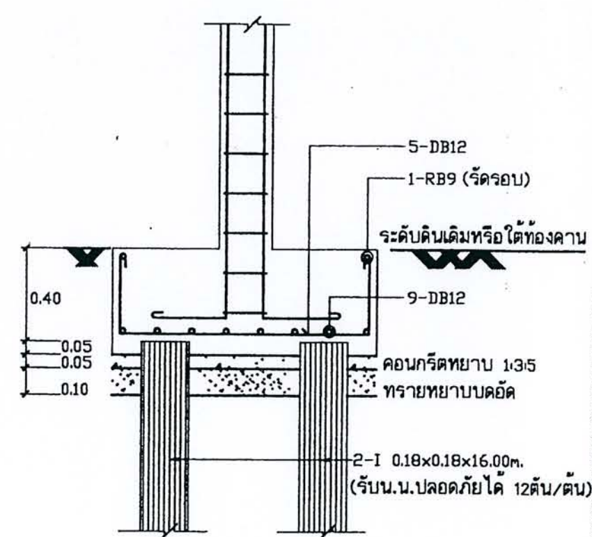
SECTION F2 1:20
