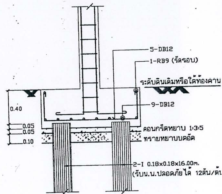
SECTION F2 1:20
