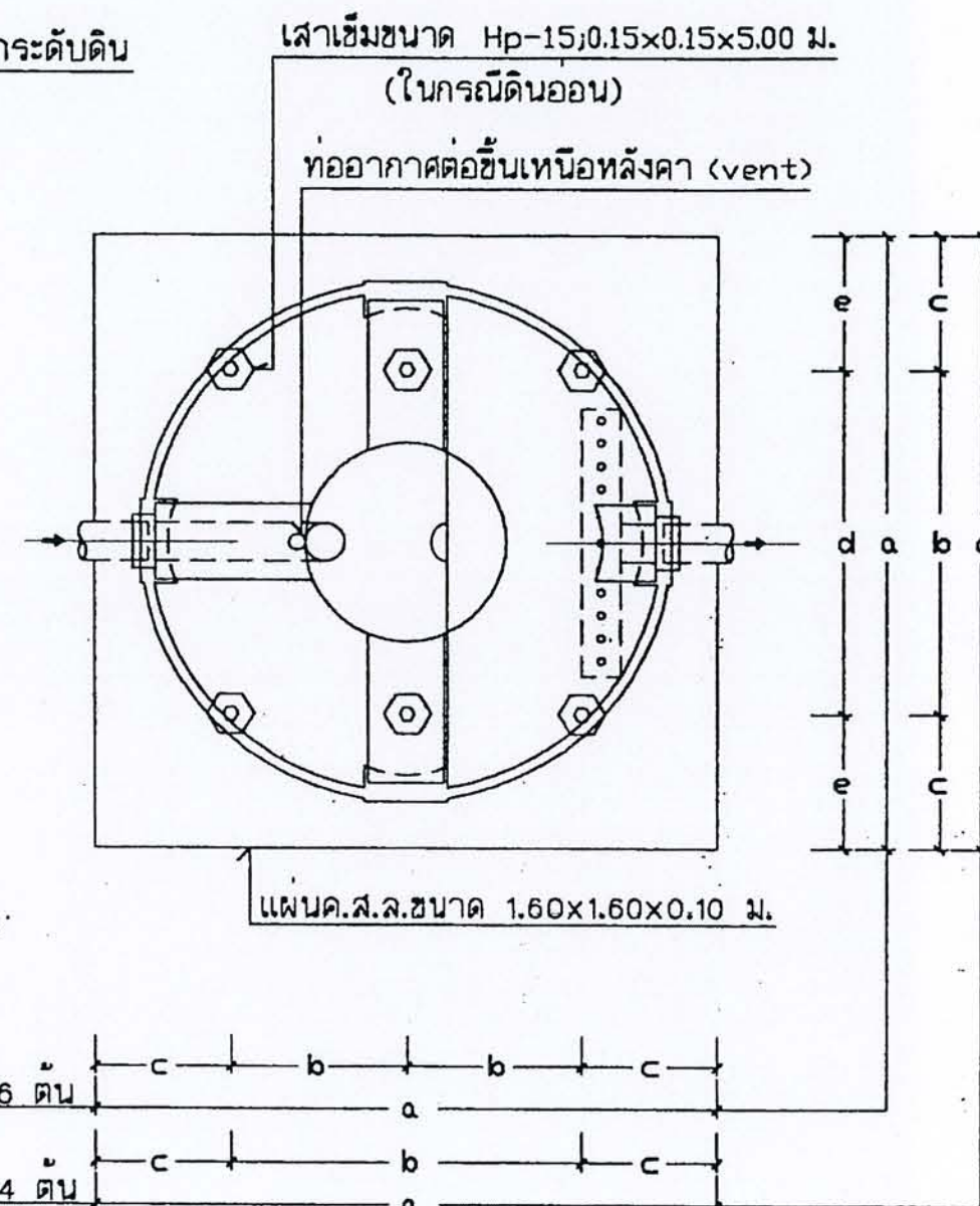
PLAN 1:20
