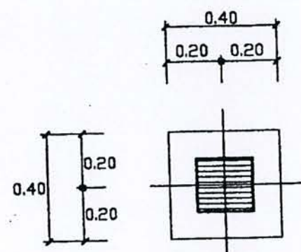
PLAN F1
