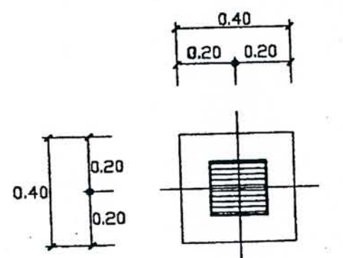
PLAN F1A
