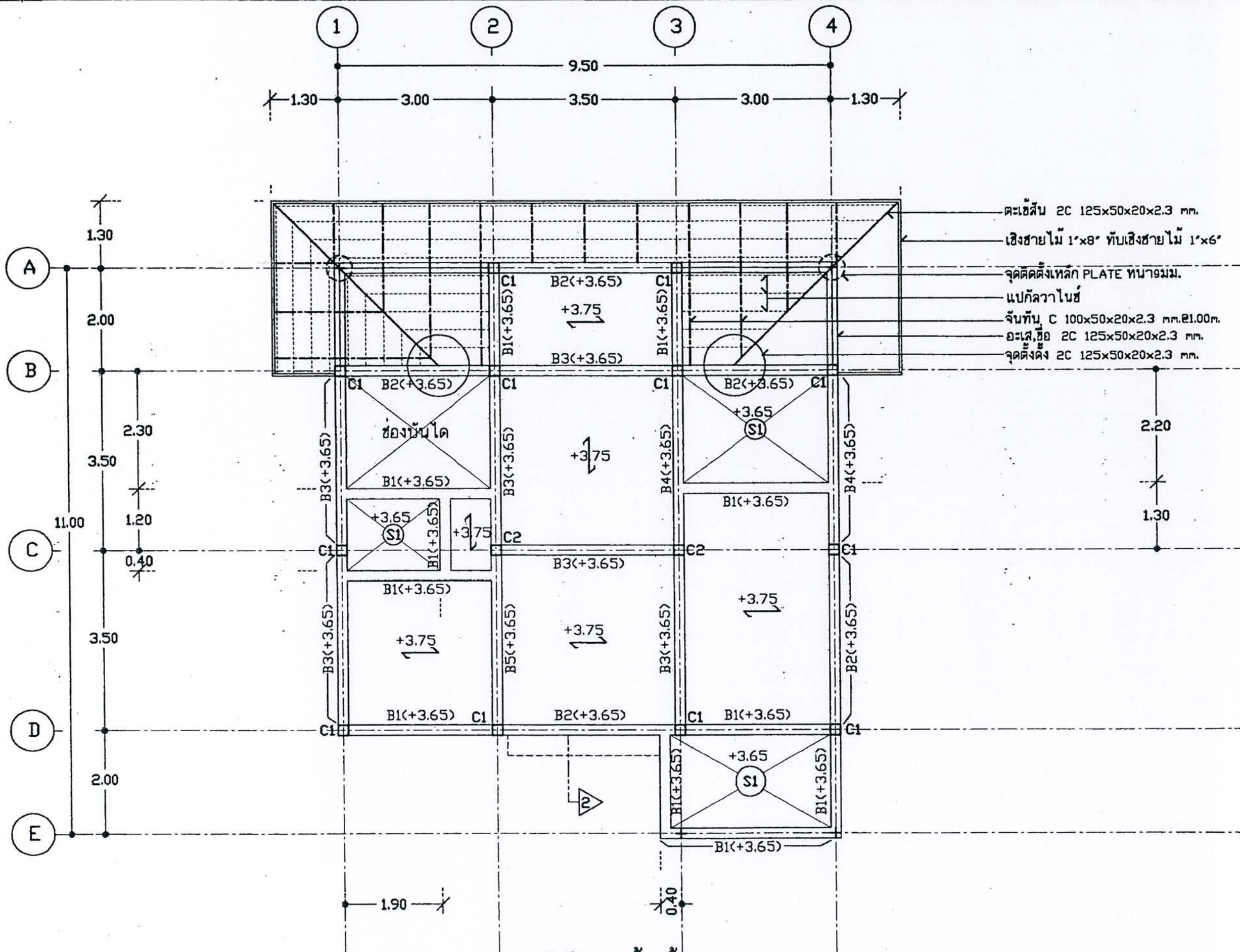
ผังโครงสร้างชั้นบน มาตราส่วน 1:75
