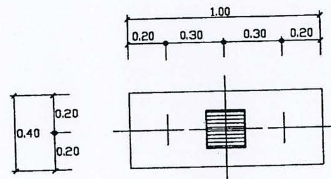
PLAN F2
