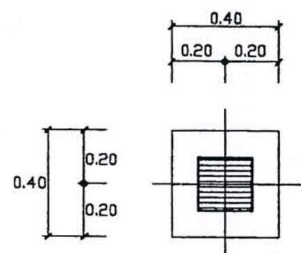
PLAN F1A
