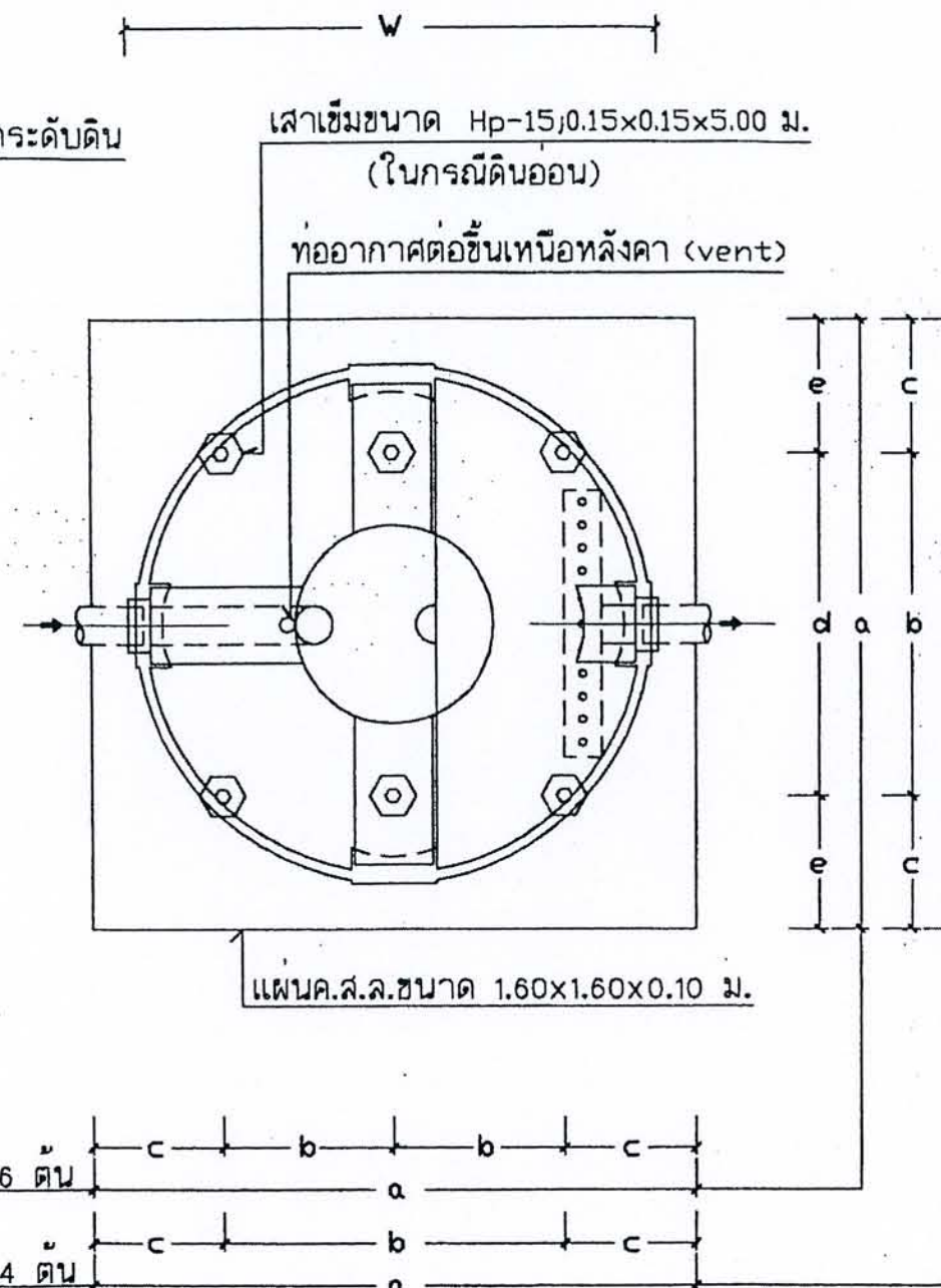
PLAN 1:20
