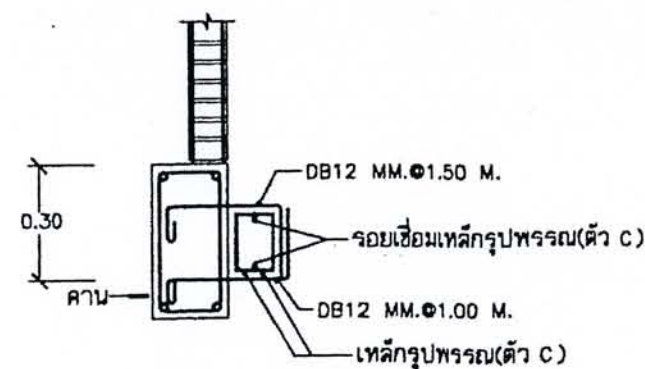
แบบขยายจุดที่มีหลังคาครอบวางติดผนัง
