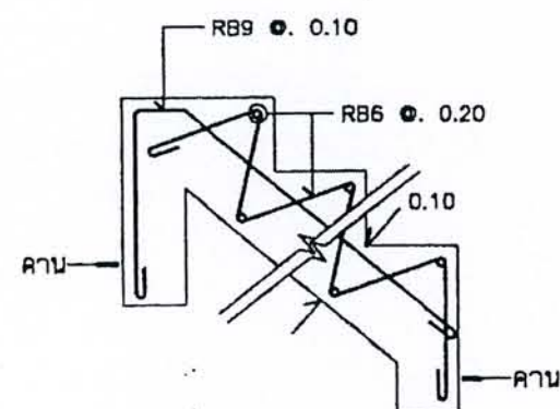
SECTION - 2 (ตามแบบโครงสร้างชั้นล่าง)
