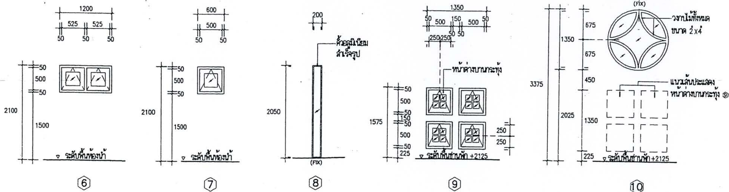
แบบขยายหน้าต่าง มาตราส่วน 1 : 50
