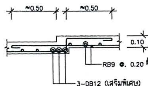
ขยายพื้นลดระดับ
