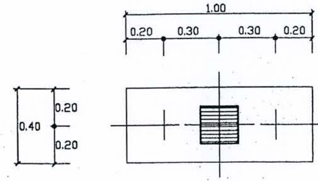
PLAN F2
