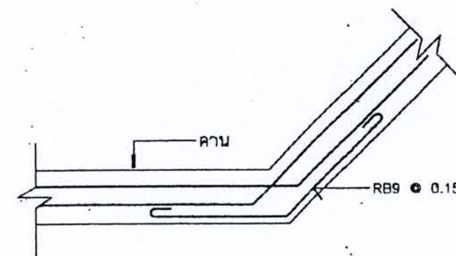
(แสดงการเดินเหล็กคานช่วงมุม)
