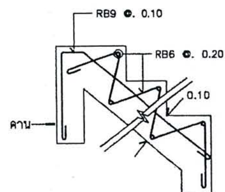
SECTION - 1 (ตามแบบโครงสร้างชั้นล่าง)
