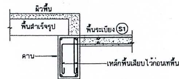
แบบขยายรอยต่อพื้นที่กับระเบียง
