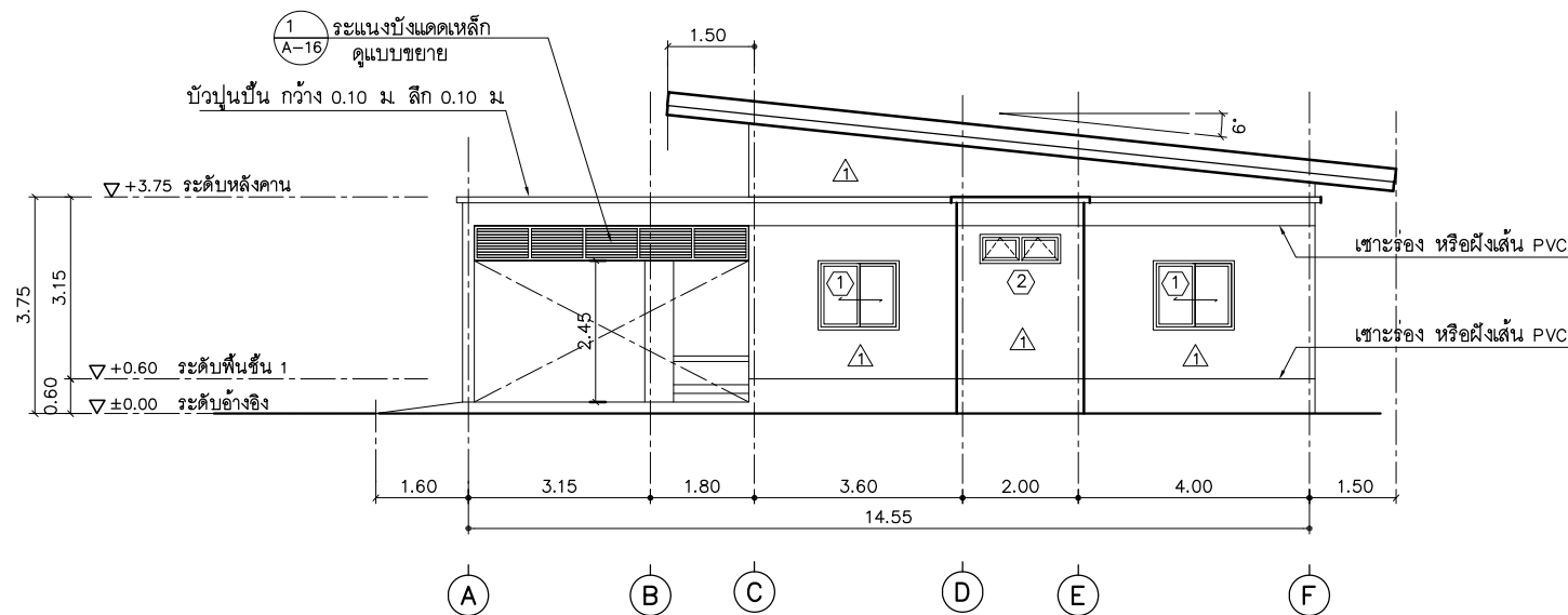
รูปด้าน 4
