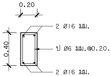
B1 1:20
