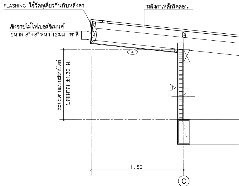
แบบขยาย เเชิงชาย 1 มาตราส่วน 1:25
