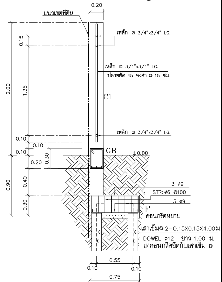
รูปตัด
