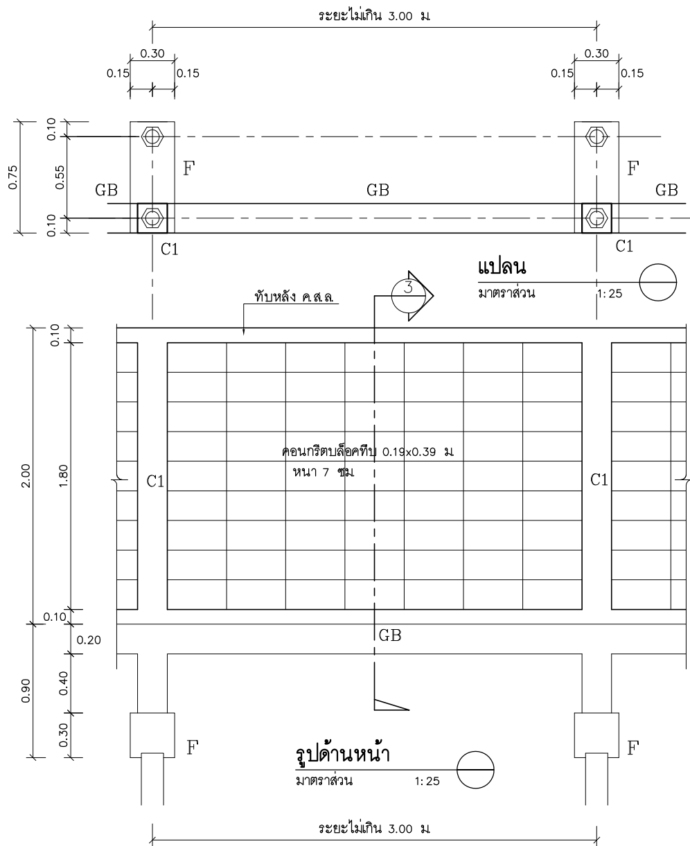
แบบขยายรูปแบบที่ 2
