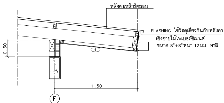
แบบขยาย เเชิงชาย 2 มาตราส่วน 1:25
