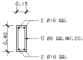
RB1A 1:20
