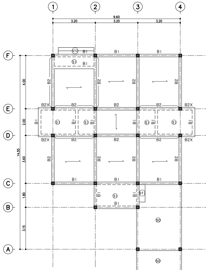
แปลนคาน, พื้นชั้น 1 มาตราส่วน 1:100
