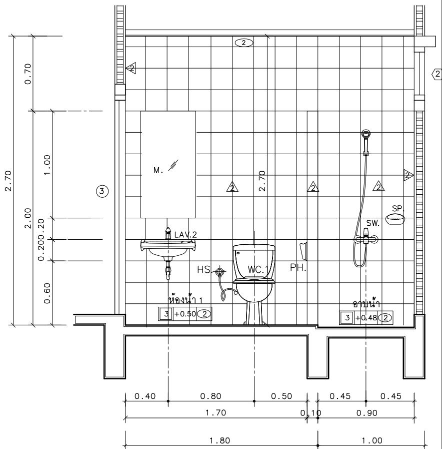
รูปตัดห้องน้ำ WC.1
