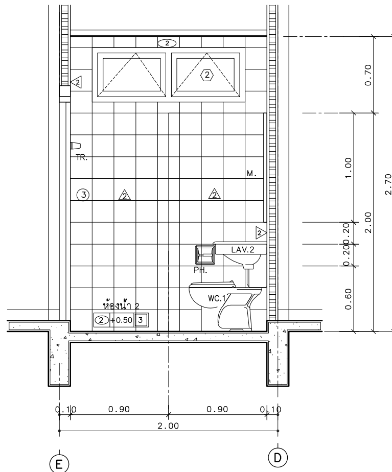
รูปตัดห้องน้ำ WC.2
