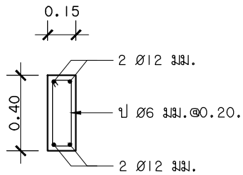
RB1 1:20
