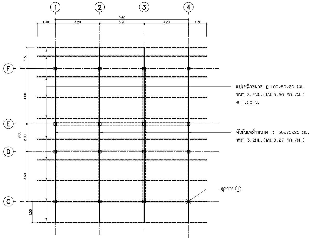
แปลนโครงสร้าง มาตราส่วน 1:100
