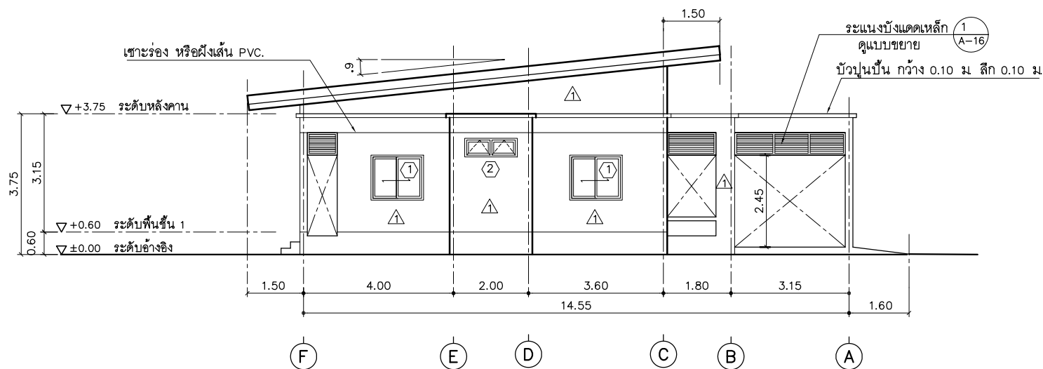
รูปด้าน 2
