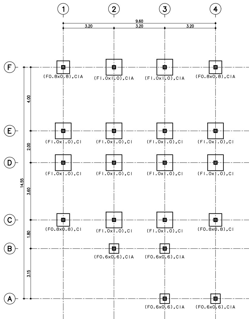
แปลนฐานรากแผ่ มาตราส่วน 1:100
