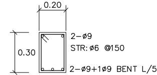
ขยายคานคอดิน
