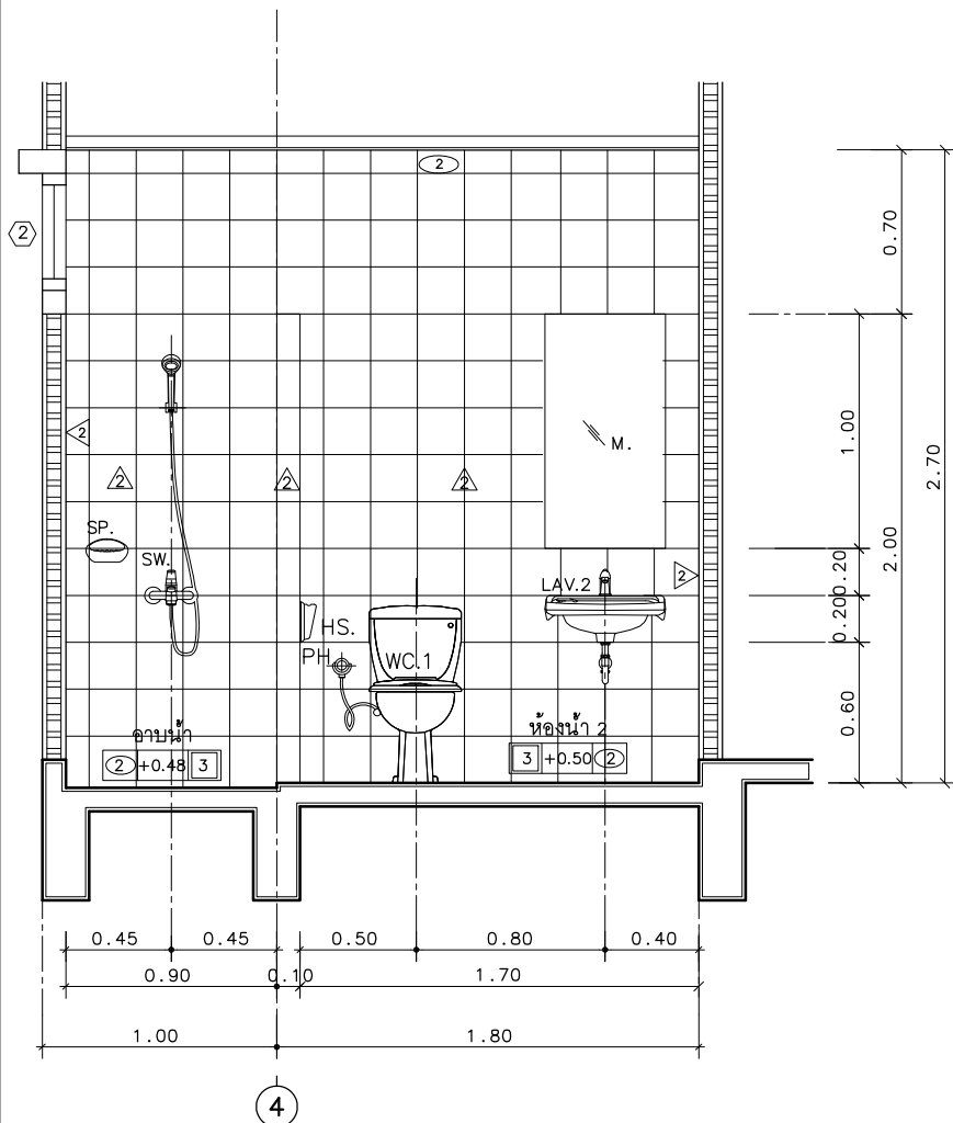
รูปตัดห้องน้ำ WC.2
