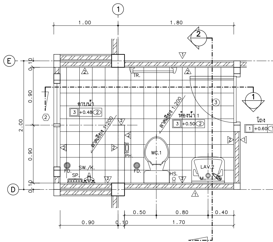
แปลนห้องน้ำ WC.1
