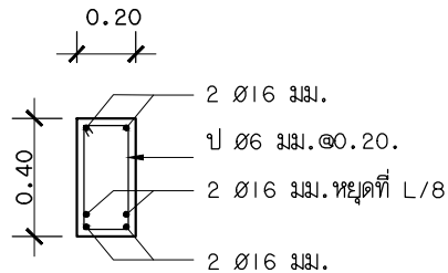
B2 1:20
