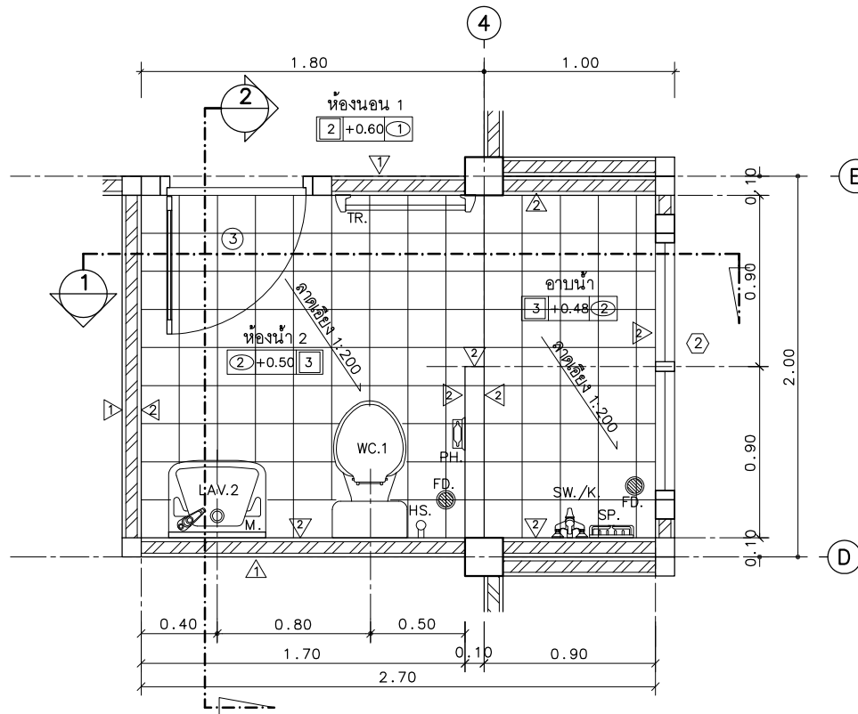
แปลนห้องน้ำ WC.2
