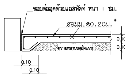
S0 1:20
