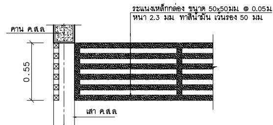
แบบขยาย ระแนงบังแดดเหล็ก มาตราส่วน 1:25
