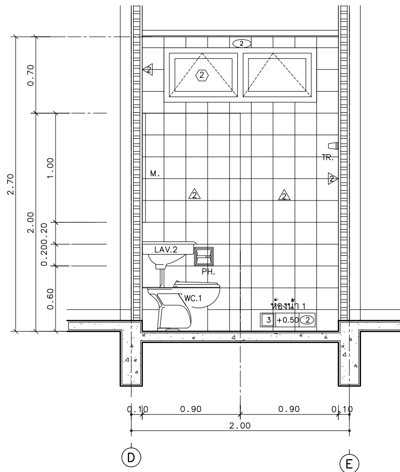
รูปตัดห้องน้ำ WC.1
