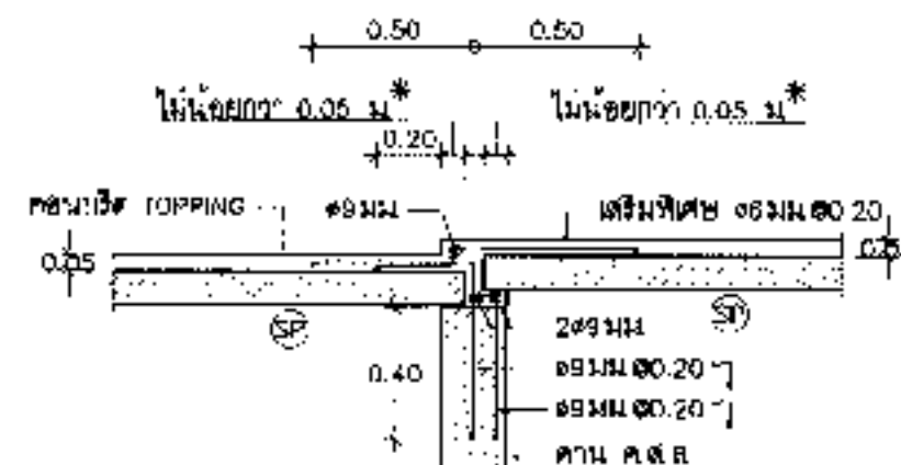
กรณียกระดับพื้นสำเร็จทางระดับกัน
