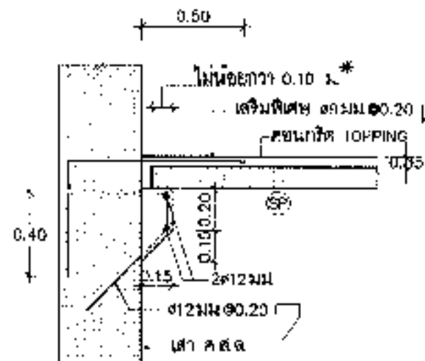
ลักษณะการวางพื้น (SP) บริเวณเสาหรือคานที่ไม่มีที่รองรับ
