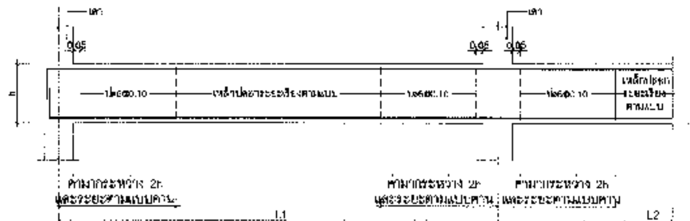
รายละเอียดการเสริมเหล็กระยะเรียงของเหล็กปลอกในคาน (TYP.) เพื่อคำนวณการดึงเส้นของแผ่นดินไหวบริเวณ 3
