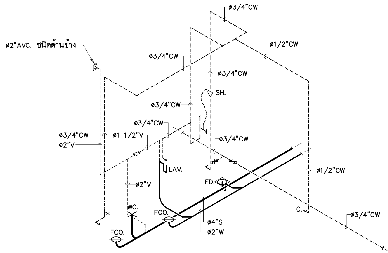
ไอโซเมตริกระบบสุขาภิบาลห้องน้ำ
