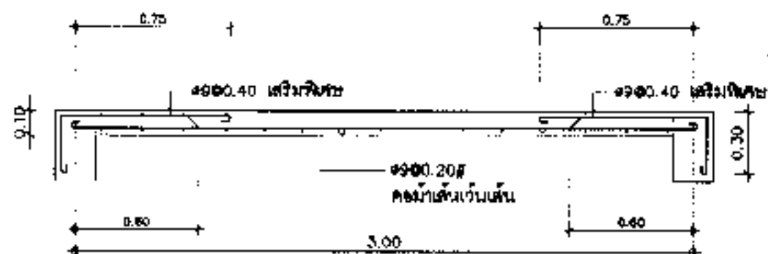
S1 (ด้านยาว) ขนาดจริง 1 : 25
