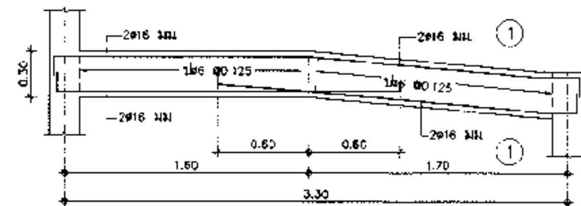
B1 ขนาดหน้าตัด 1 : 25
