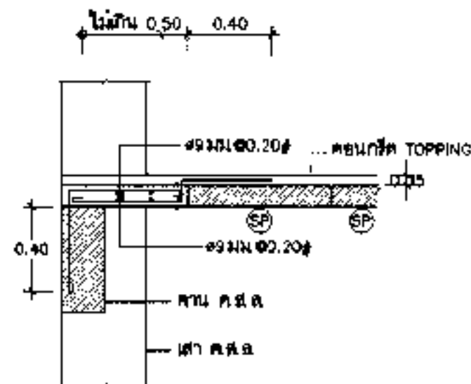
ลักษณะการหล่อพื้นเสริมเกร็ดเสริมช่องว่างที่คานริม
