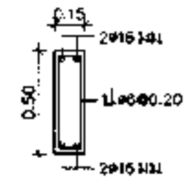
B3 ขนาดหน้าตัด 1 : 25
