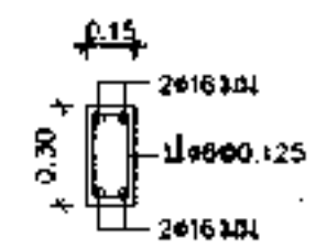
B5 ขนาดหน้าตัด 1 : 25
