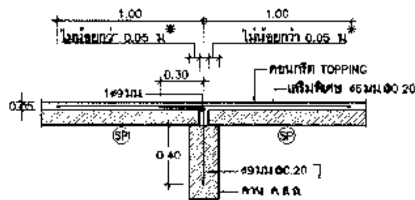
ลักษณะการวางพื้น (SP) ภายใน
