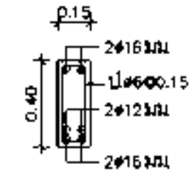
B2 ขนาดหน้าตัด 1 : 25
