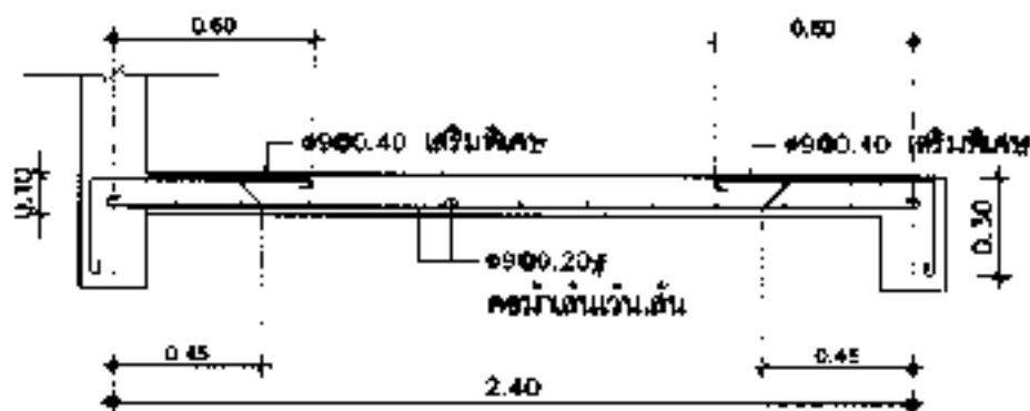
S1 (ด้านสั้น) ขนาดจริง 1 : 25
