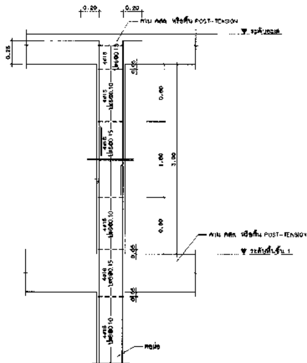
รายละเอียดของระยะห่างของเหล็กในเสา (TYP.) เพื่อกำหนดการเสริมเหล็กของแผ่นดินไหวบริเวณ 3
