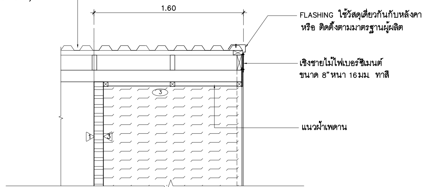
แบบขยายหลังคา มาตราส่วน 3 A-15
