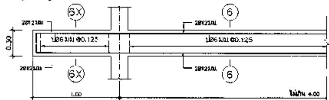
B6, B6X ขนาดหน้าตัด 1 : 25
