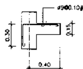
SX ขนาดจริง 1 : 25
