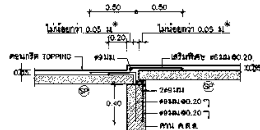
กรณียกกระดานพื้นต่ำไว้ต่างระดับกัน
