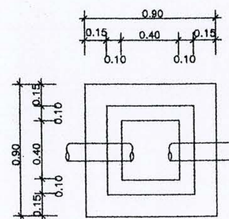
แปลนขยายบ่อพัก
