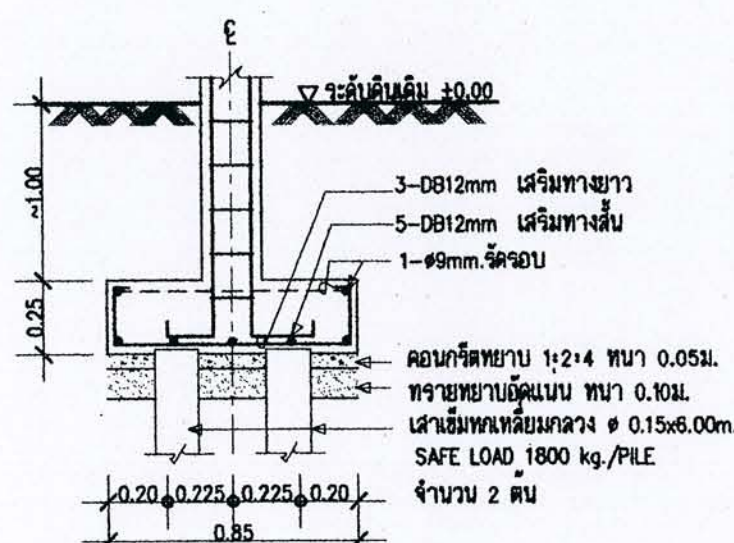
รูปตัด F1
