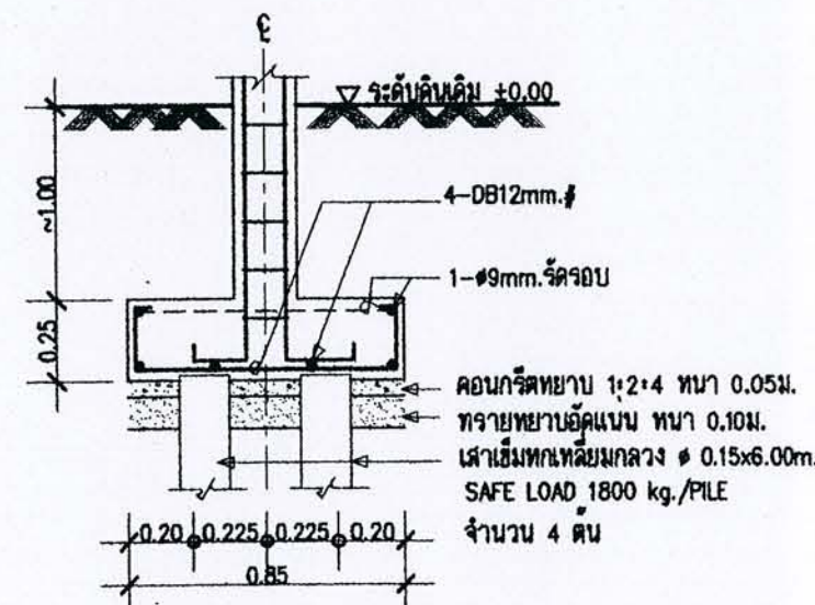
รูปตัด F2
