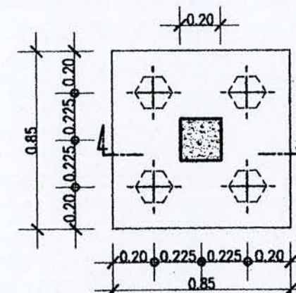
แบบขยาย F2
