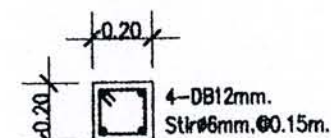
C1 ฐานราก - ทิ้งค่า
