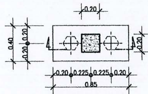
แบบขยาย F1
