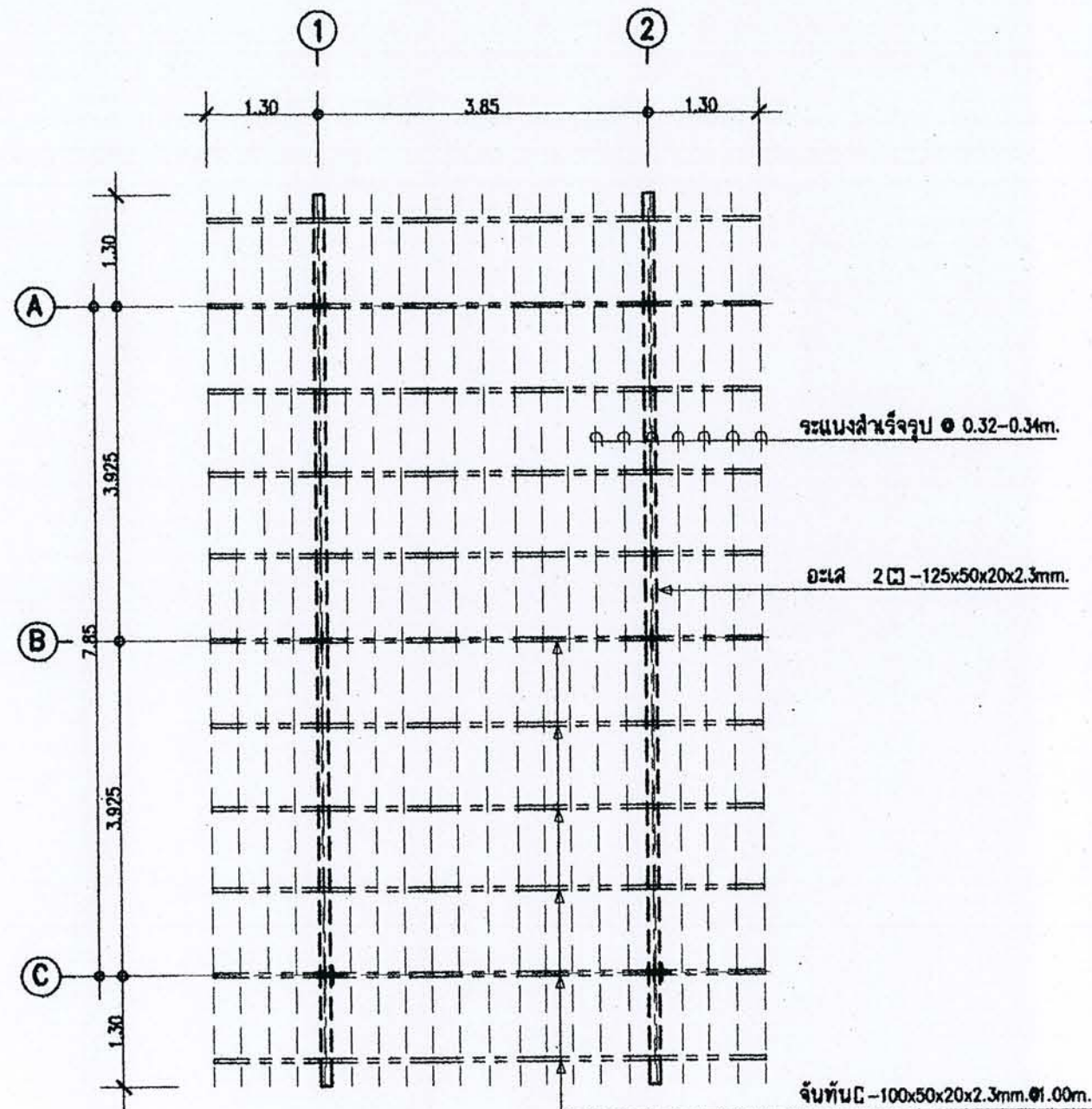
แปลนคานและโครงหลังคา
