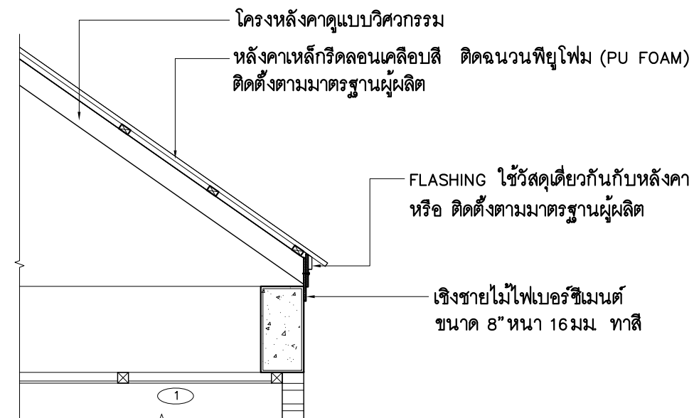
แบบขยายหลังคา
