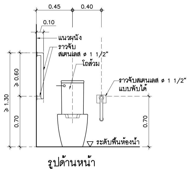
แบบขยายราวจับโถส้วมคนพิการ
