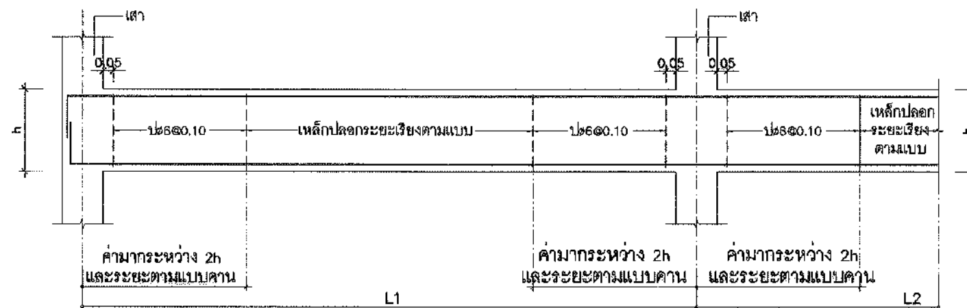
รายละเอียดการเสริมเหล็กของเหล็กปลอกในคาน (TYP.) เพื่อดำเนินการสันสีเทือนของแผ่นดินไหวบริเวณ 1 และ 2
