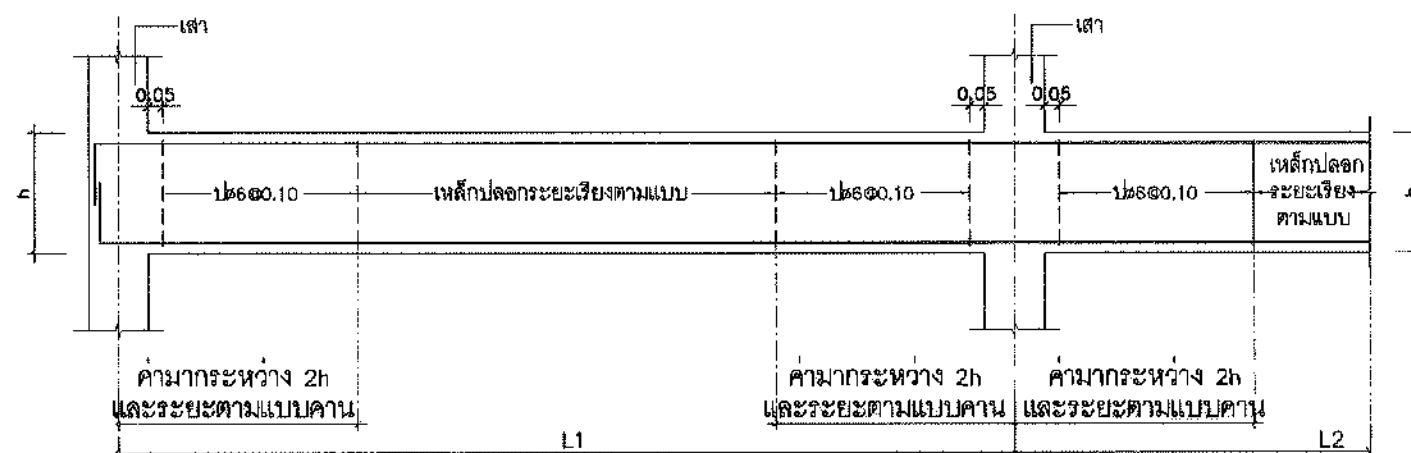
รายละเอียดการเสริมเหล็กระยะเรียงของเหล็กปลอกในคาน (TYP.) เพื่อคำนวณการสันสะท้อนของแผ่นดินไหวบริเวณ 3
