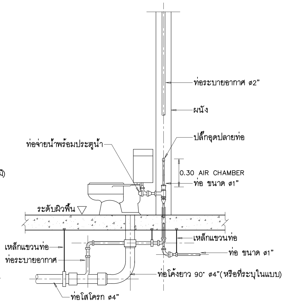
ส้วมชนิดถังน้ำล้าง (FLUSH TANK)
