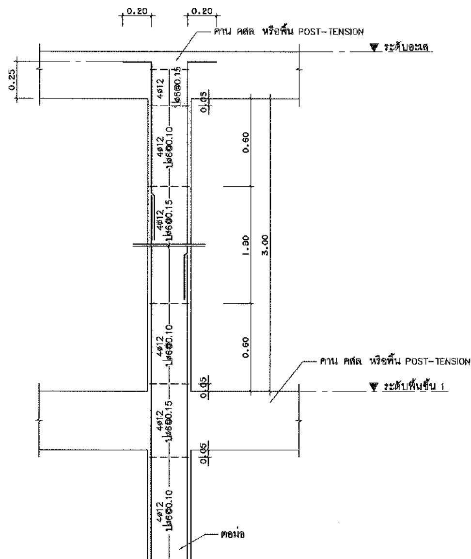
รายละเอียดระยะเรียงของเหล็กในเสา (TYP.) เพื่อดำเนินการสันสีเทือนของแผ่นดินไหวบริเวณ 1 และ 2
