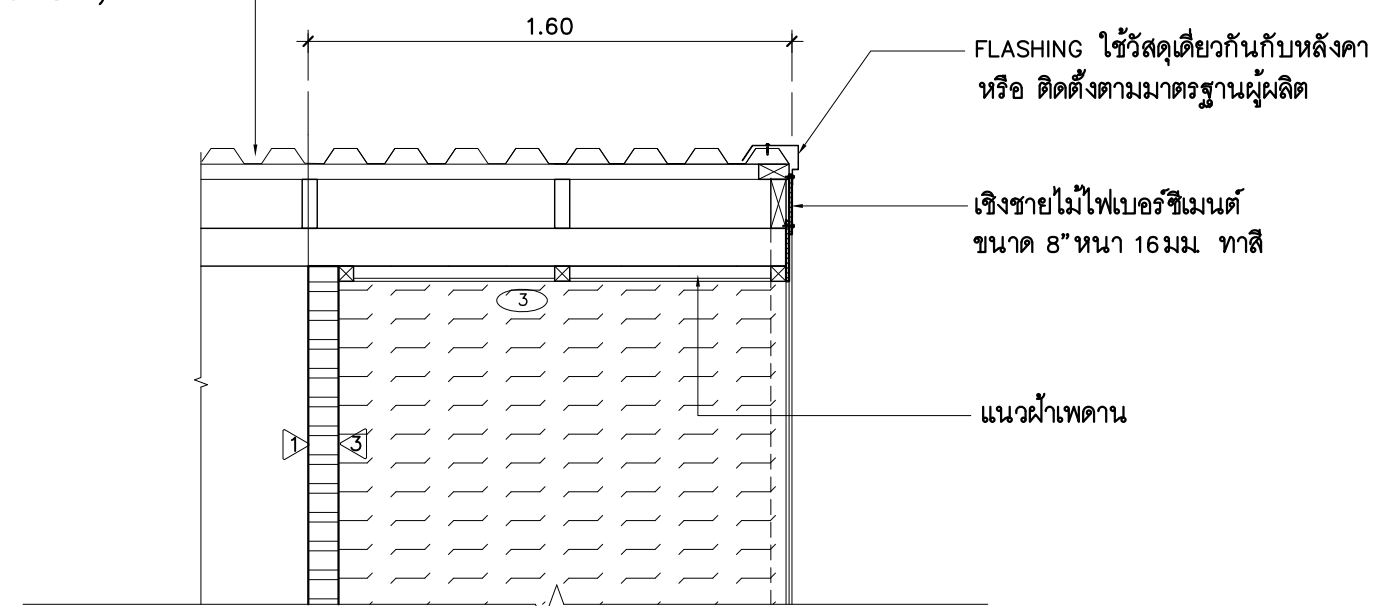
แบบขยายหลังคา
