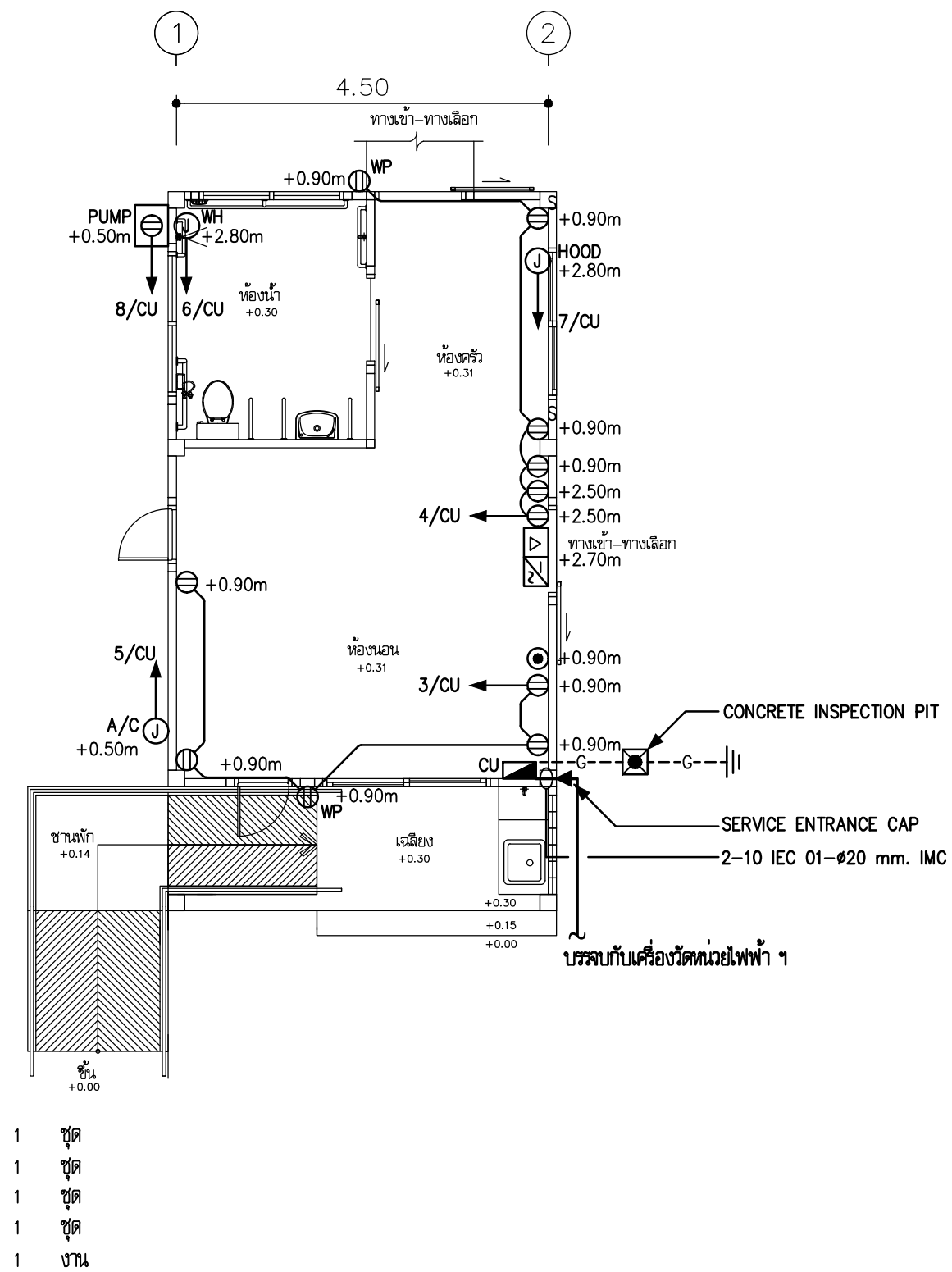
ผังระบบเดินรับไฟฟ้าและระบบเดินรับทีวี 1 : 75
