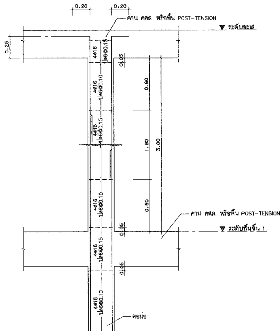
รายละเอียดระยะเรียงของเหล็กในเสา (TYP.) เพื่อคำนวณการสันสะท้อนของแผ่นดินไหวบริเวณ 3
