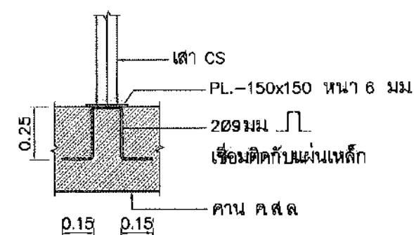
ขยายรอยต่อเสา CS กับคาน ค.ส.ล.
