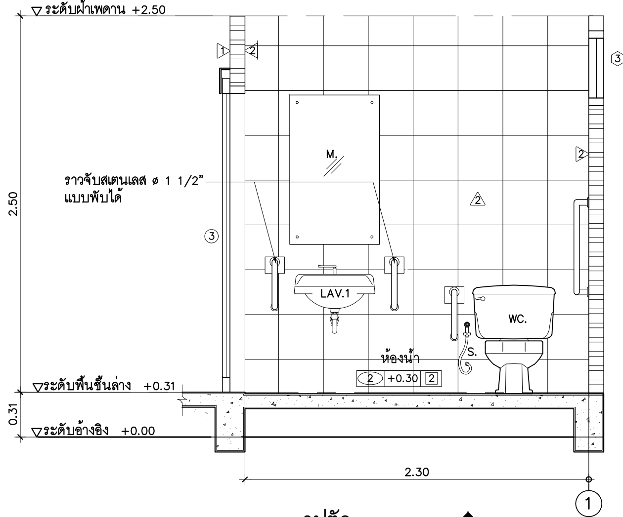
รูปตัด มาตราส่วน 1 : 25 A-10
