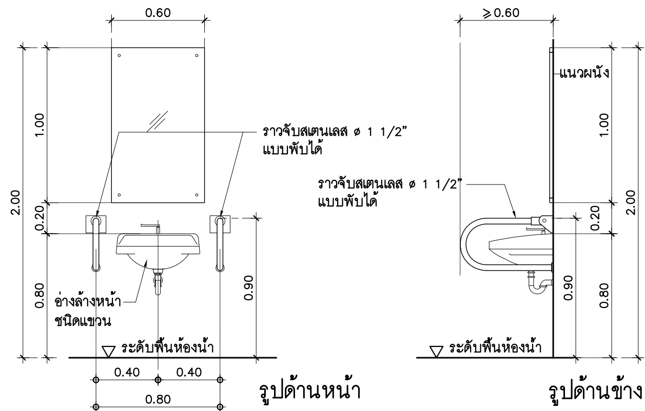
แบบขยายราวจับอ่างล้างหน้าคนพิการ
