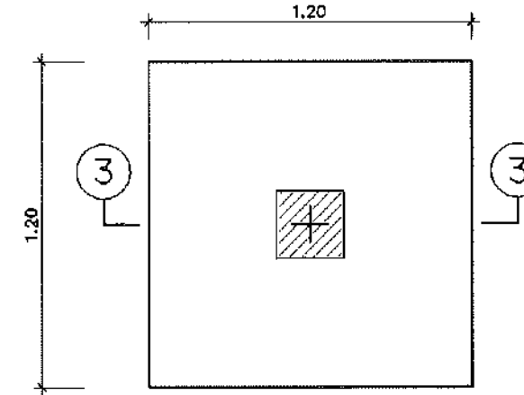
F 1.20x1.20 มาตรฐาน 1 : 25
