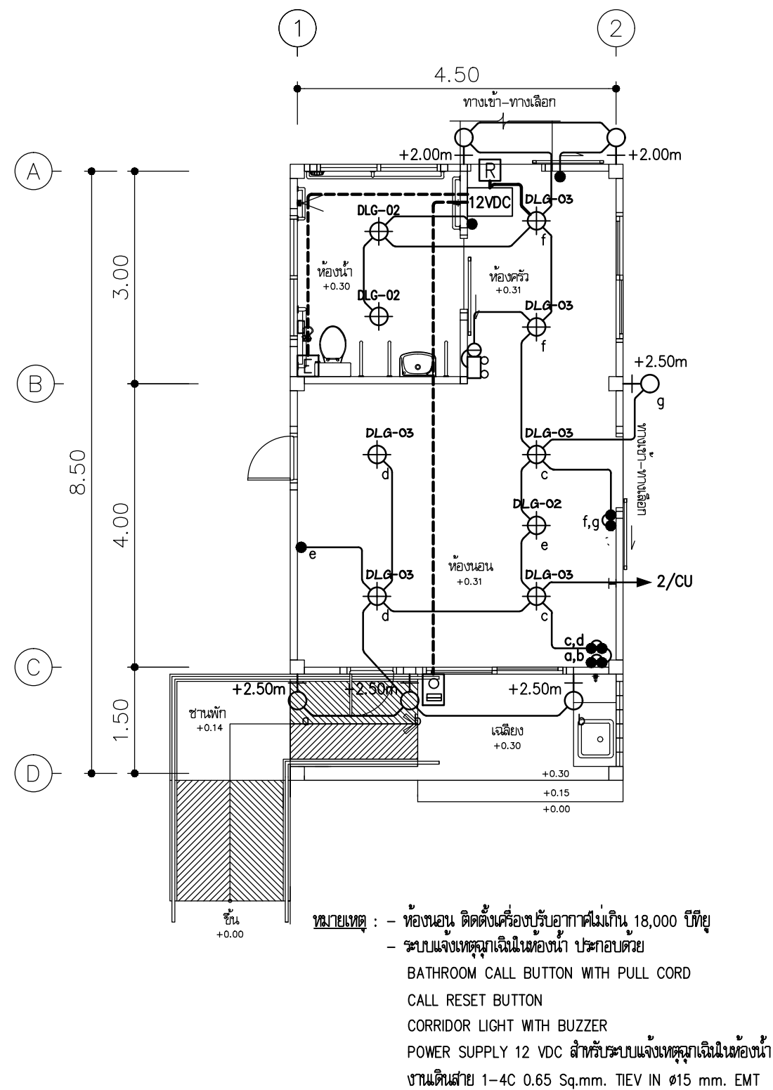
ผังระบบไฟฟ้าแสงสว่าง 1 : 75
