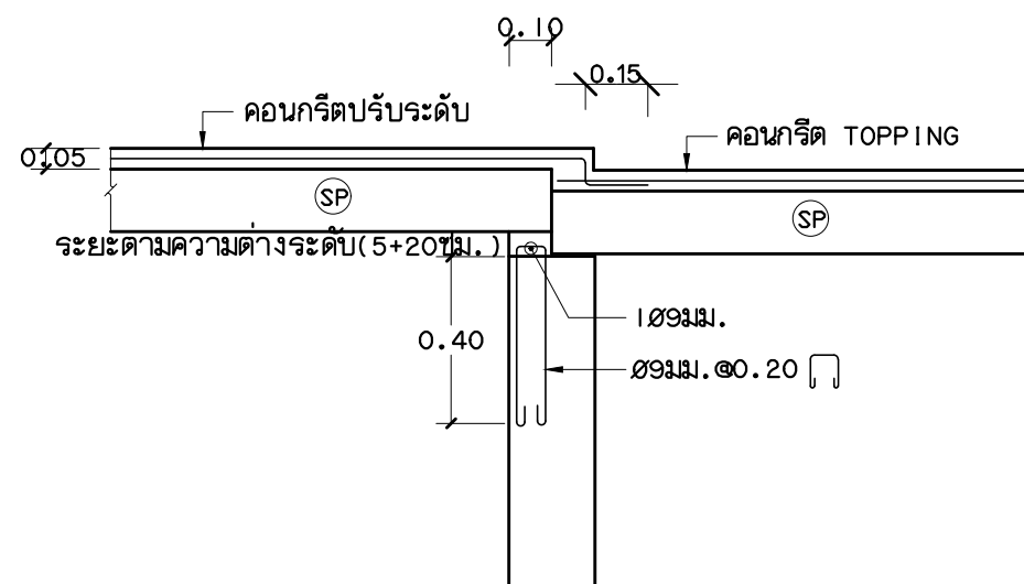
กรณียกกระดานพื้นสำเร็จต่างระดับกัน มาตราส่วน 1: 20
