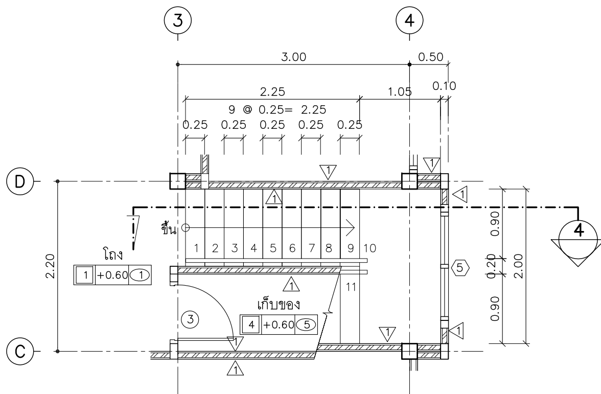
แปลนชั้น 1 บ้านไค ST.3
