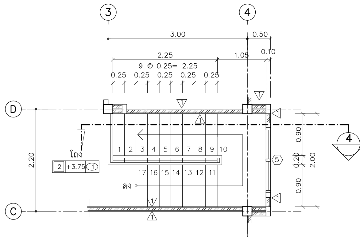
แปลนชั้น 2 บ้านไค ST.3
