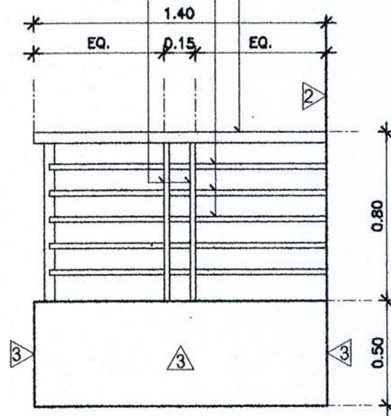
รูปด้าน 2
