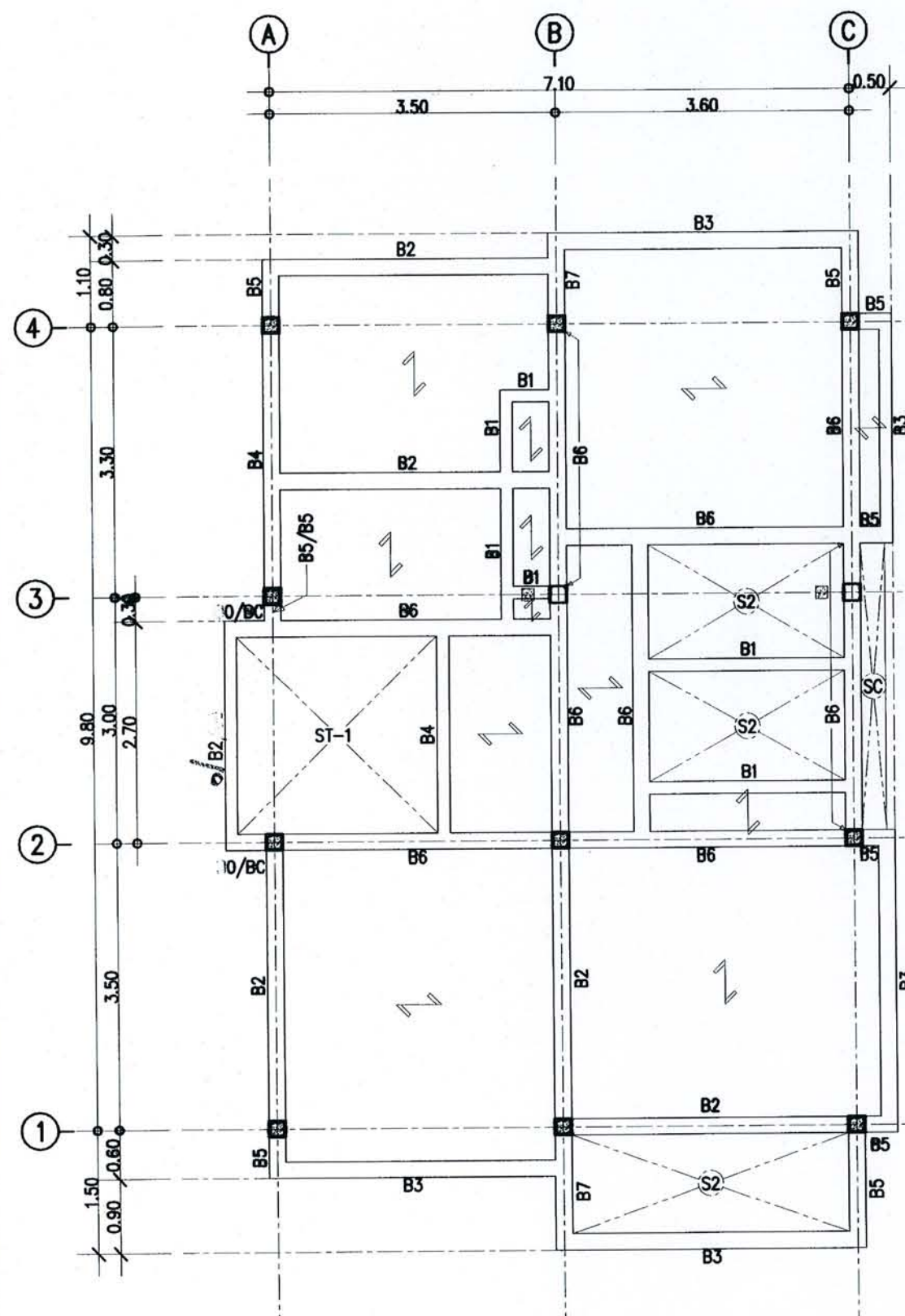
แปลนโครงสร้างชั้น 2 มาตราส่วน 1 : 75
