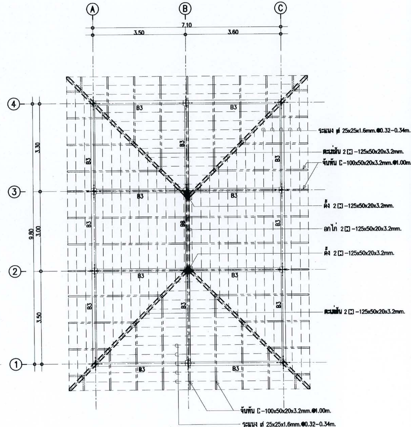
แปลนโครงสร้างหลังคา มาตราส่วน 1 : 75
