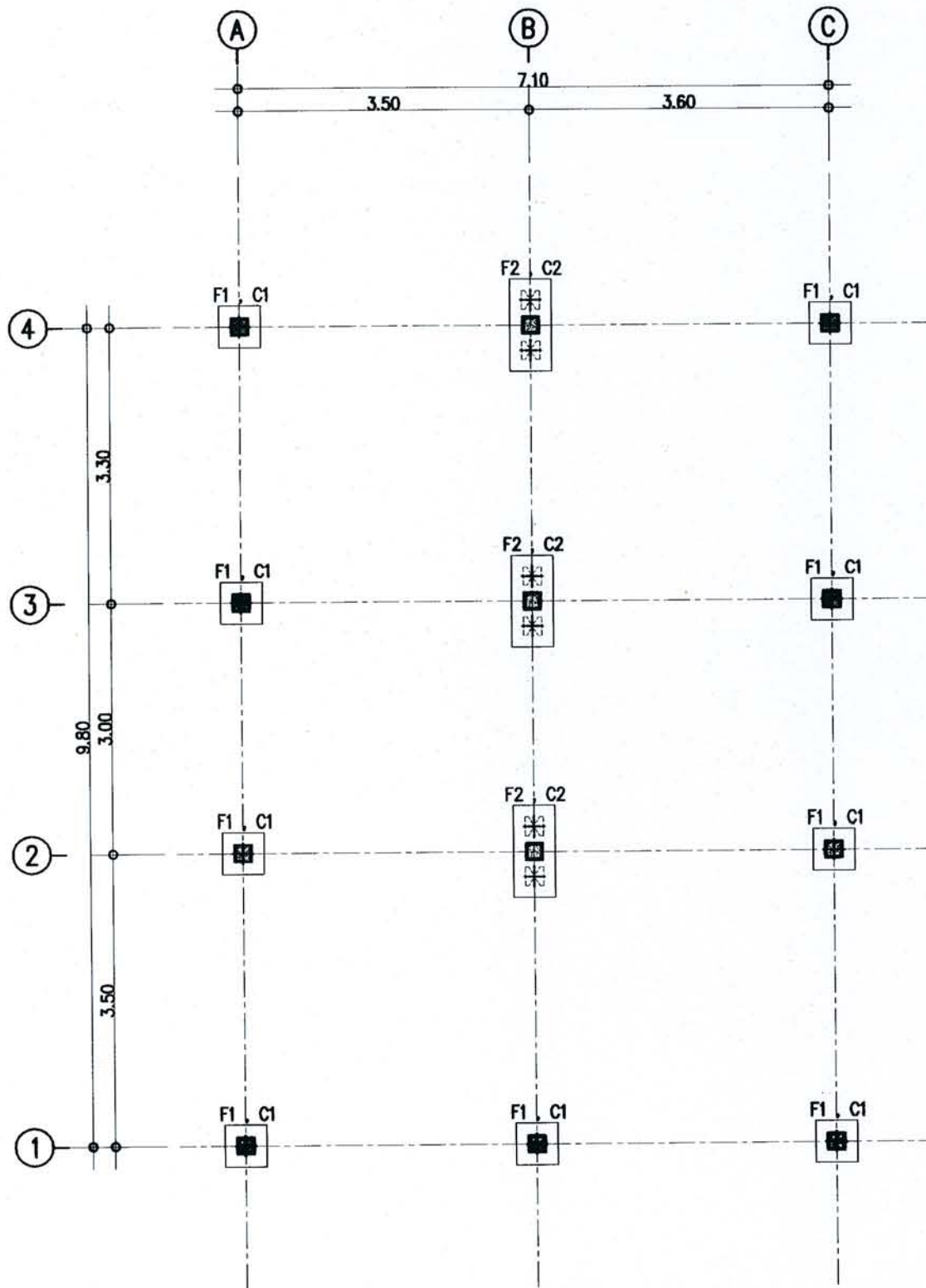
แปลนเสาเข็มและฐานราก มาตราส่วน 1 : 75
