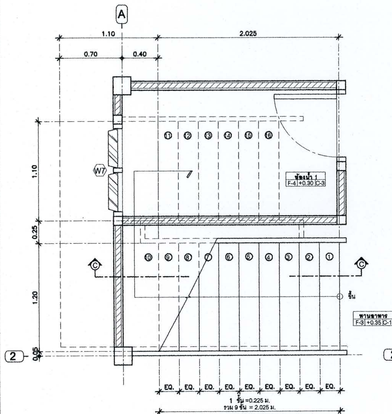
ผังบ้านได้ชั้น 1 มาตราส่วน 1:25
