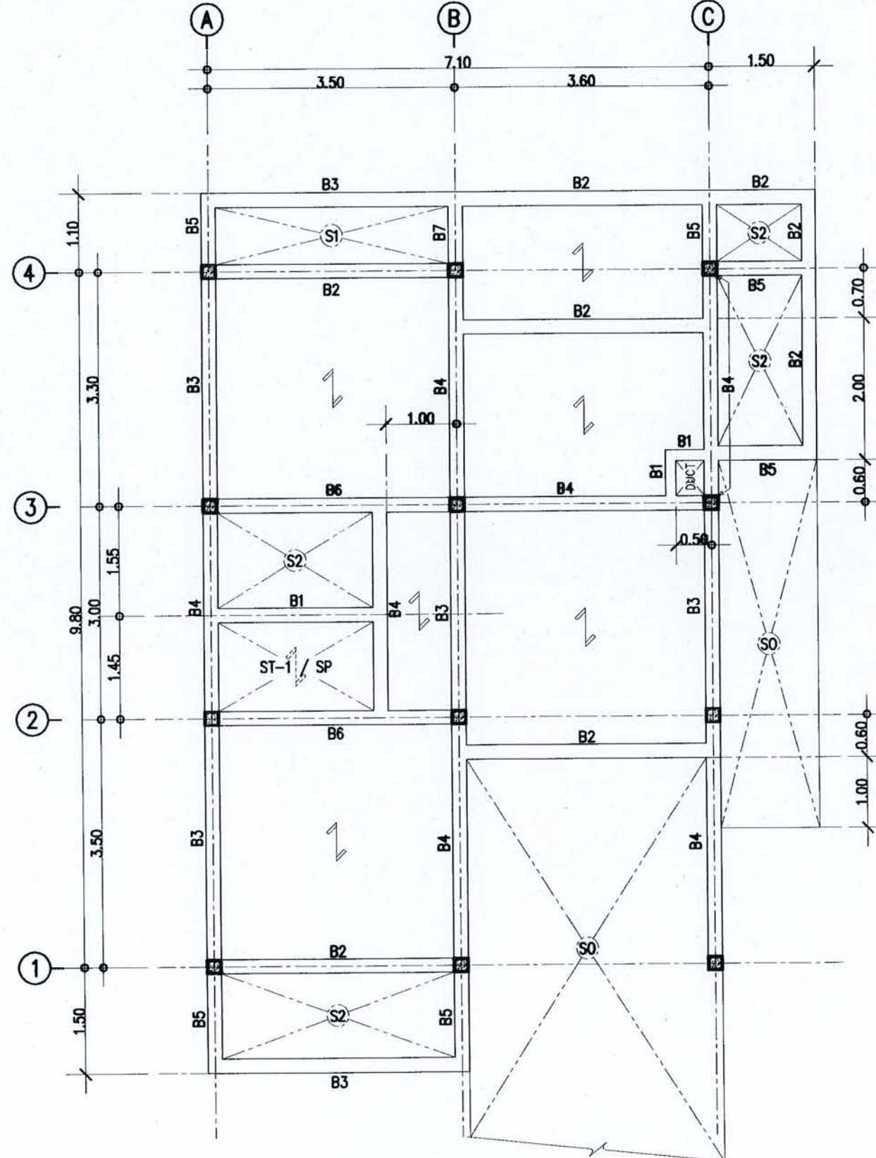
แปลนโครงสร้างชั้นล่าง มาตราส่วน 1 : 75
