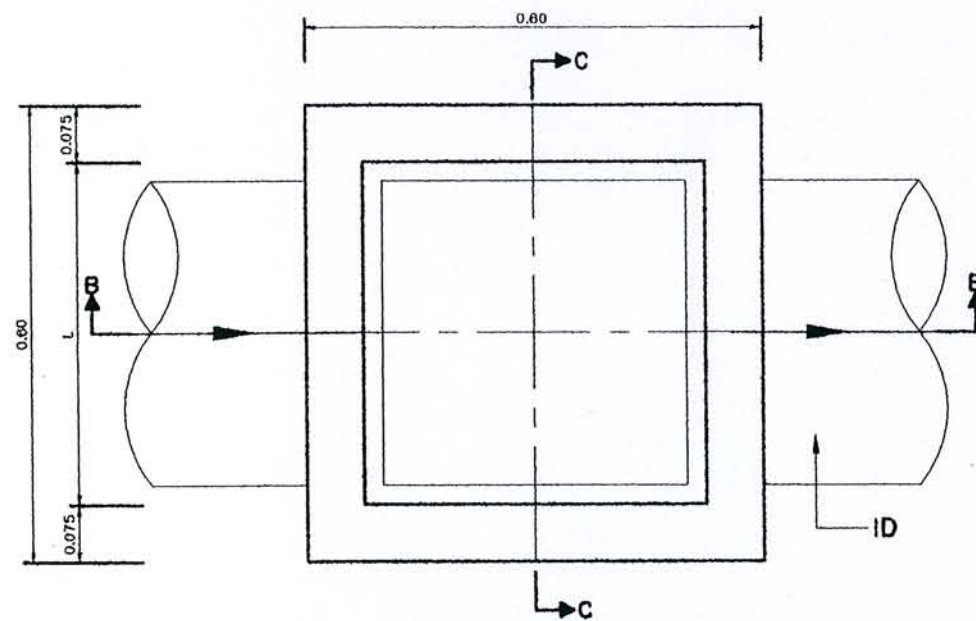
แบบขยายข้อพักสำเร็จรูปมาตรฐาน มาตราส่วน 1:10
