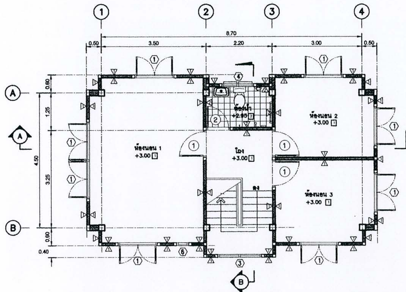
แปลนพื้นชั้นบน มาตราส่วน 1:75
