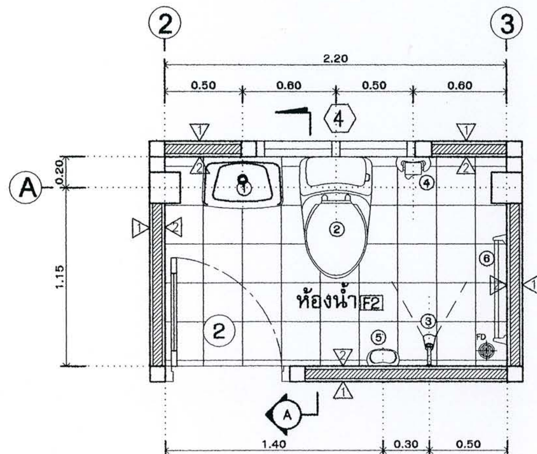
ขยายห้องน้ำ 1, 2 มาตราส่วน 1:25
