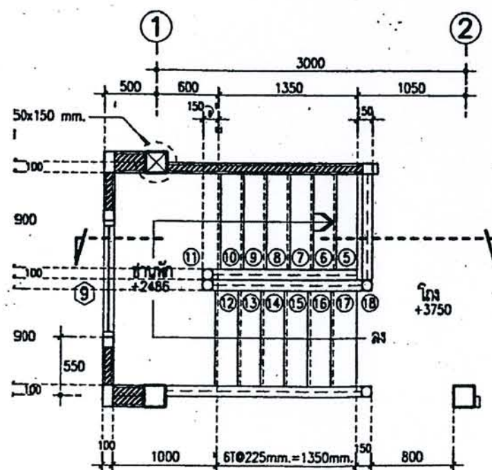
แปลนขยายบันไดชั้นบน มาตรฐาน 1:50
