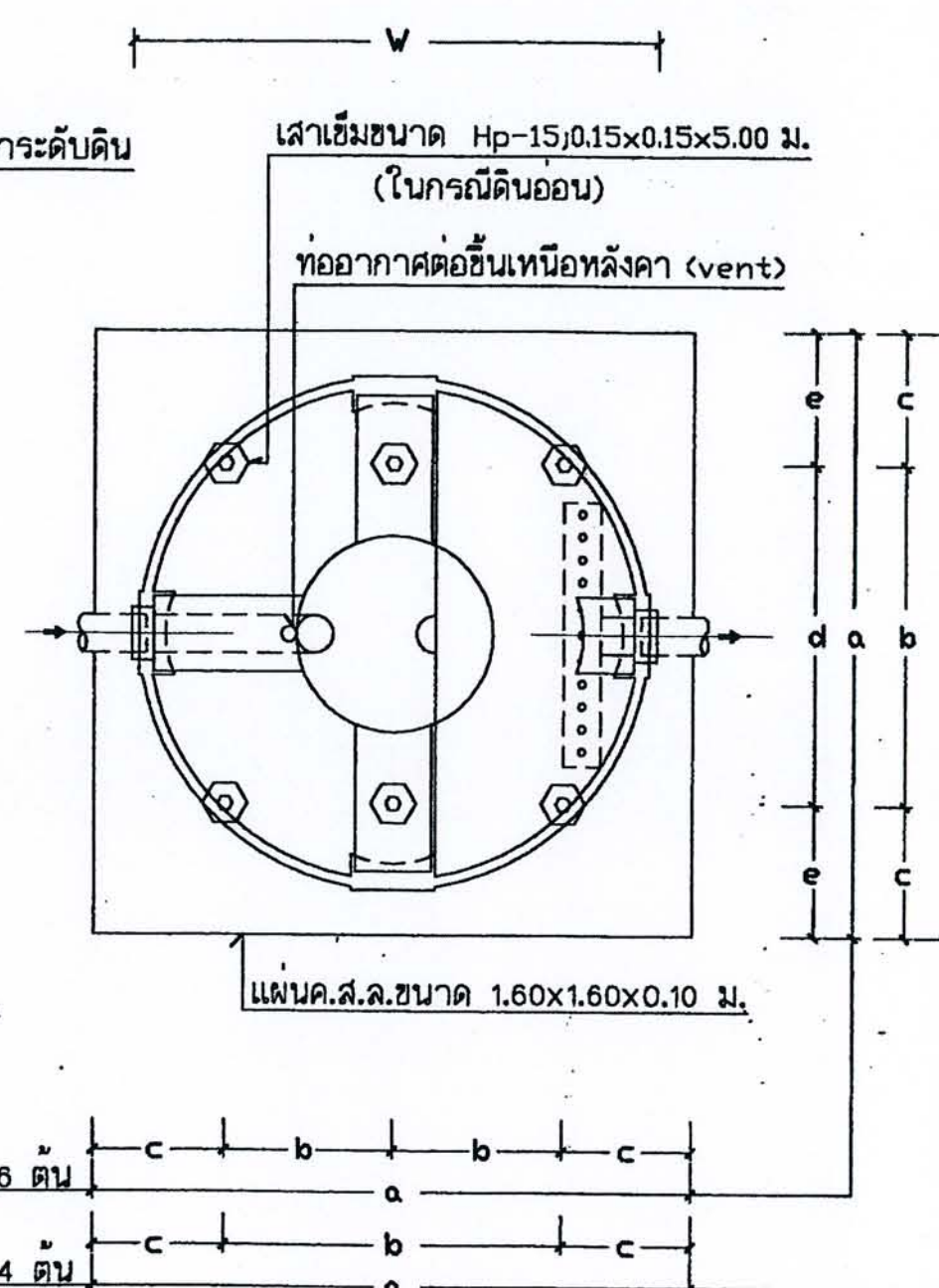
PLAN 1:20
