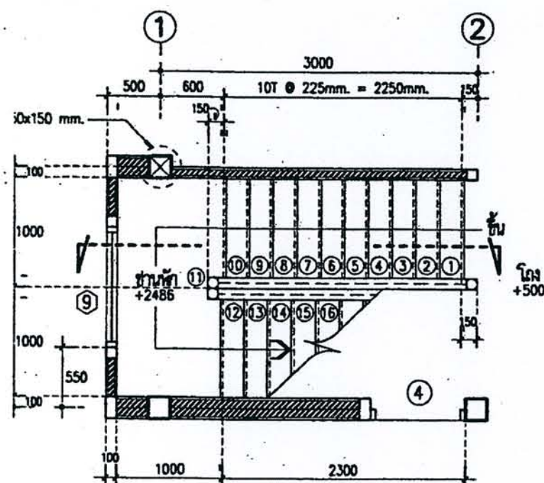
แปลนขยายบันไดชั้นล่าง มาตรฐาน 1:50
