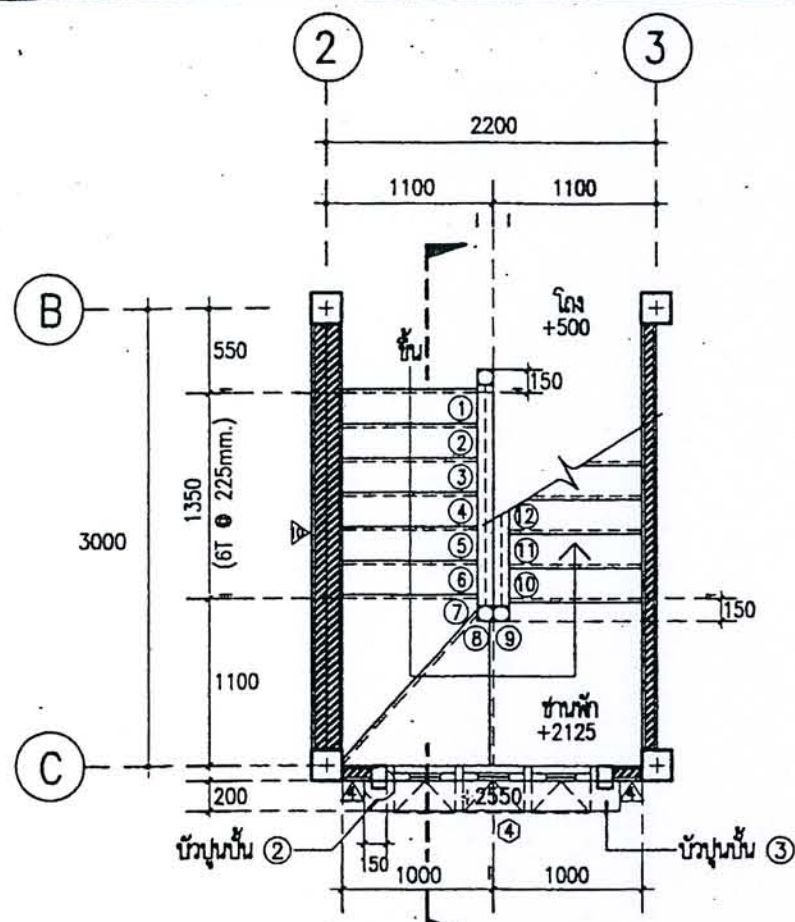
แปลนขยายบันไดชั้นล่าง
