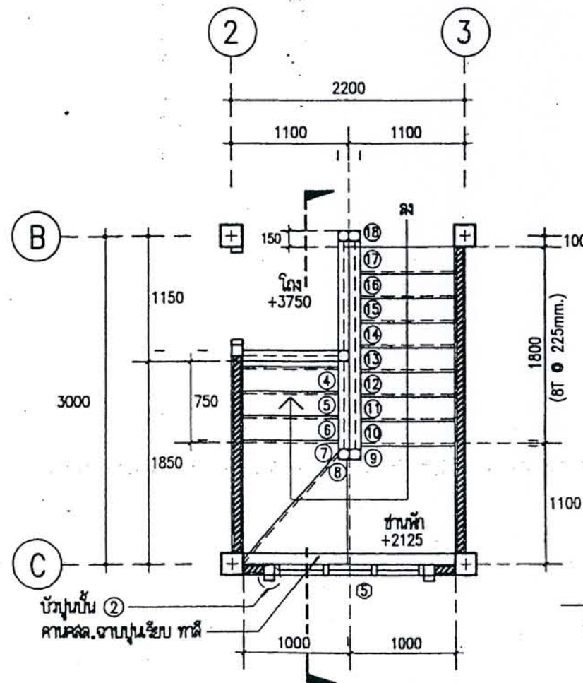
แปลนขยายบ้านได้ชั้นบน
