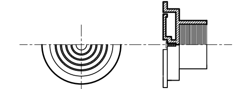
แบบขยายฝักบัวท่อระบายอากาศเหล็กหล่อชนิดออกด้านข้าง ( AVC )
