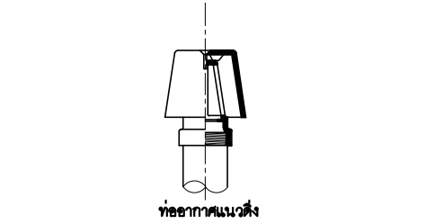
แบบขยายฝักบัวท่อระบายอากาศเหล็กหล่อ ( AVC )
