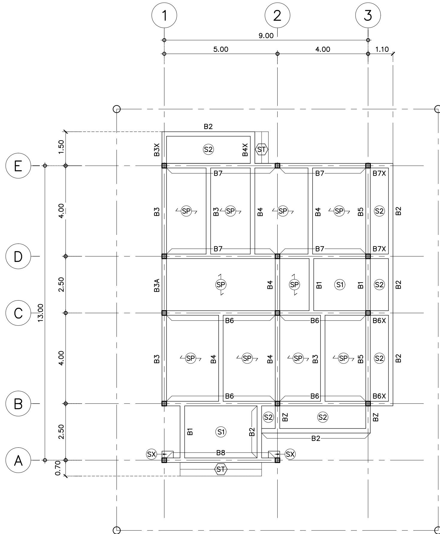
แปลนเสา คาน และพื้นชั้นล่าง มาตราส่วน 1:100
