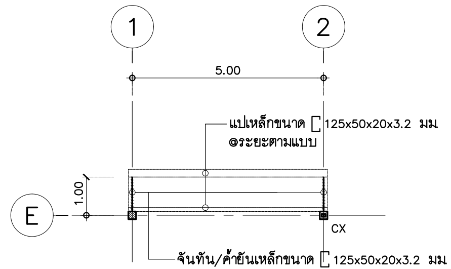
แปลนหลังคาคลุมซีกล่าง
