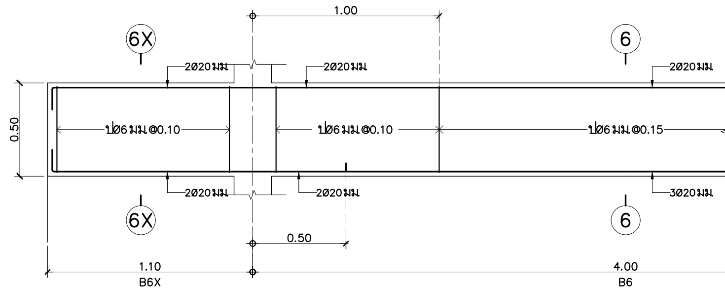
B6X, B6 มาตรฐาน 1: 20
