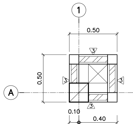
แปลนขยายฐานเสา มาตราส่วน 1 : 20
