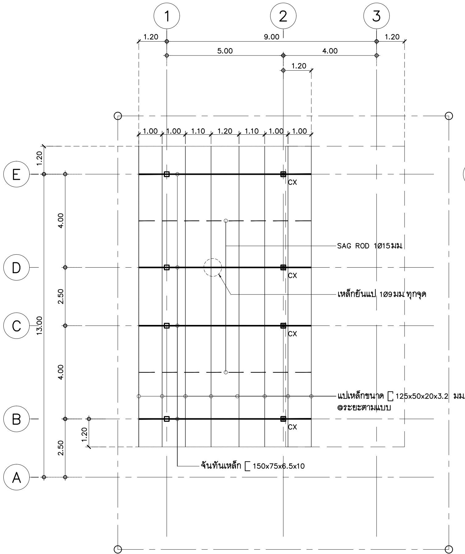
แปลนโครงหลังคาเหล็ก 2
