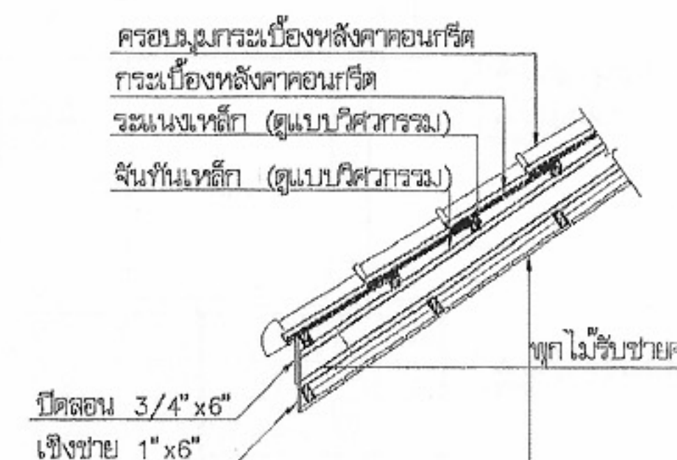
แบบขยายหลังคา 2
