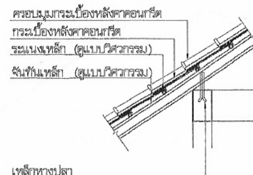
แบบขยายหลังคา 2
