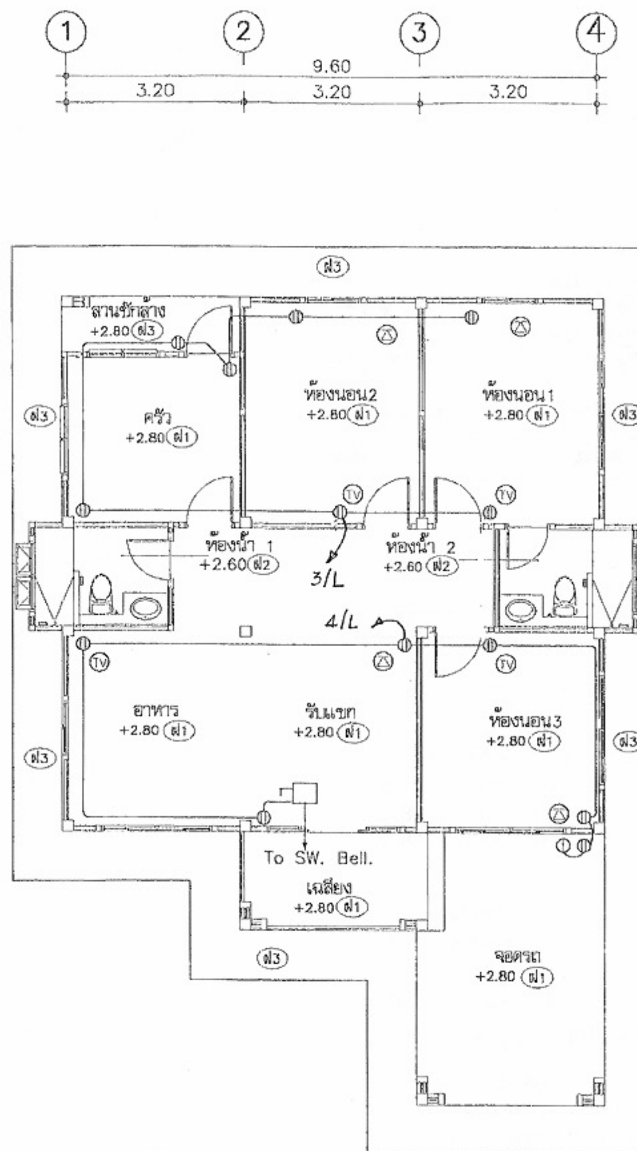
แปลนเดินรับไฟฟ้า, ไทรอคัพท์ และที่รี มาตราส่วน 1:100
