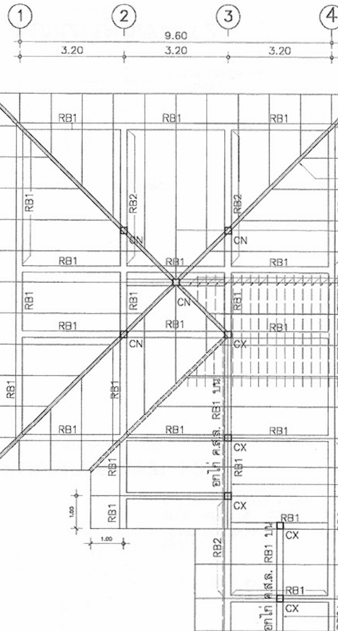
แปลนโครงหลังคา มาตราส่วน 1:100
