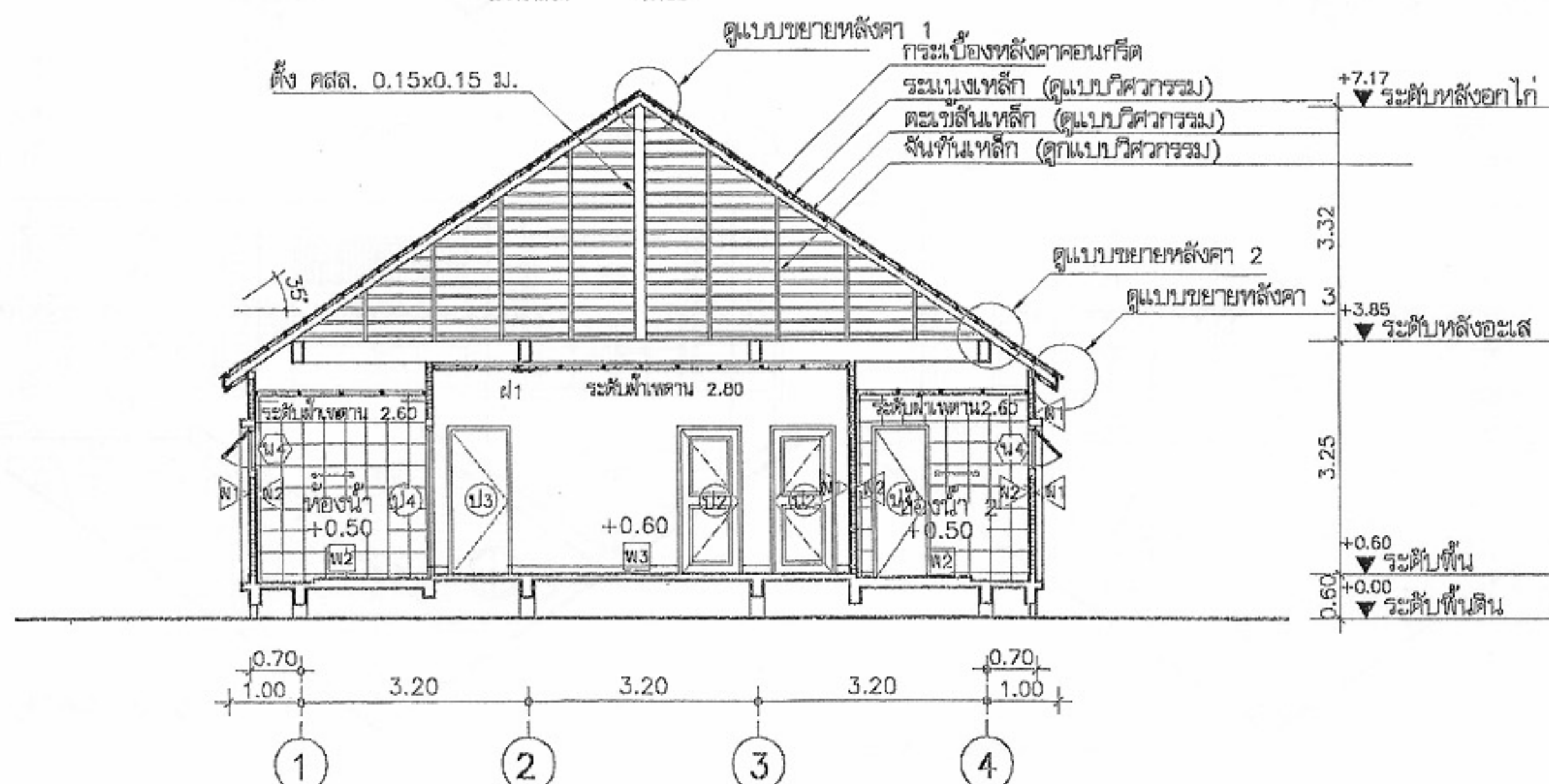
รูปที่ ๒ มาตราส่วน 1:100
