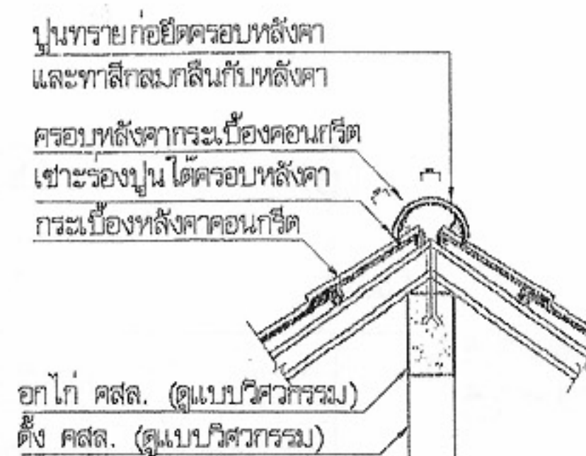
แบบขยายหลังคา 1
