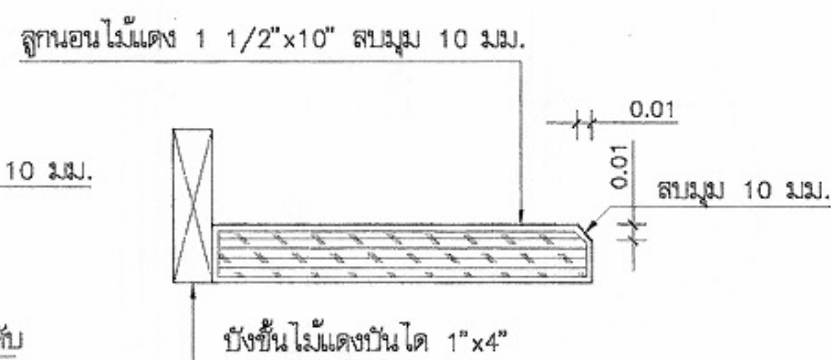
แบบขยายบันไดชั้นบน มาตราส่วน 1:25
