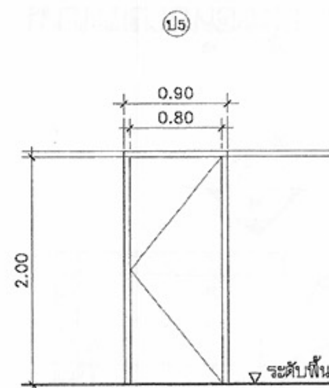
ประตูบานเปิดเดี่ยว วงกบ ไม้เต็ง ขนาด 2"x4" ไฟเบอร์สำเร็จรูป
