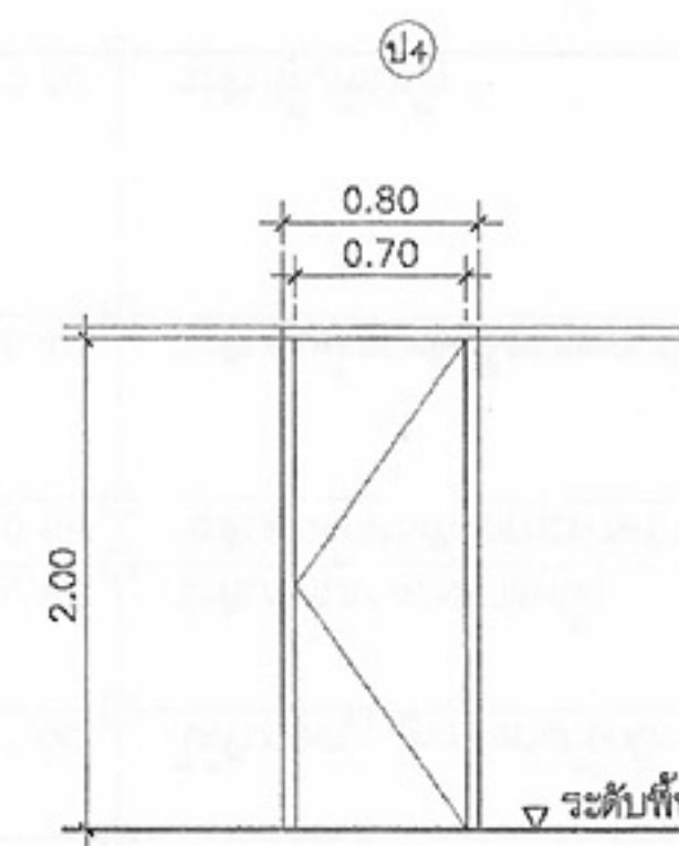
ประตูบานเปิดเดี่ยว วงกบ ไม้เต็ง ขนาด 2"x4" กรอบบาน ไม้อัดยางกันน้ำ ทาสีน้ำมัน 2 ด้าน
