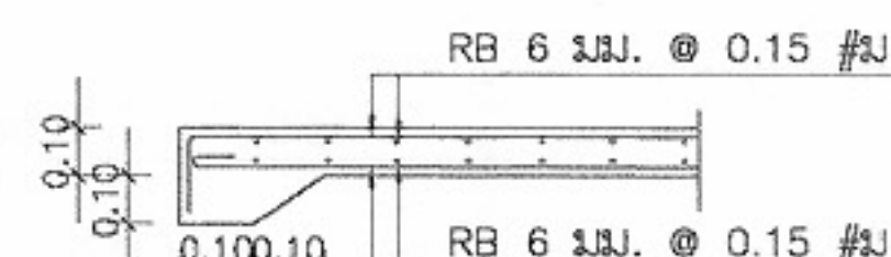
แบบขยายพื้น GS
