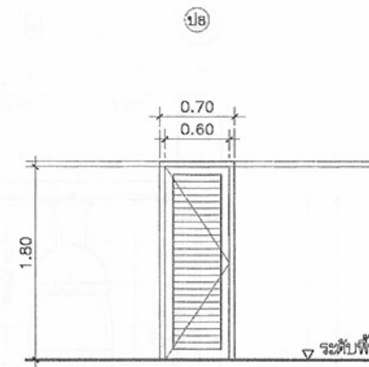
ประตูบานเกร็ด วงกบ ไม้เต็ง ขนาด 2"x4" กรอบบาน ไม้สัก 1 1/4"x4" ลูกฟัก เกร็ดไม้สัก 1 1/2"x2" ทาสีน้ำมันทั้ง 2 ด้าน
