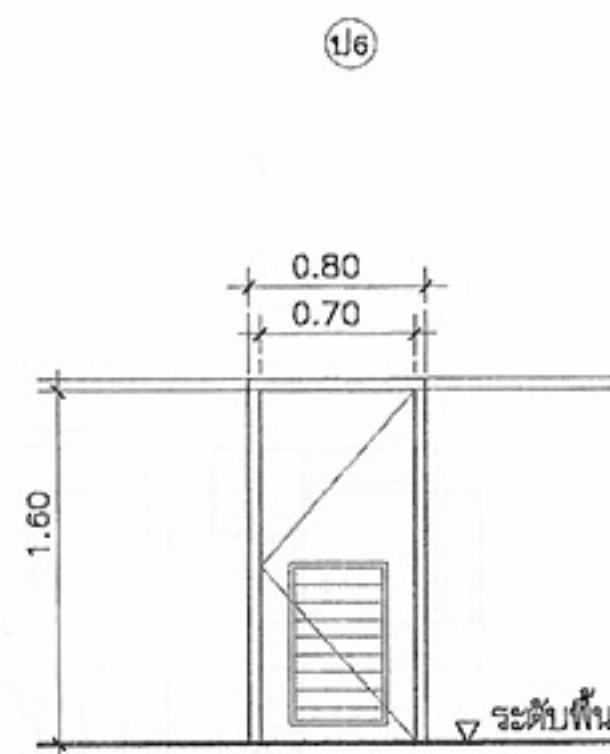
ประตูบานเปิดเดี่ยว วงกบ ไม้เต็ง ขนาด 2"x4" กรอบบาน ไม้อัดยาง ทาสีน้ำมัน 2 ด้าน
