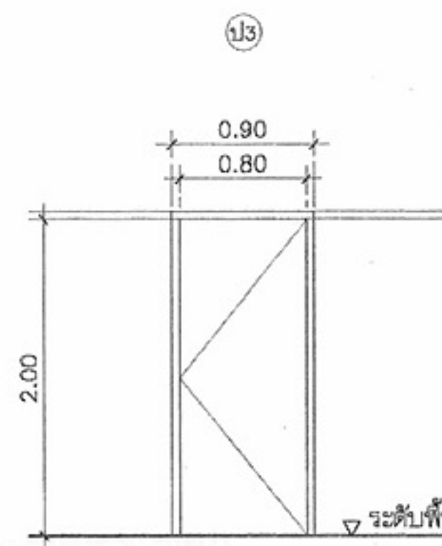
ประตูบานเปิดเดี่ยวสำเร็จรูป วงกบ ไม้เต็ง ขนาด 2"x4" กรอบบาน ไม้อัดยางกันน้ำ ทาสีน้ำมัน 2 ด้าน
