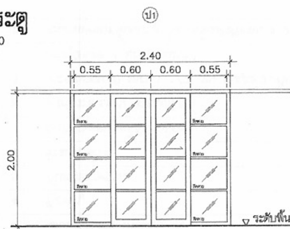
ประตูบานเปิดคู่พร้อมบานกระຈักติดตาย วงกบ อลูมิเนียม กรอบบาน อลูมิเนียม ลูกฟักกระຈักใส่หนา 5 มม.
