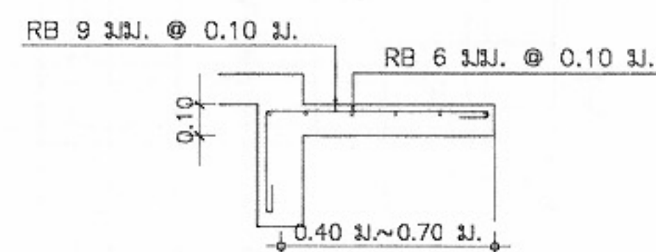
แบบขยายพื้น S3
