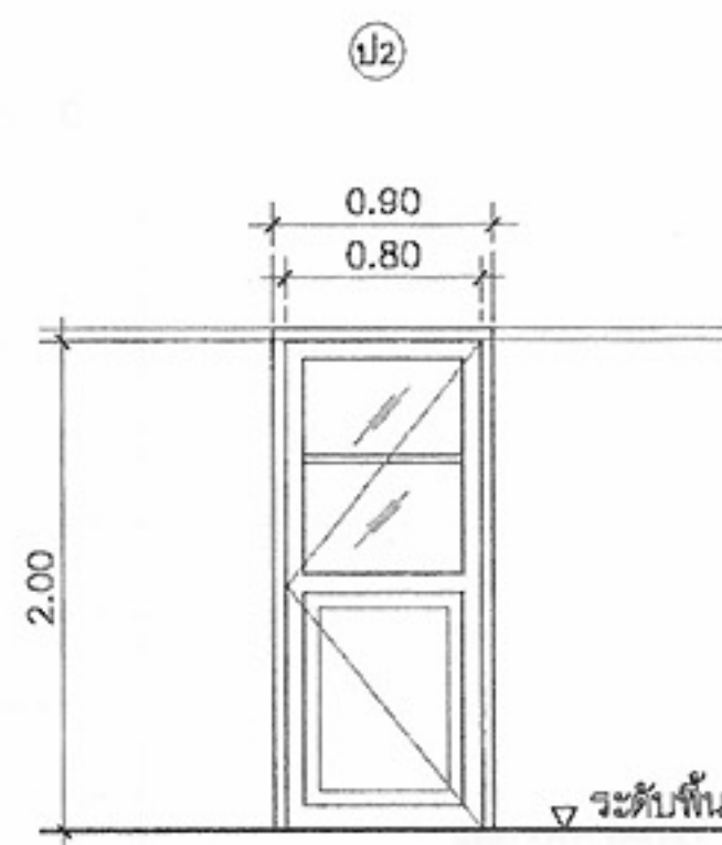
ประตูบานเปิดเดี่ยว วงกบ ไม้เต็ง ขนาด 2"x4" กรอบบาน ไม้สัก 3/4"x1 1/4" เข้าลิ้น ลูกฟักกระຈักใส่หนา 5 มม. ทาสีน้ำมัน 1 ด้าน สีล็ก 1 ด้าน
