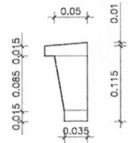
แบบขยายบัวหัวเสา มาตราส่วน 1:5
