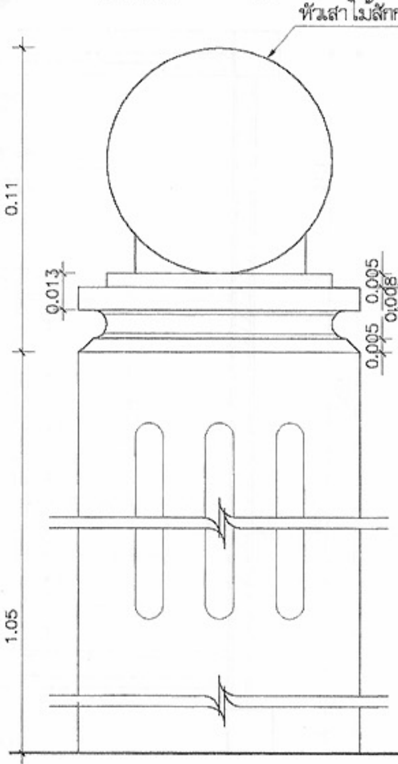
แบบขยายหัวบันได มาตราส่วน 1:2
