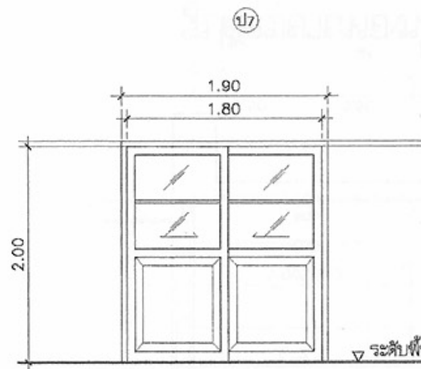
ประตูบานเลื่อน วงกบ ไม้เต็ง 2"x4" กรอบบาน ไม้สัก 1 1/2"x4" ลูกฟัก กระຈักใส่หนา 6 มม., ไม้สักเข้าลิ้น ทาสีน้ำมันทั้ง 2 ด้าน
