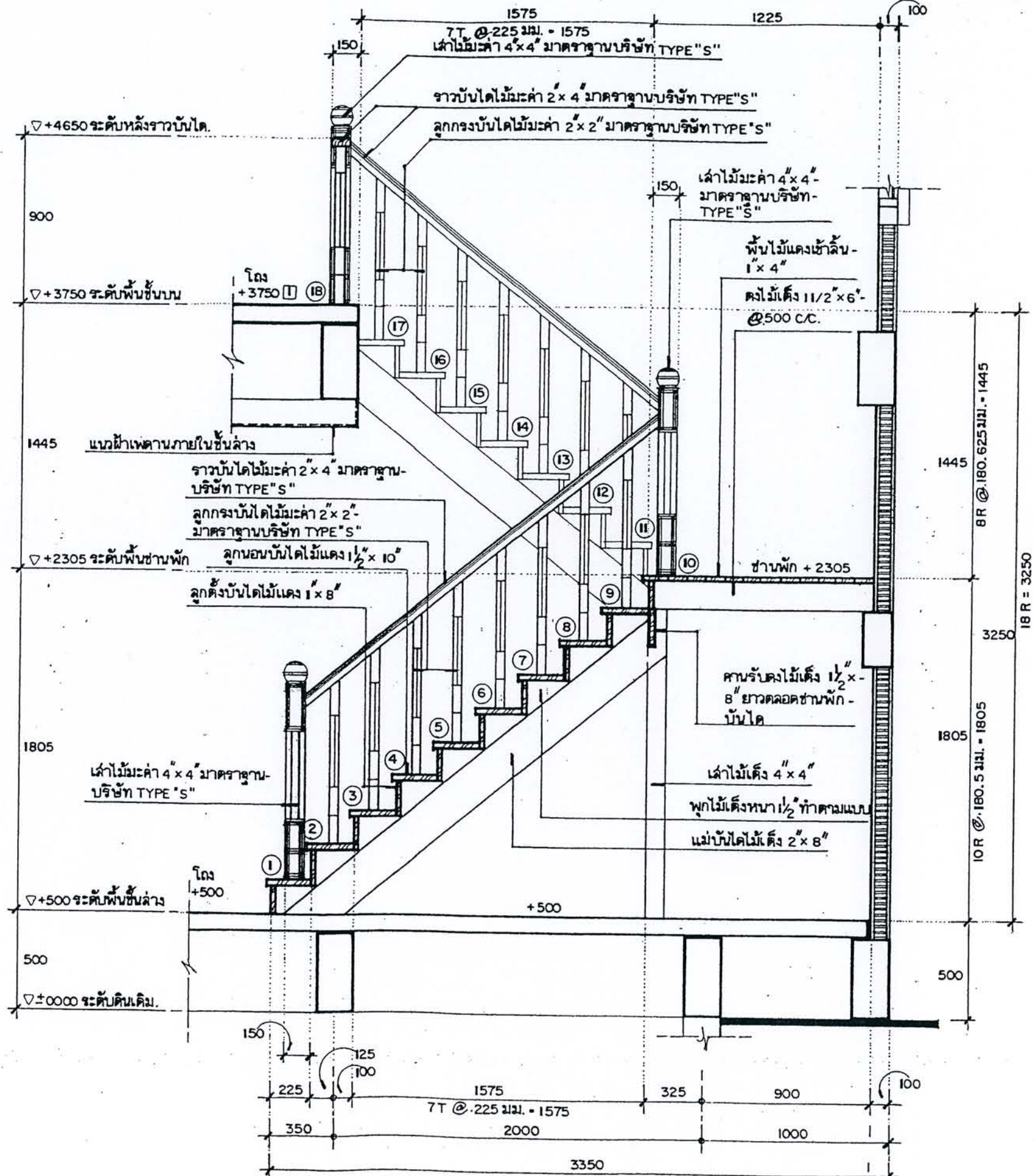
รูปตัดขยายบันได
