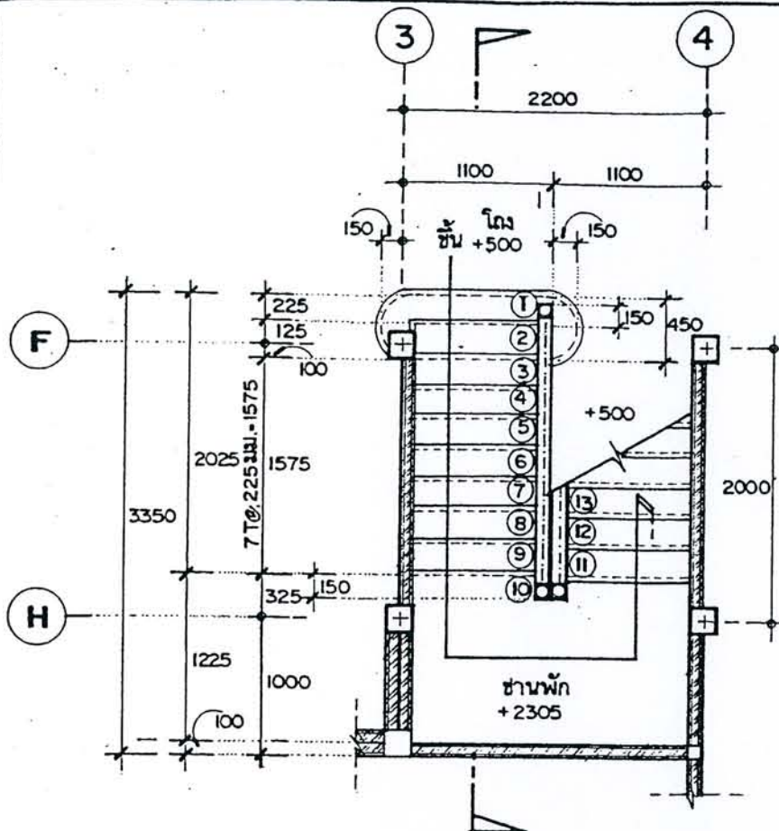
แปลนขยายบันไดชั้นล่าง
