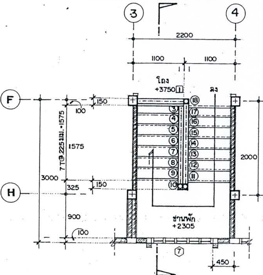
แปลนขยายบันไดชั้นบน
