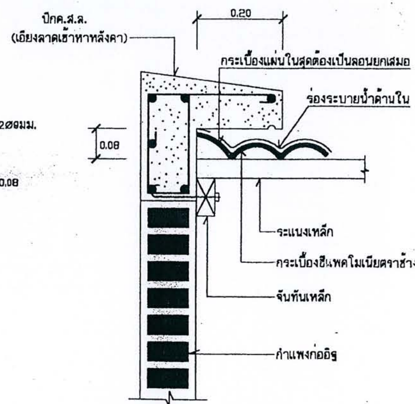
การทำปีกค.ส.ล.ชนผนัง 1:10
