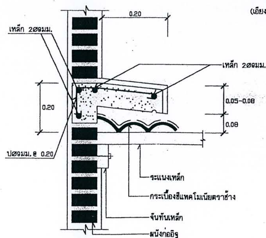
การทำปีกค.ส.ล.ชนผนัง 1:10
