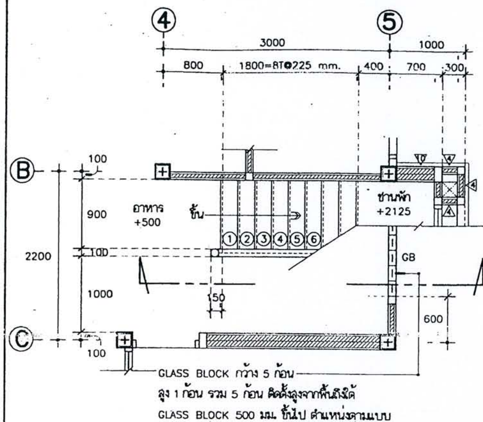
แปลนขยายบ้านได้ชั้นล่าง
