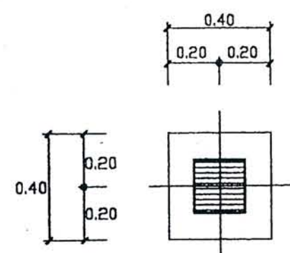
PLAN F1A
