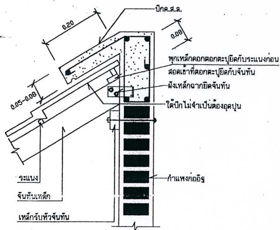
การทำปีกค.ส.ล.ชนผนัง 1:10
