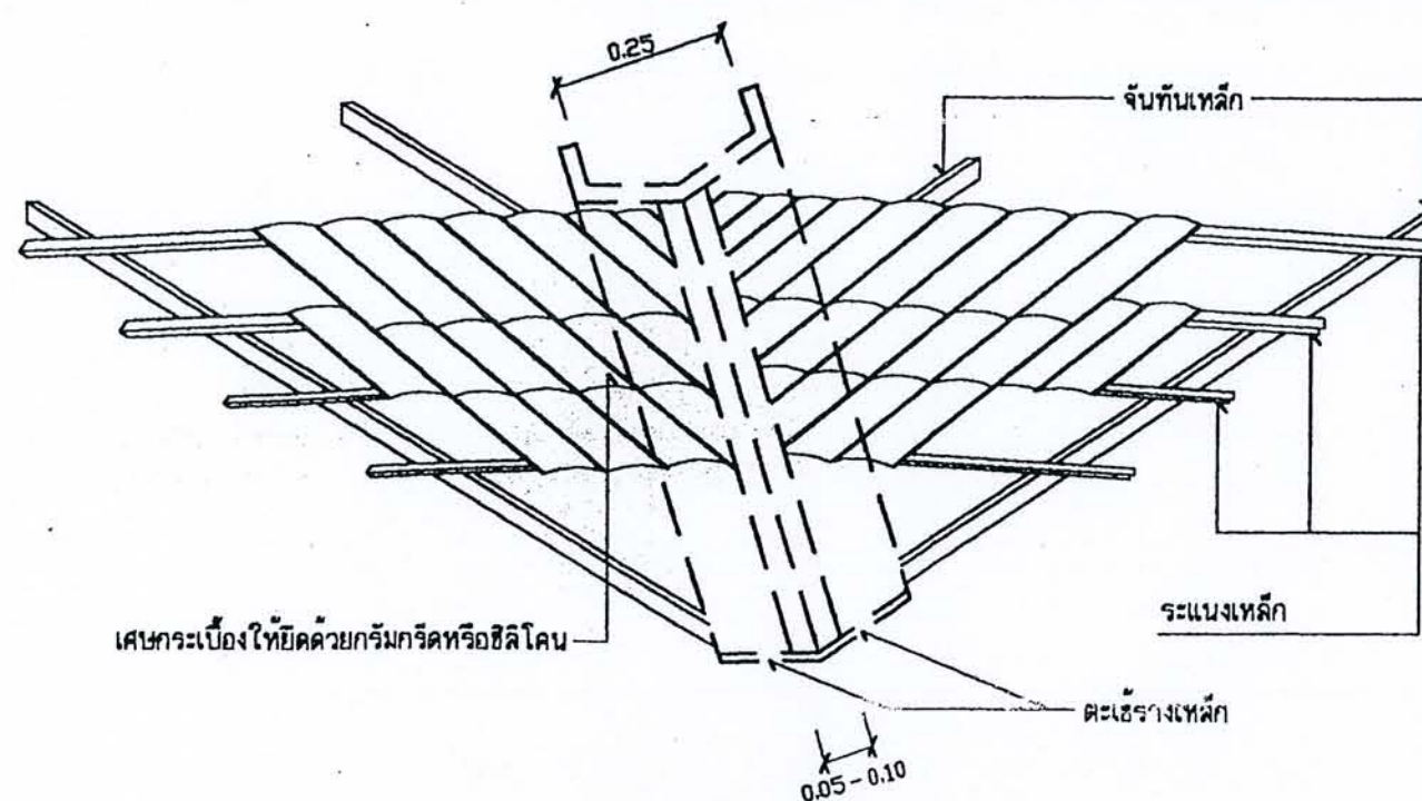
แบบขยายการทำตะเข็บราง 1:10
