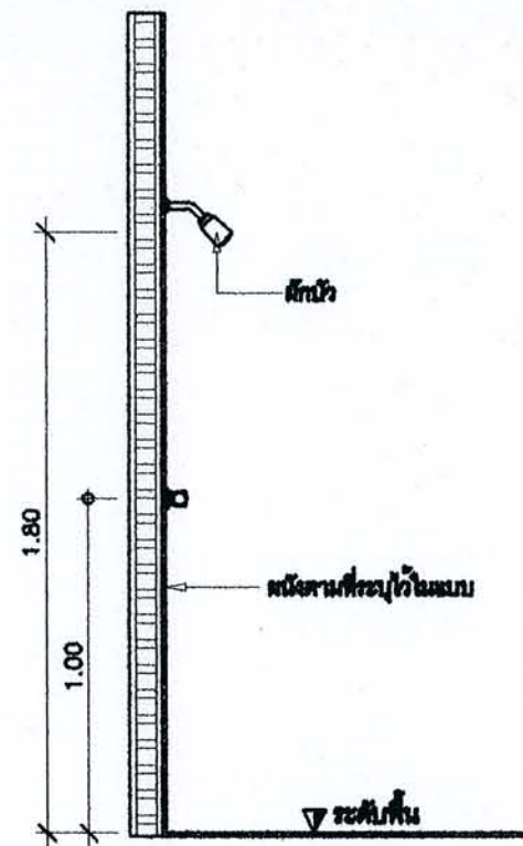
ฝักบัวอาบน้ำก้านแข็ง
