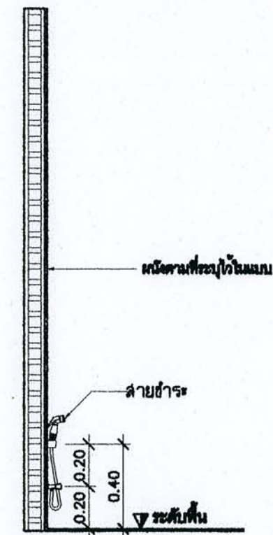
สายชำระ
