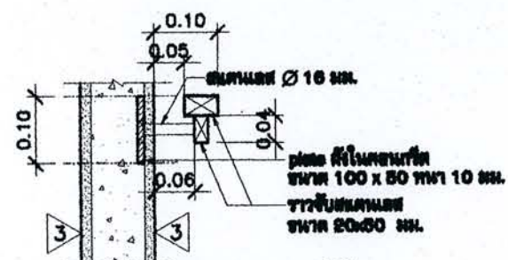
แบบขยาย 1
