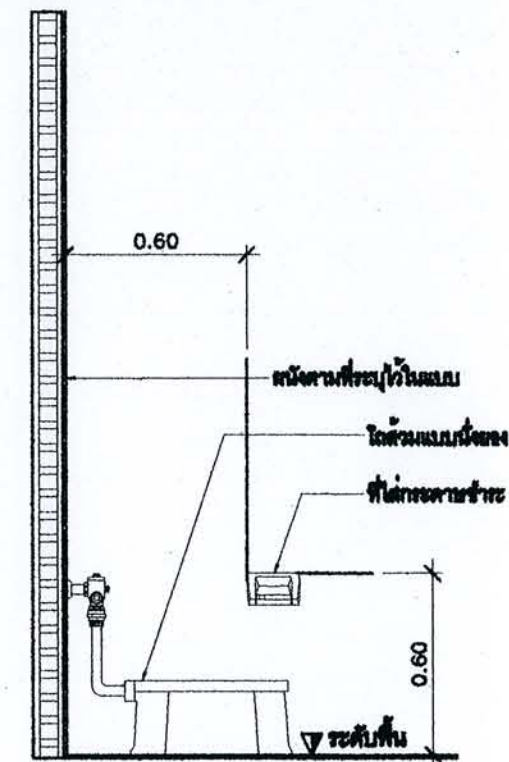
โถ้วมแบบนั่งยอง
