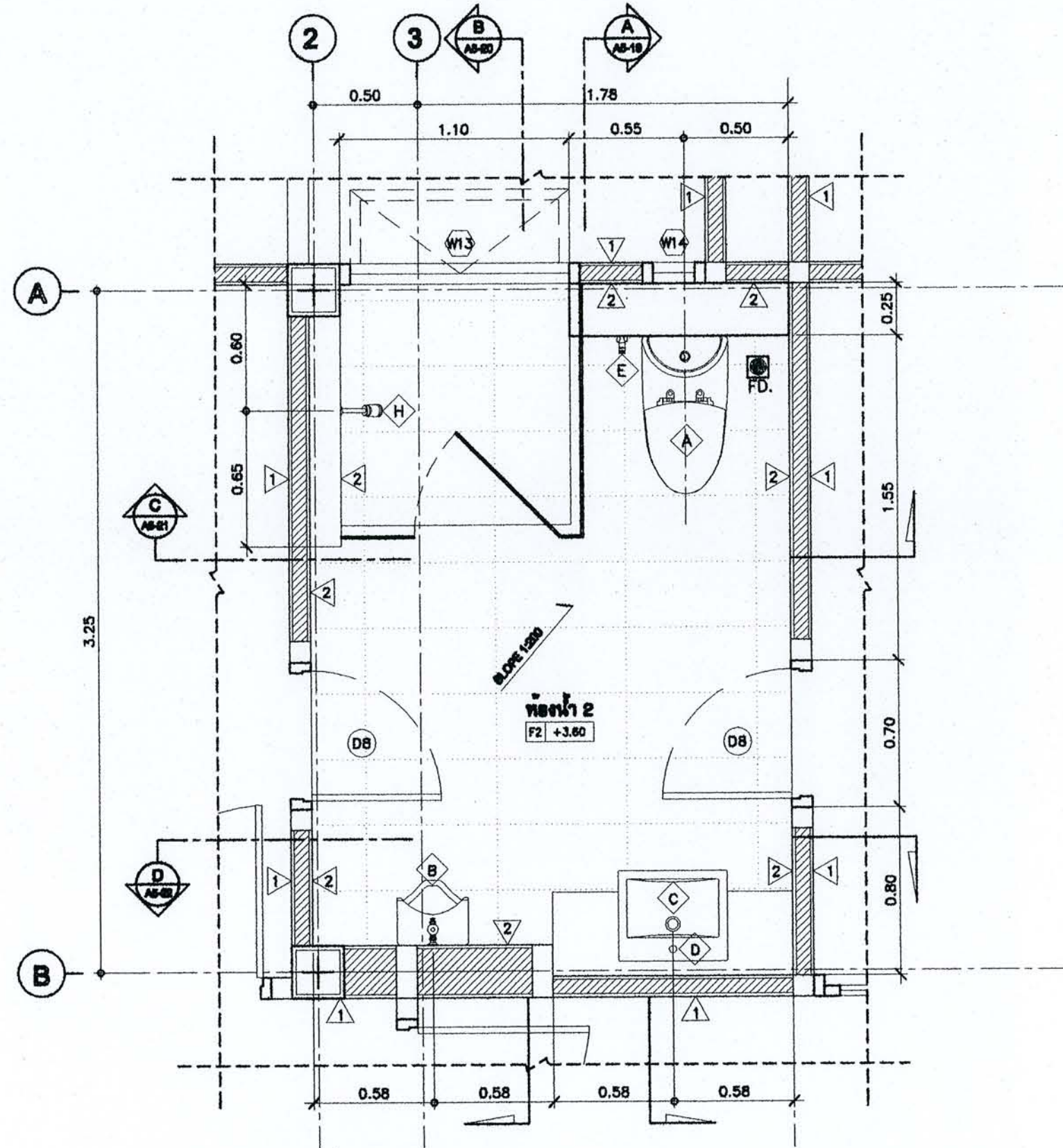
แบบขยายห้องน้ำ 2,3 มาตราส่วน 1:25
