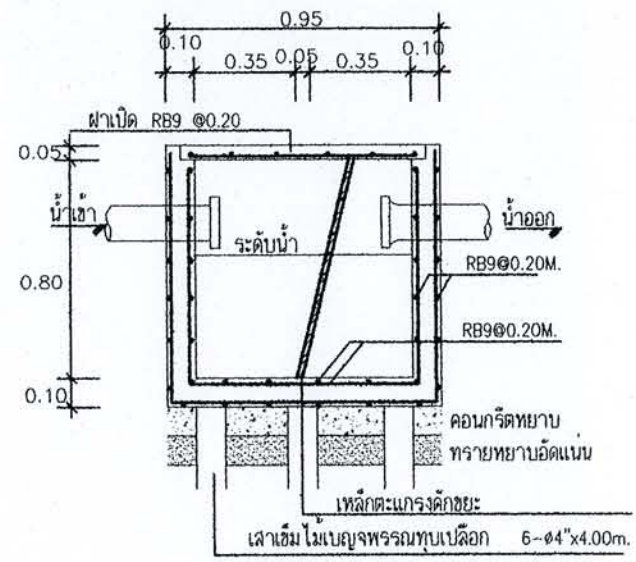
รูปตัดขยายบ่อพัก
