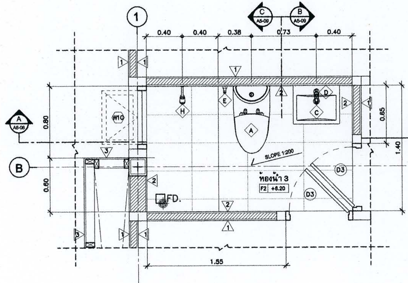
แบบขยายห้องน้ำ 3 มาตราส่วน 1:25
