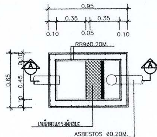
แปลนขยายบ่อพัก
