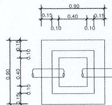
แปลนขยายบ่อพัก
