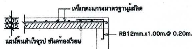
PS ช่วงริม
