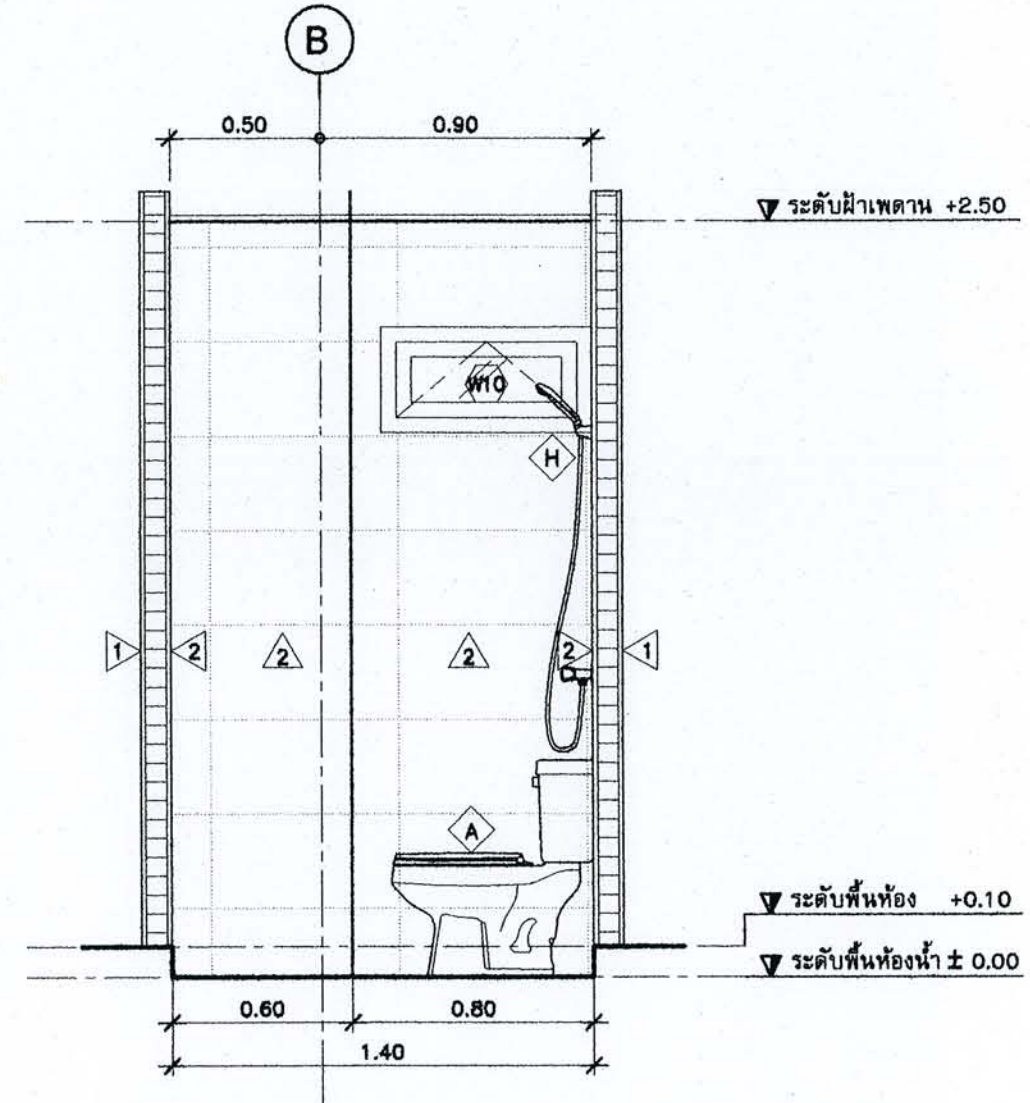
รูปตัด มาตราส่วน 1:25
