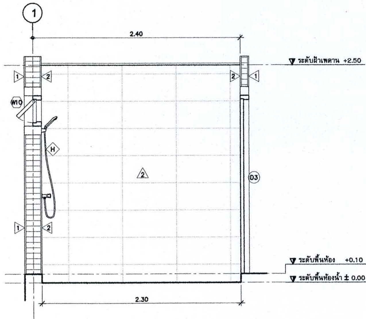
รูปตัด มาตราส่วน 1:25
