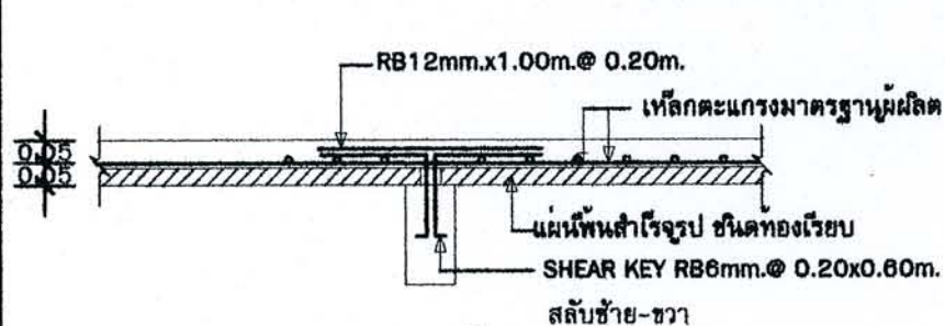
PS ช่วงต่อเนื่อง
