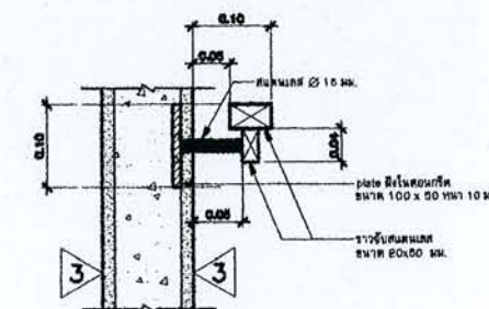
แบบขยาย ① มาตราส่วน 1:10
