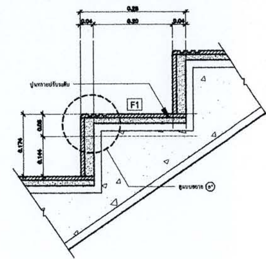
แบบขยาย ② มาตราส่วน 1:10
