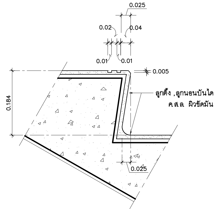
แบบขยายจุกบันได
