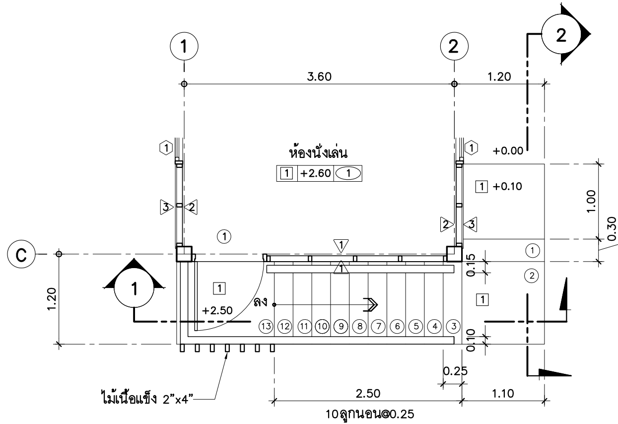
แบบขยายบันได ST.1
