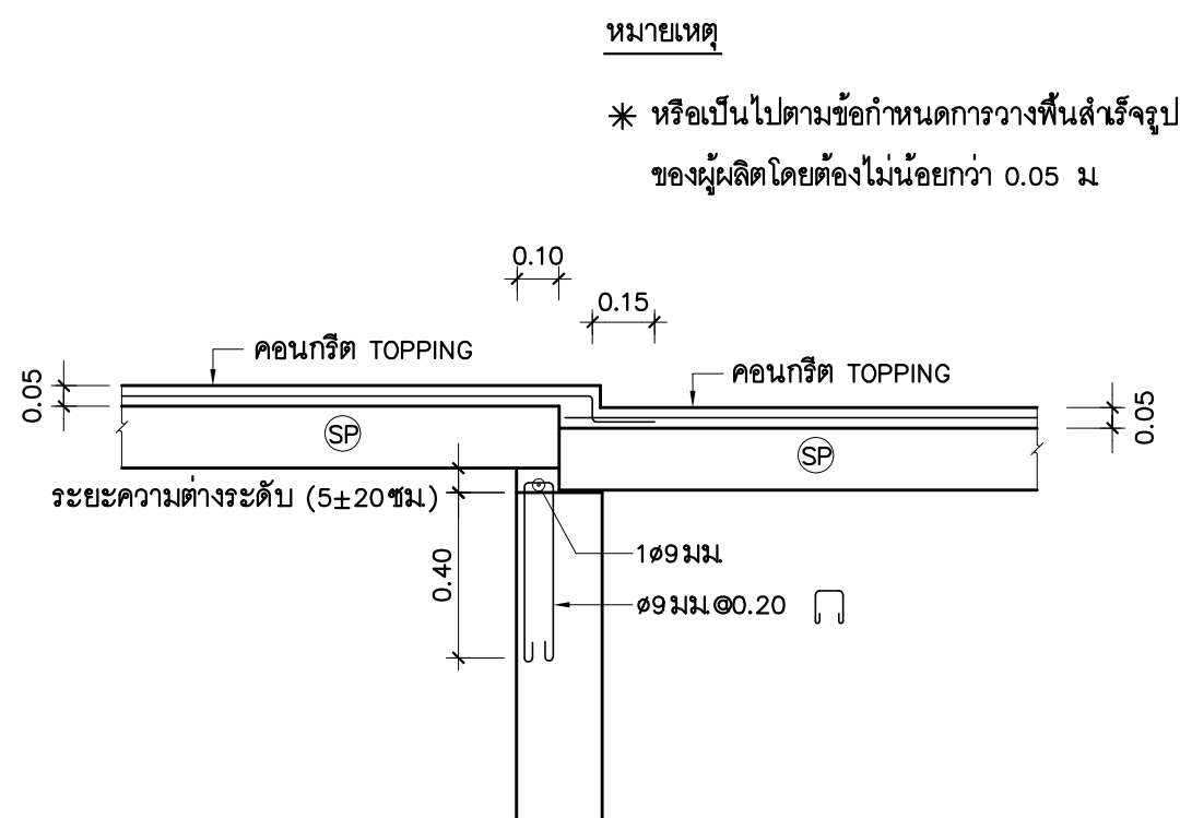
ลักษณะการหล่อพื้นเสริมกรณีเศษช่องว่างที่คานริม มาตราส่วน 1: 20
