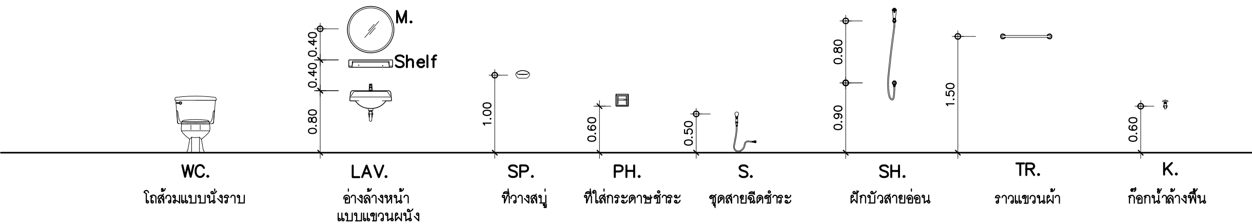
มาตรฐานการติดตั้งสุขภัณฑ์ มาตราส่วน 1 : 50
