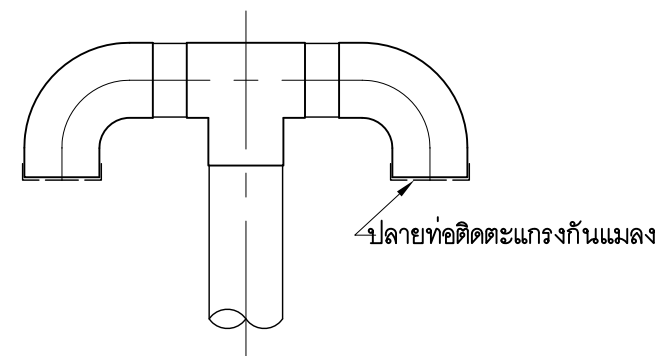
แบบขยายฝาปิดท่อระบายอากาศ ชนิดใช้ท่อและข้อต่อประกอบ ( VTR )
