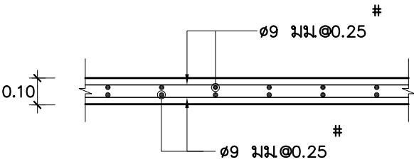
S2(ด้านสั้น)
