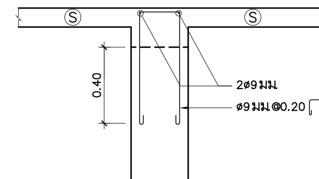
ลักษณะพื้น (S) ระดับสูงกว่าหลังคาน มาตราส่วน 1: 20
