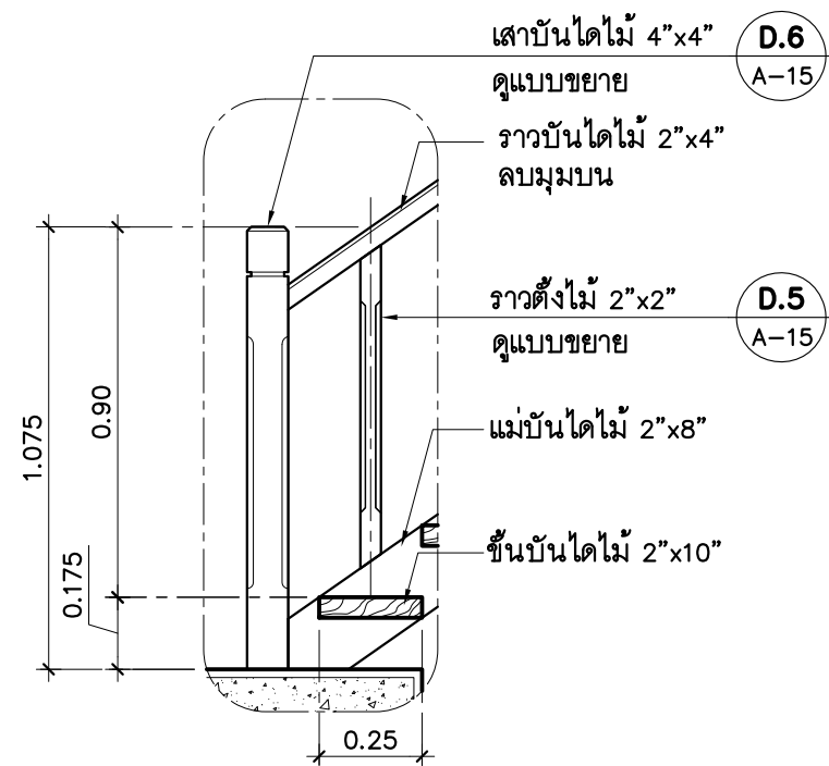
แบบขยาย D.3 มาตราส่วน 1 : 20
