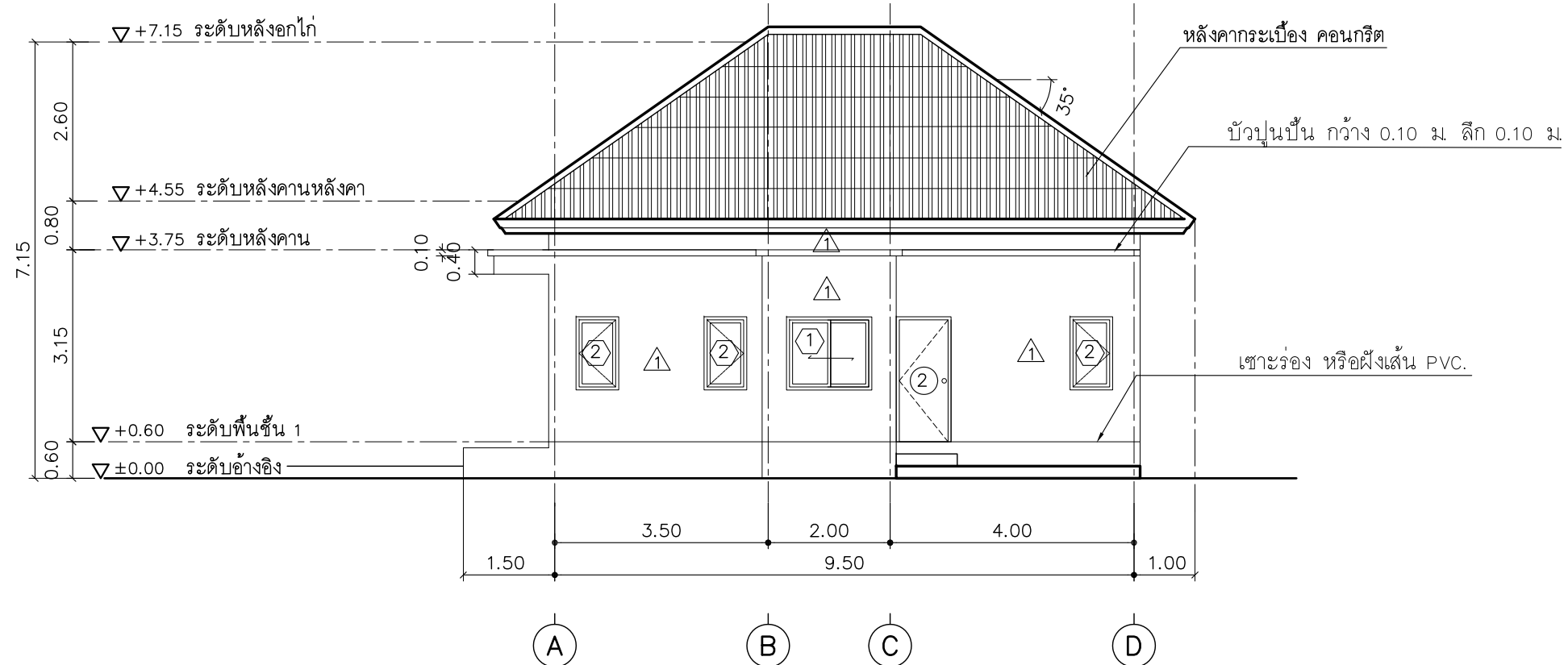
รูปด้าน 4
