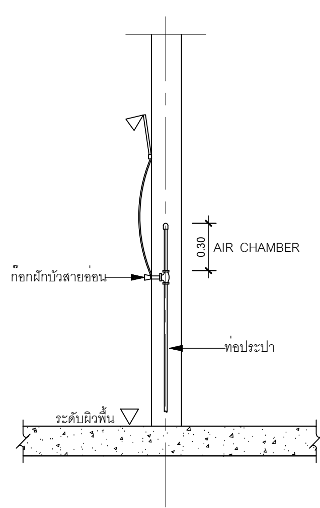
ฝักบัวอาบน้ำ ( SH )
