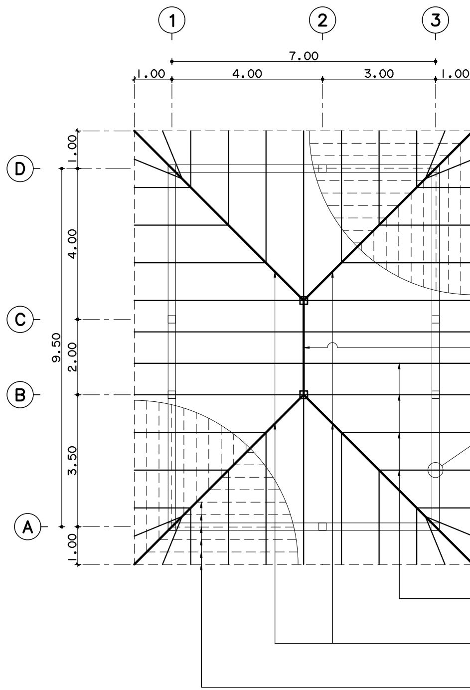
แปลนโครงหลังคา มาตราส่วน 1:100
