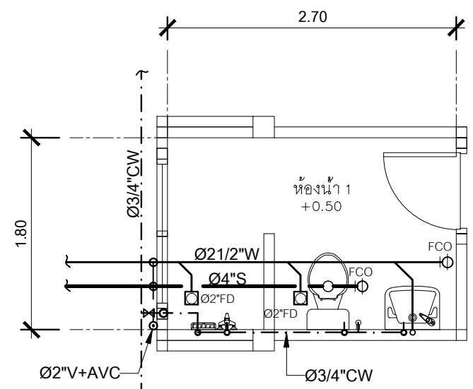
แปลนระบบสุขาภิบาลห้องน้ำ มาตรฐาน 1 : 50 ( ท่อประปาเดินใต้พื้น )
