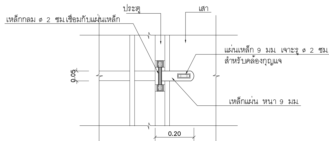
แบบขยายกลอนประตู
