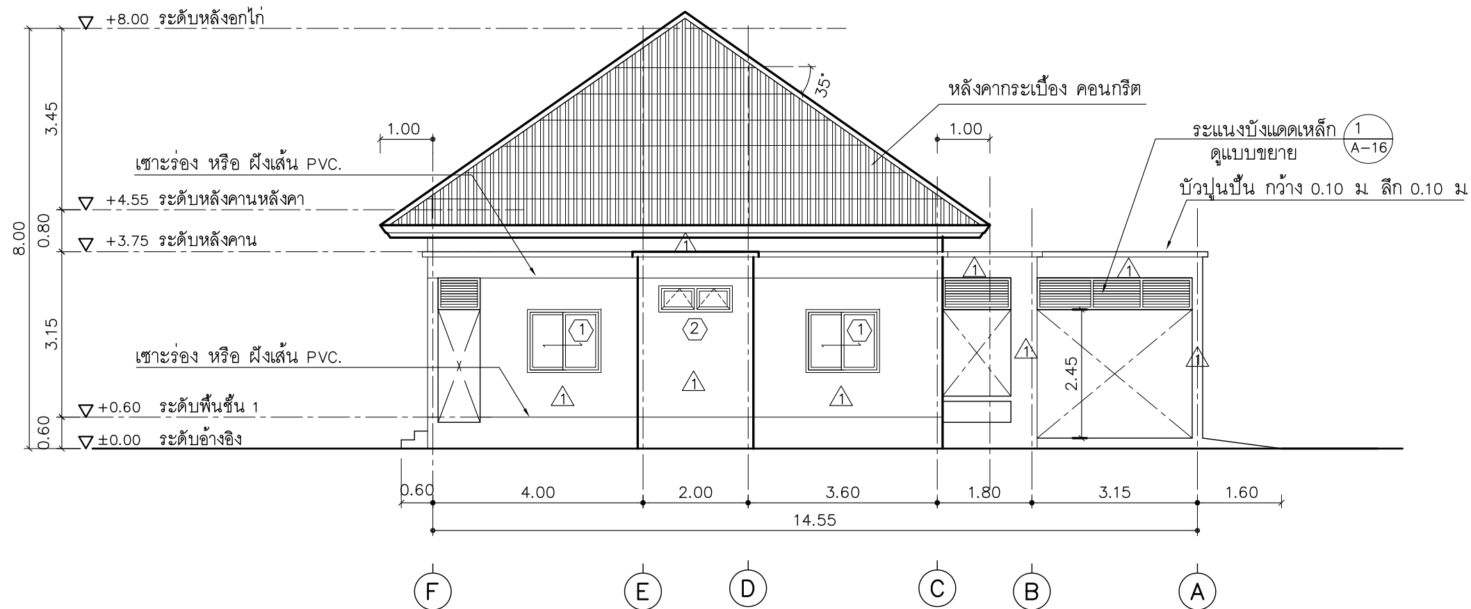
รูปด้าน 2
