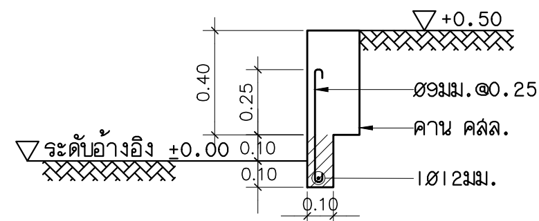
แบบขยายครีป ค.ล.ล. รอบอาคาร 1:20
