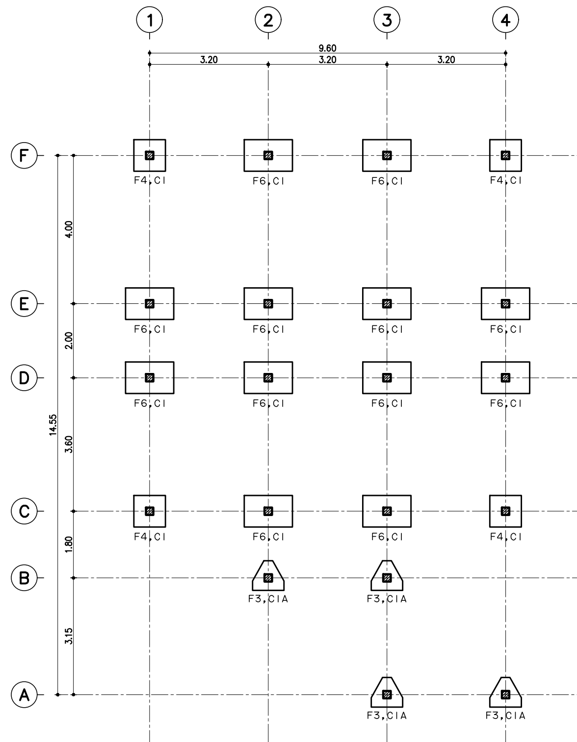
แปลนฐานรากแบบตอกเข็ม มาตรฐาน 1 : 100
