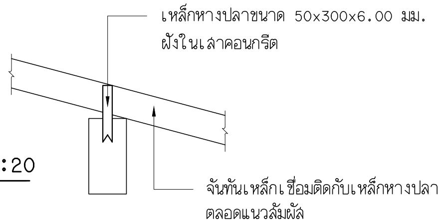
แบบขยายครีป ค.ล.ล. รอบอาคาร 1:20
