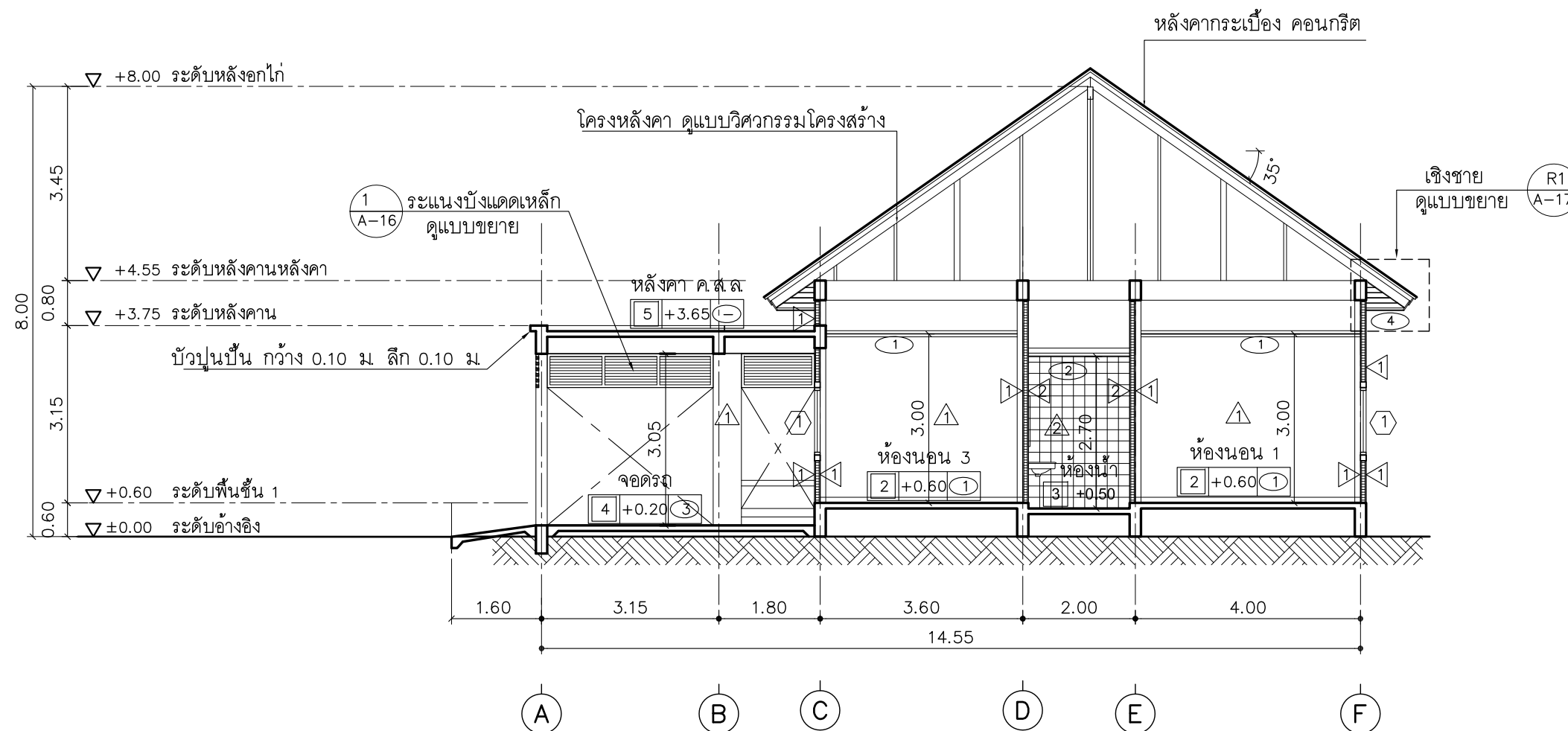
รูปตัด 2 มาตราส่วน
