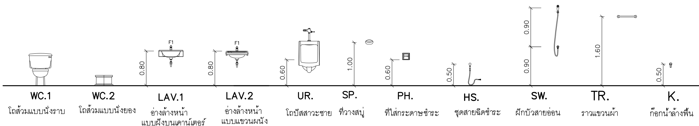
มาตรฐานระดับการติดตั้งสัญลักษณ์
