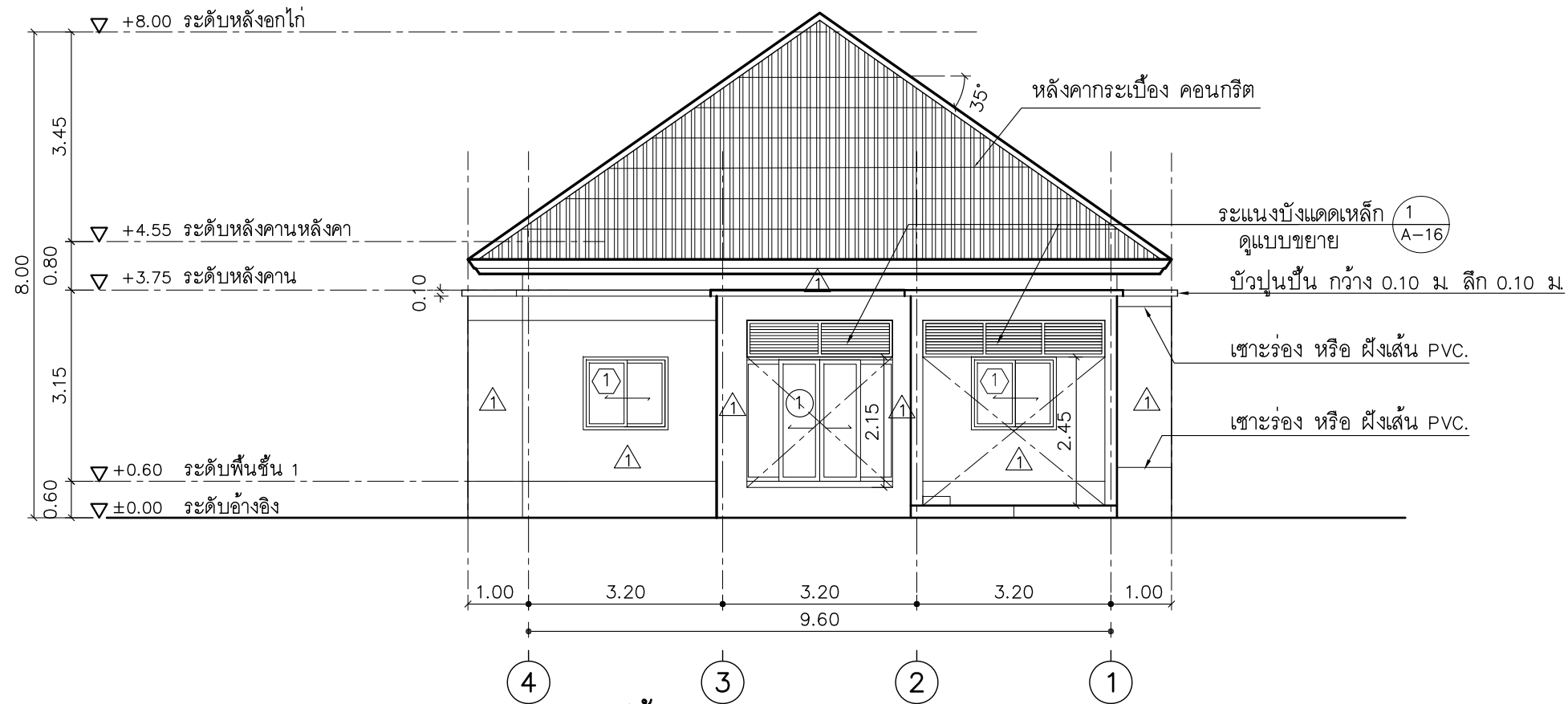
รูปด้าน 1
