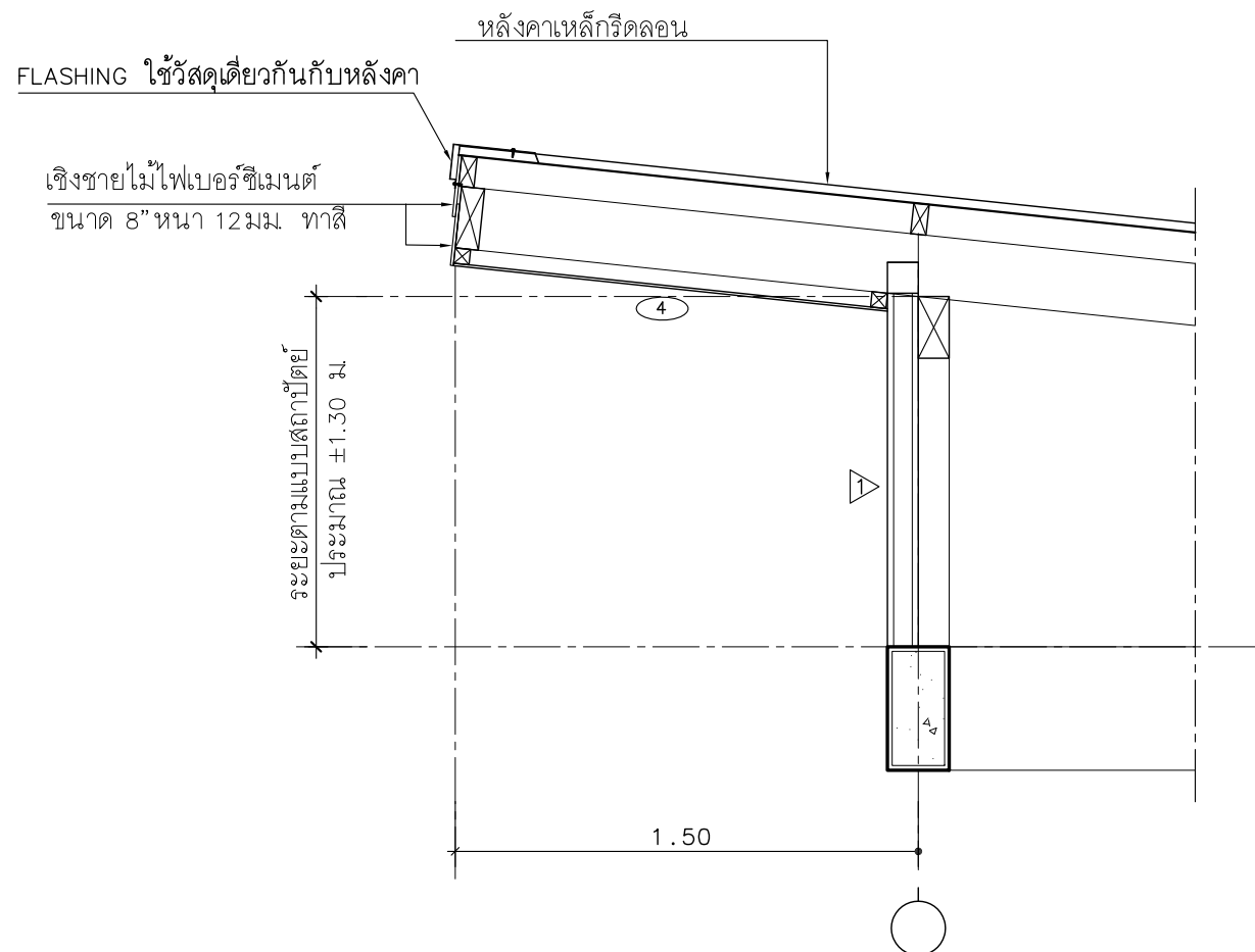
แบบขยาย เชิงชาย 1 มาตราส่วน 1: 25 (R1)
