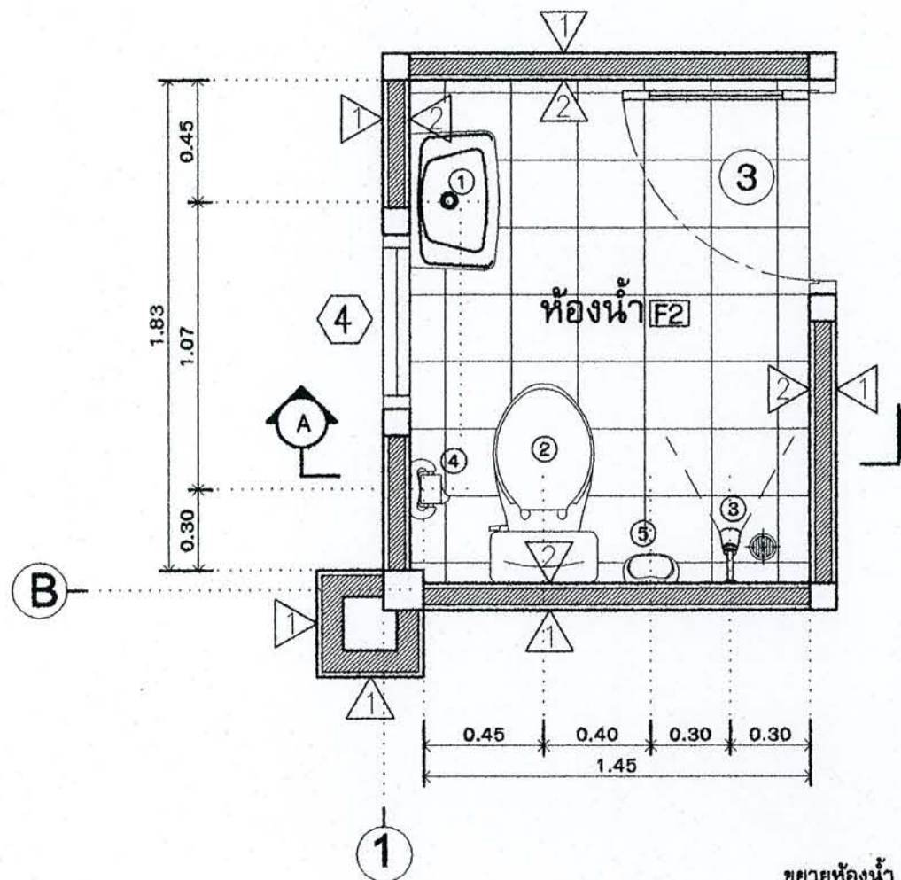
ขยายห้องน้ำ 1, 2 มาตราส่วน 1 : 25
