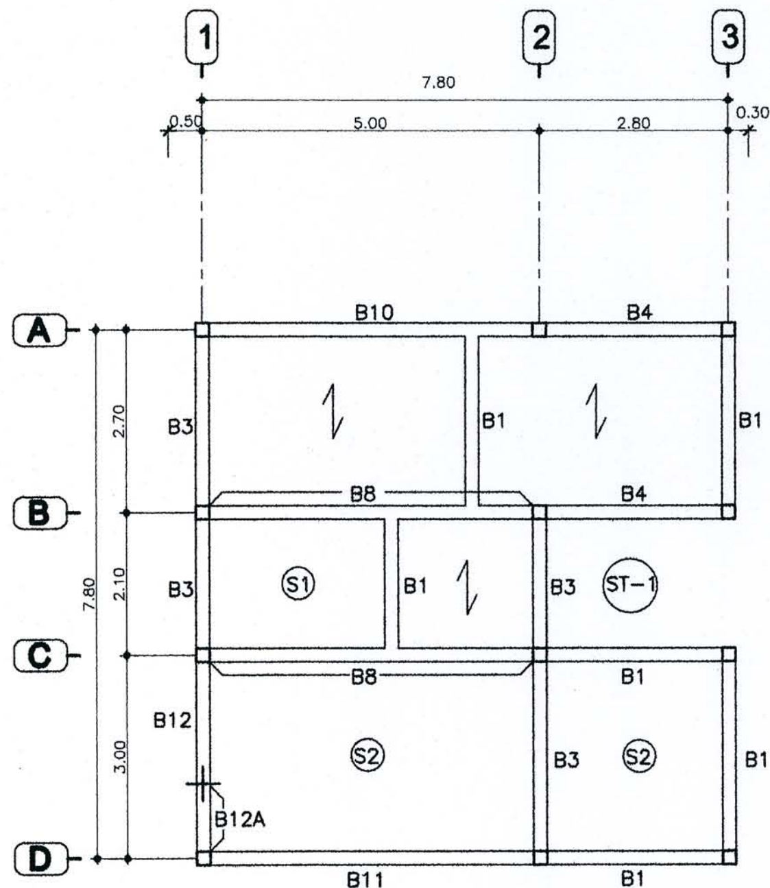
ผังโครงสร้าง ชั้น 3 มาตราส่วน 1:75
