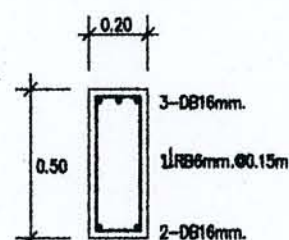
B6A ②-② 1:25
