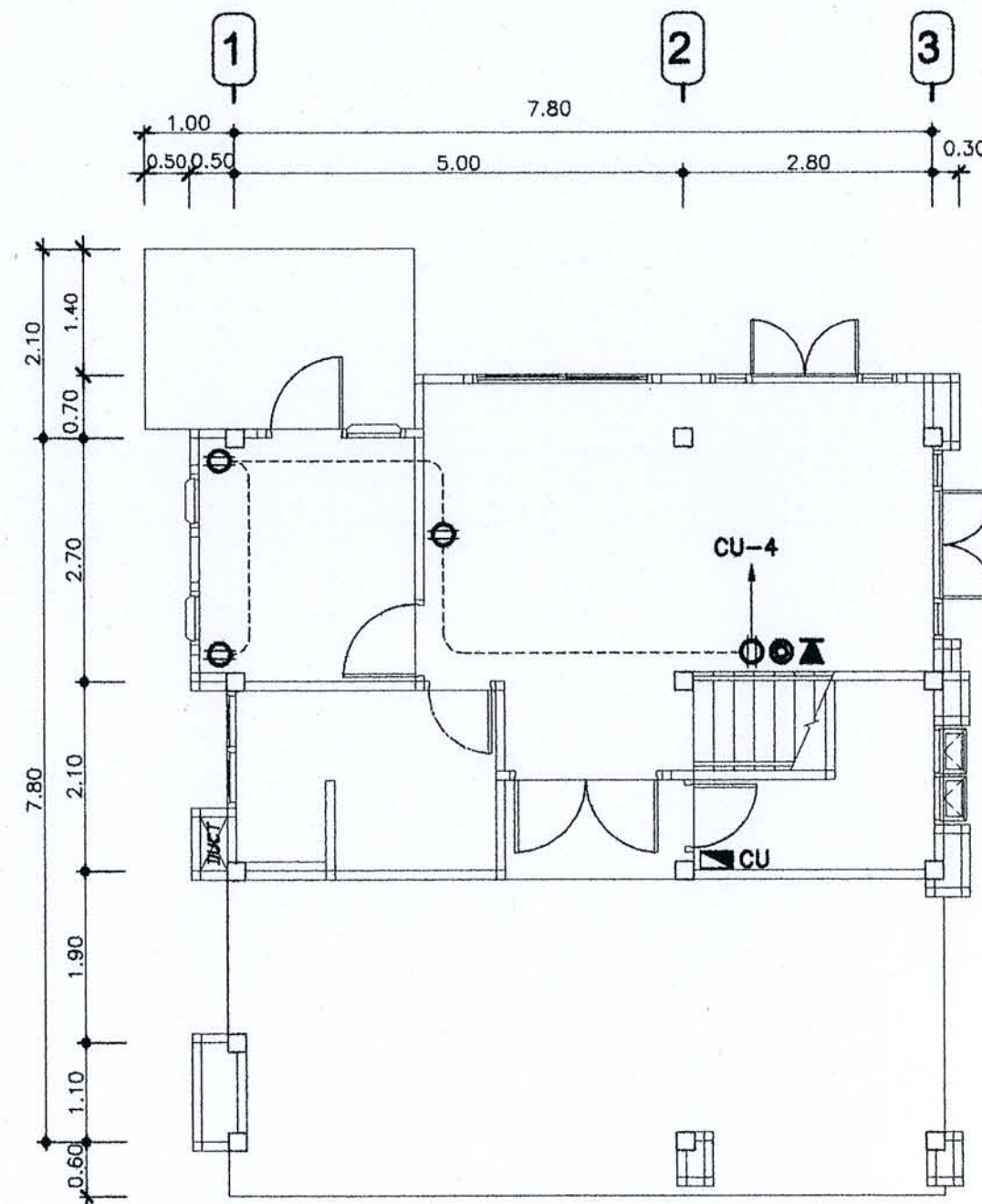
แปลนเดินไฟฟ้า โทรศัพท์ โทรทัศน์ ชั้นล่าง
