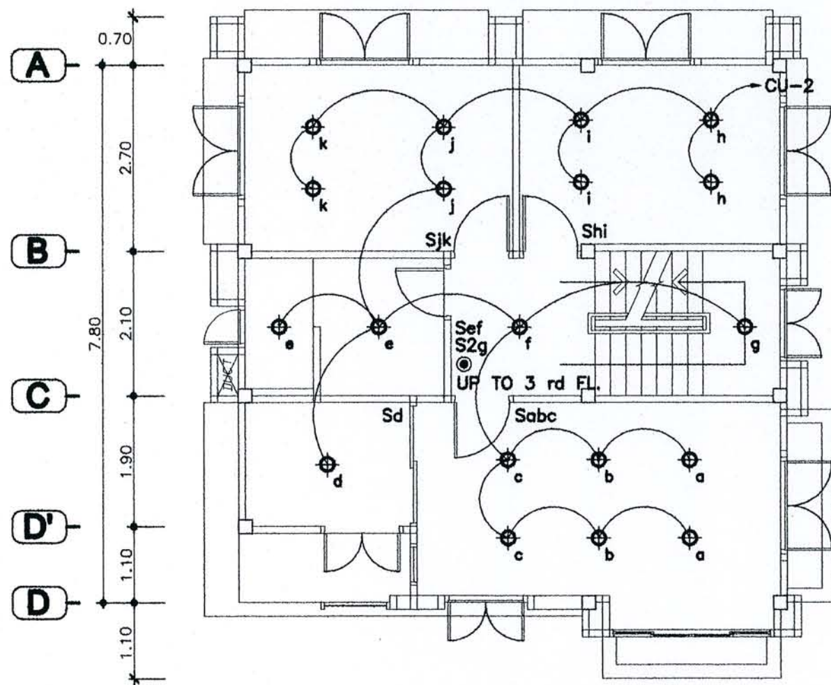
แปลนไฟฟ้าแสงสว่างชั้นที่ 2
