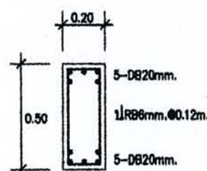
B9 1:25
