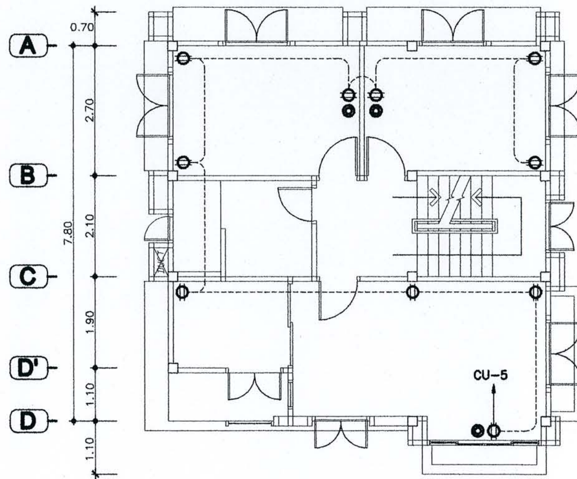
แปลนเดินไฟฟ้า โทรศัพท์ ชั้นที่ 2
