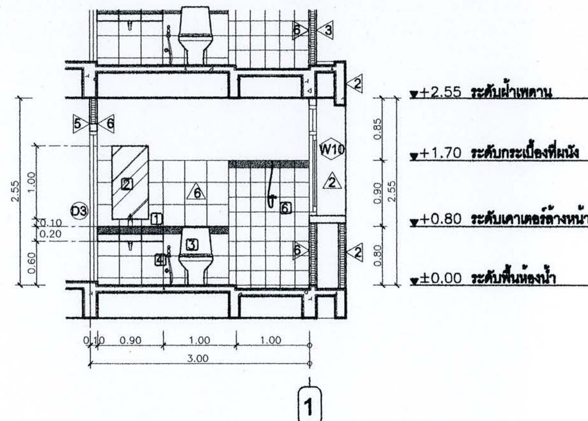
รูปตัด B-B
