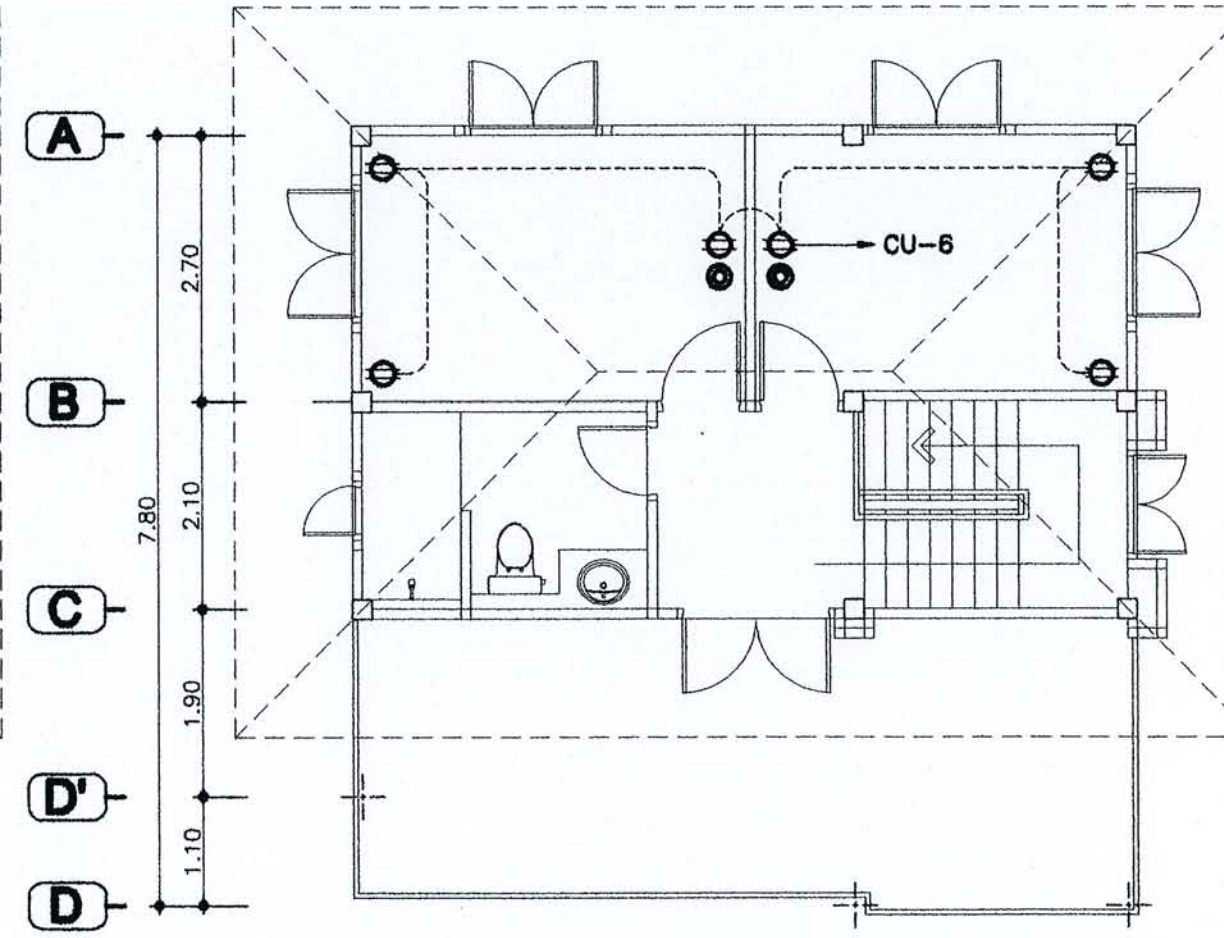
แปลนเดินไฟฟ้า โทรศัพท์ ชั้นที่ 3
