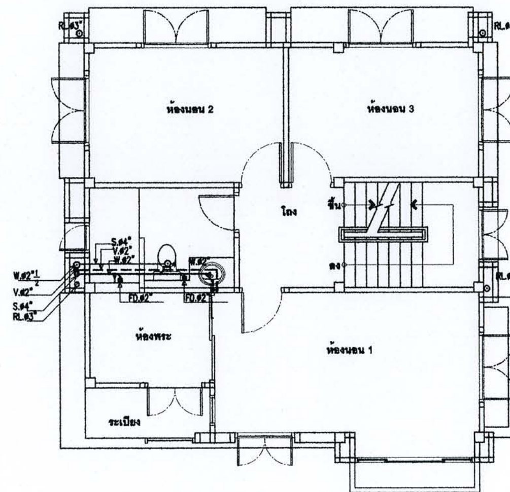
แปลนระบบสุขาภิบาลและท่อน้ำฝน ชั้น 2
