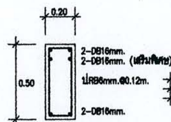
B7A ②-② 1:25
