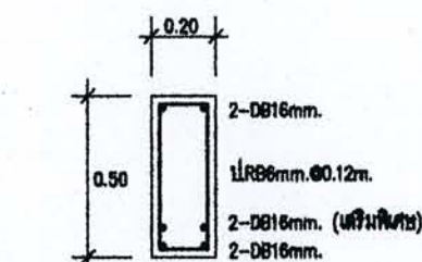
B7 ①-① 1:25
