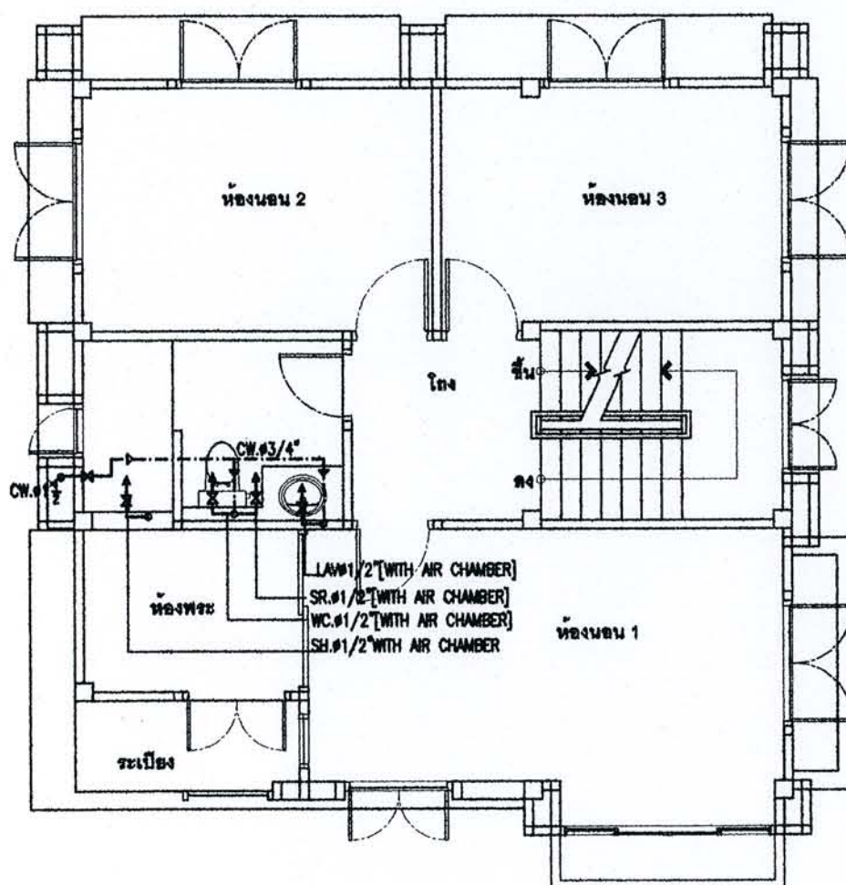
แปลนระบบท่อน้ำประปา ชั้น 2
