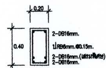
B12 ①-① 1:25
