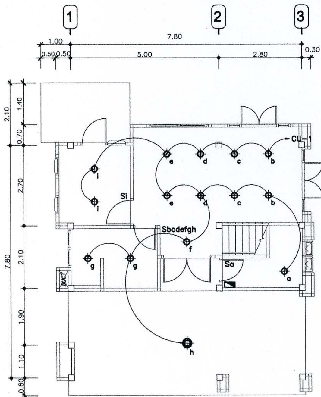
แปลนไฟฟ้าแสงสว่างชั้นล่าง
