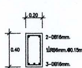
B11 1:25
