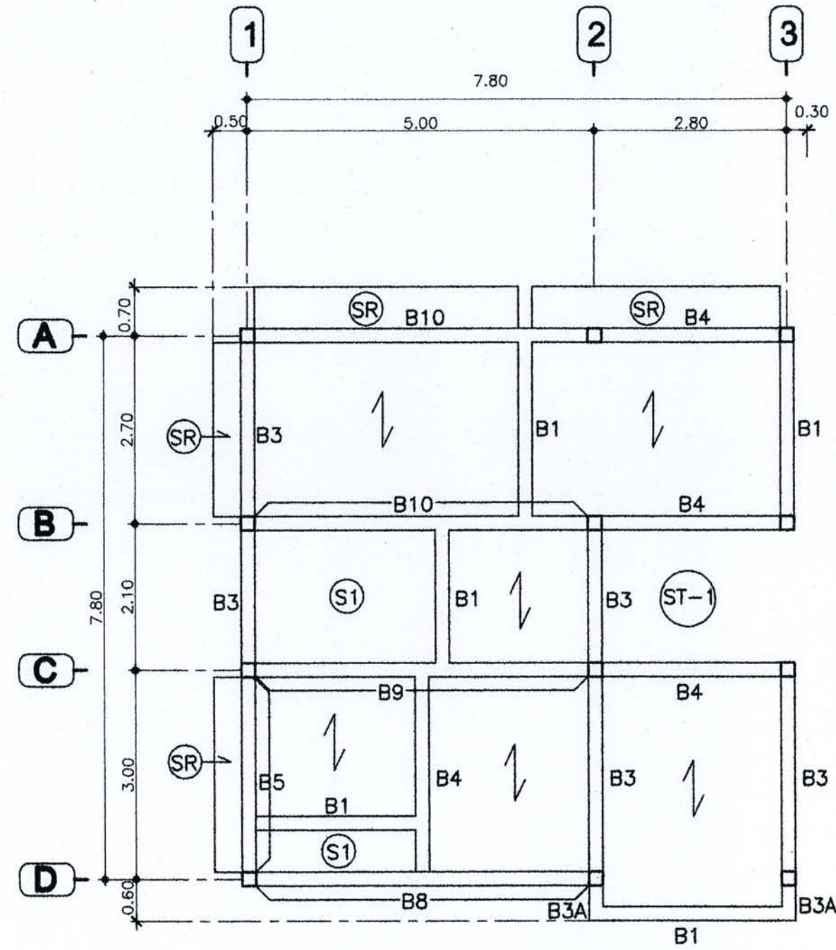
ผังโครงสร้าง ชั้น 2 มาตราส่วน 1:75
