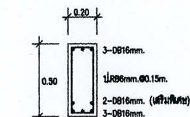
B6 ①-① 1:25
