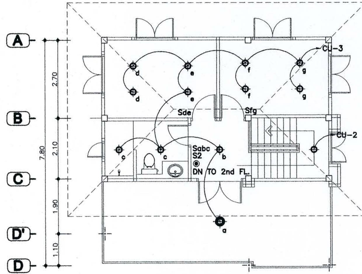
แปลนไฟฟ้าแสงสว่างชั้นที่ 3
