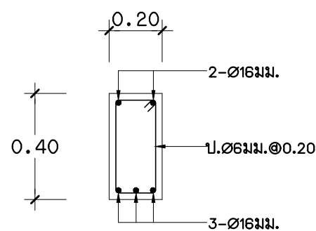
B3 1:20
