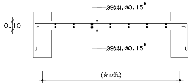
S2 1:20
