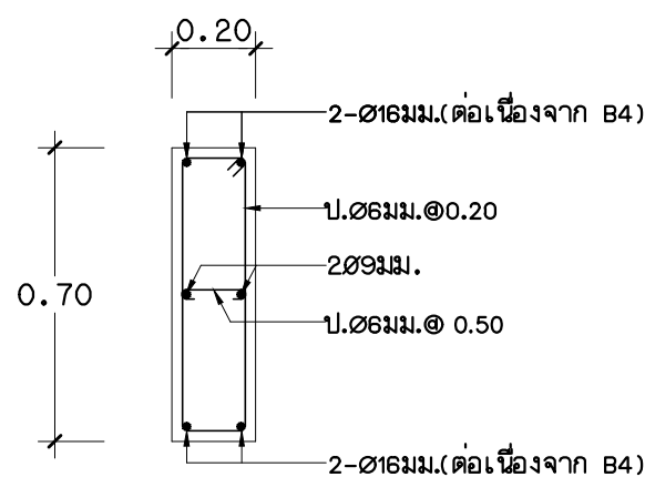
B4X 1:20
