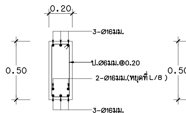
B5 1:20
