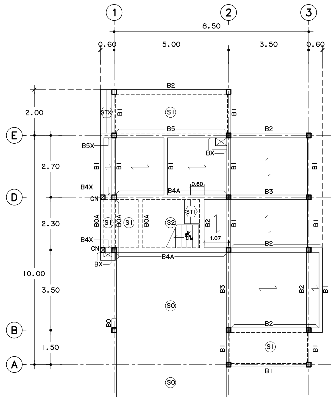
แปลนคาน, ฟันชั้น। มาตราส่วน 1:100
