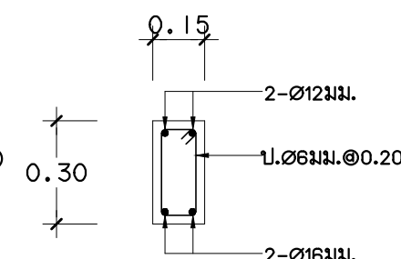
B0A 1:20
