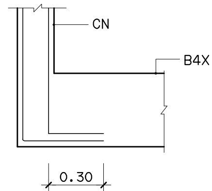
รอยต่อเสาคอนกรีต CN กับ คาน ค.ส.ล. 1:20
