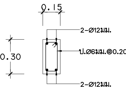
0-0 1:20
