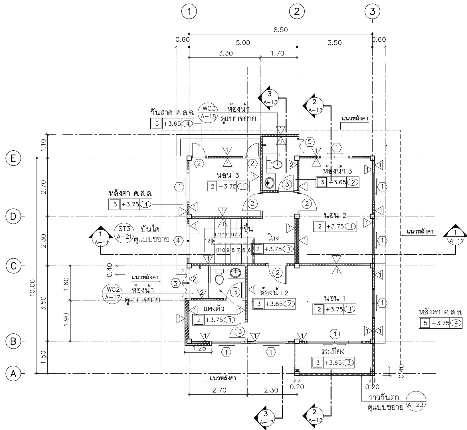
แปลนพื้นที่ 2
