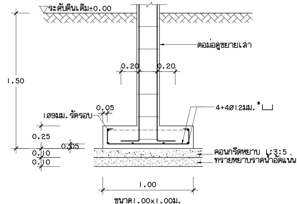
F1.00x1.00 1:25
