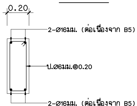
B1 1:20
