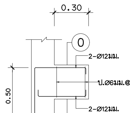
B0 1:20
