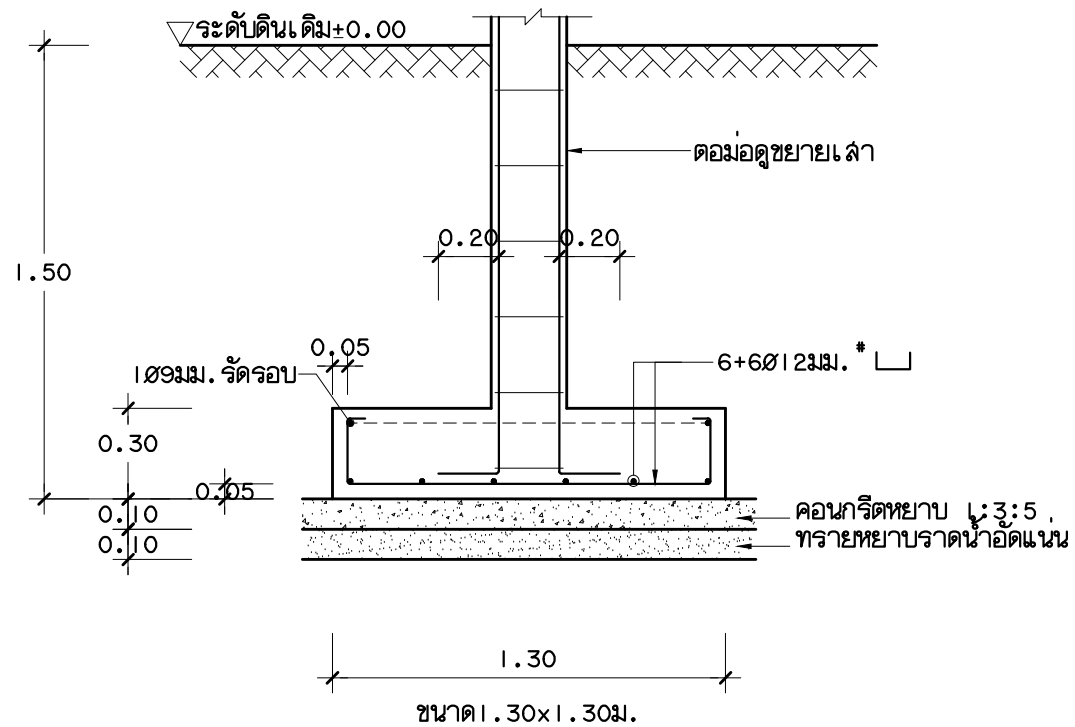
F 1.30x1.30 1:25
