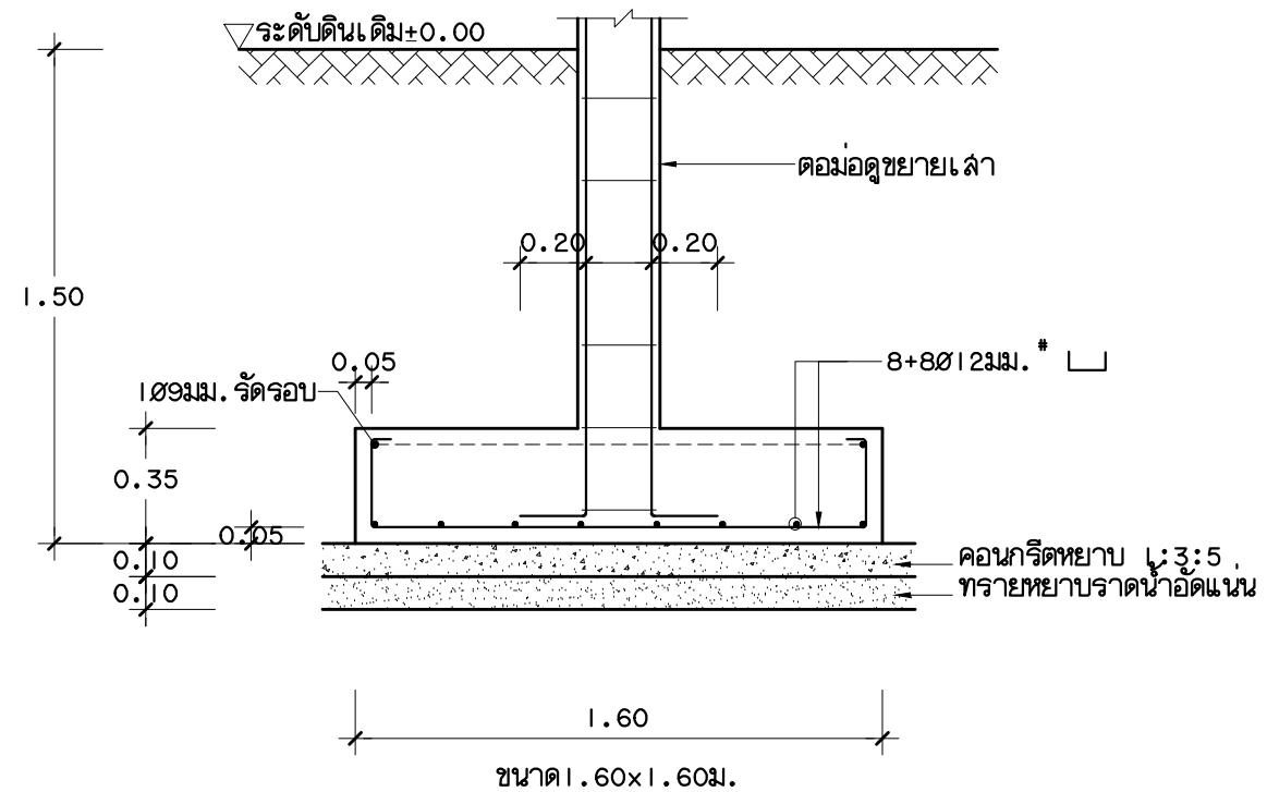
F 1.60x1.60 1:25
