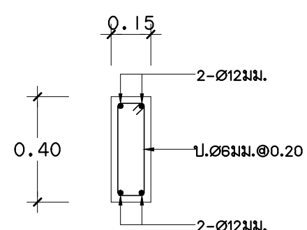
B1 1:20
