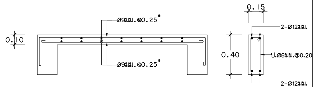
RB1 1:20
