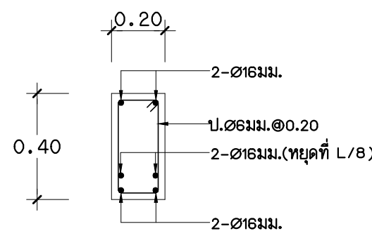
B0 1:20
