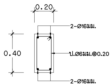
B2 1:20
