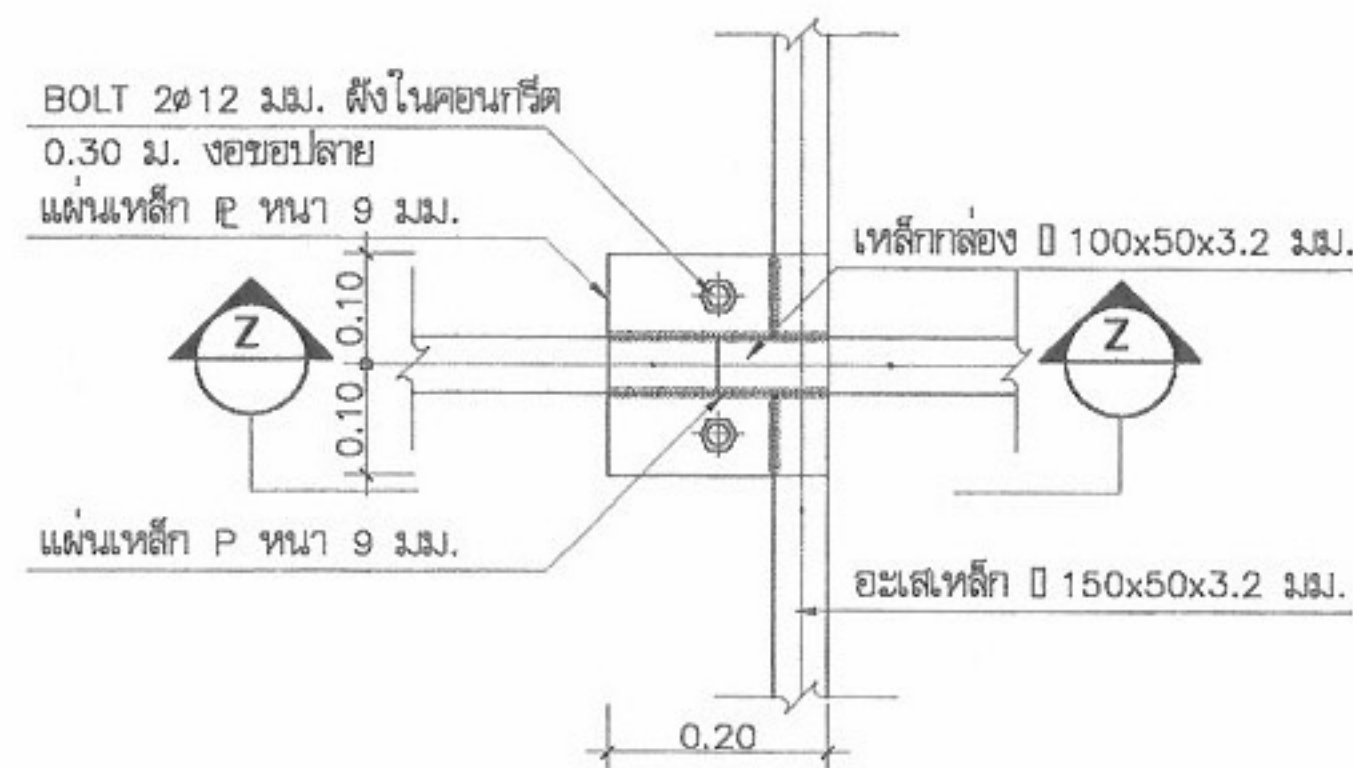
แบบขยายจุดต่อ ๑ มาตราส่วน 1:10
