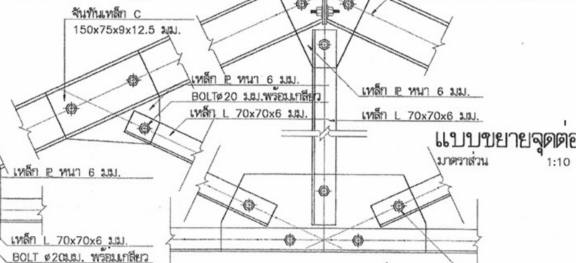
แบบขยายจุดต่อ ④ มาตราส่วน 1:10
