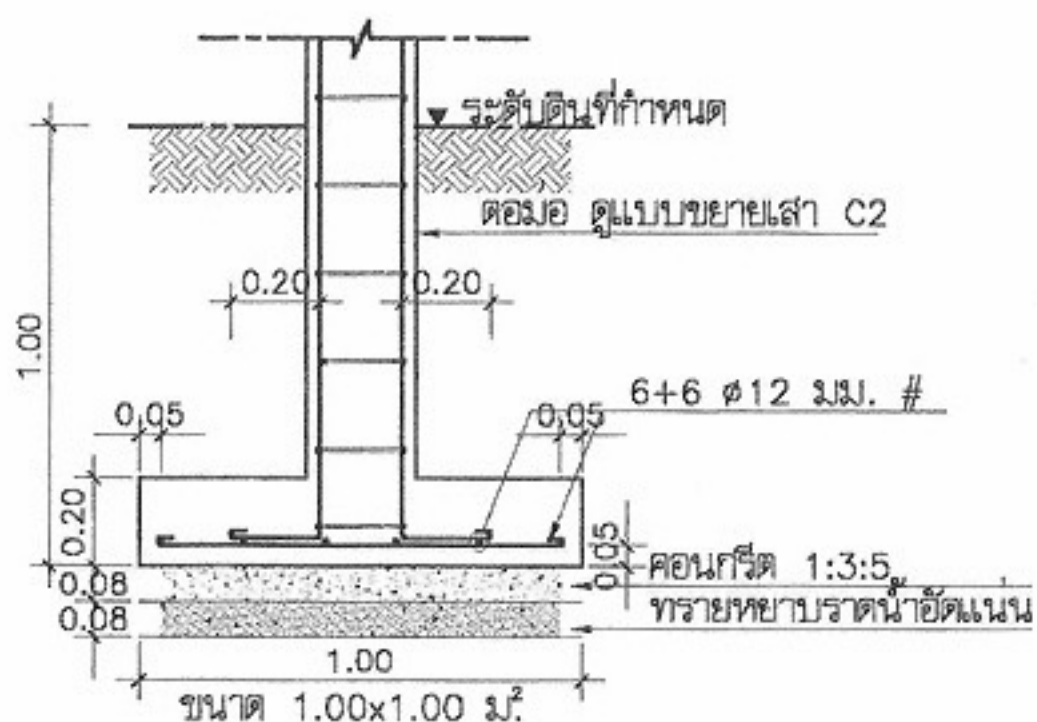
F3 1:25 (แบบฐานแผ่)
