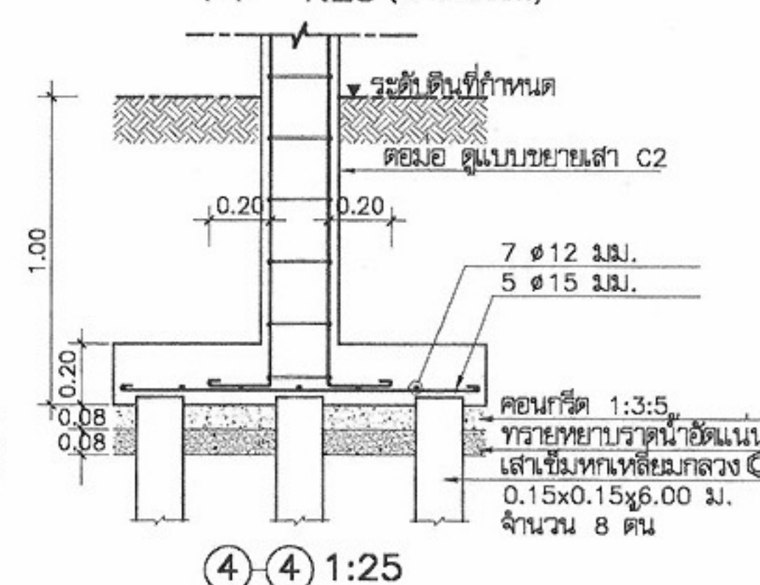
F4 1:25 (แบบตอกเข็ม)
