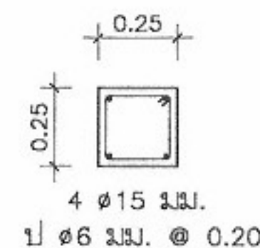
C-1 (ฐานราก-หลังคา)
