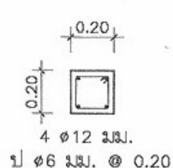
C-2 (ฐานราก-หลังคา)
