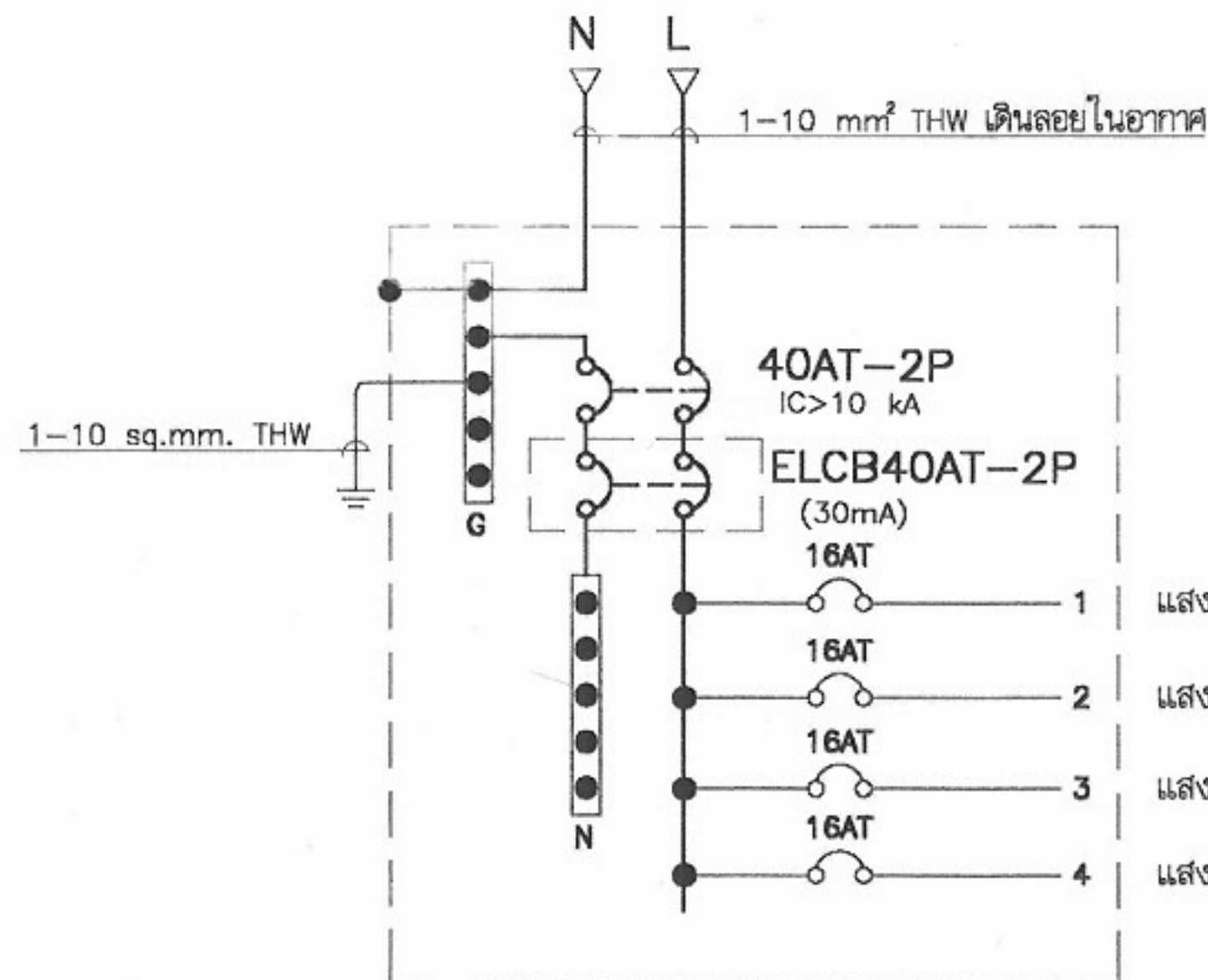
แผงสวิตช์ LP บ้านเรือนแถว
