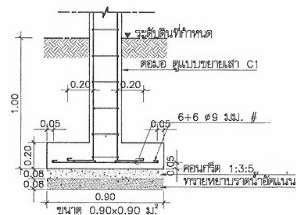
F1 1:25 (แบบฐานแผ่)
