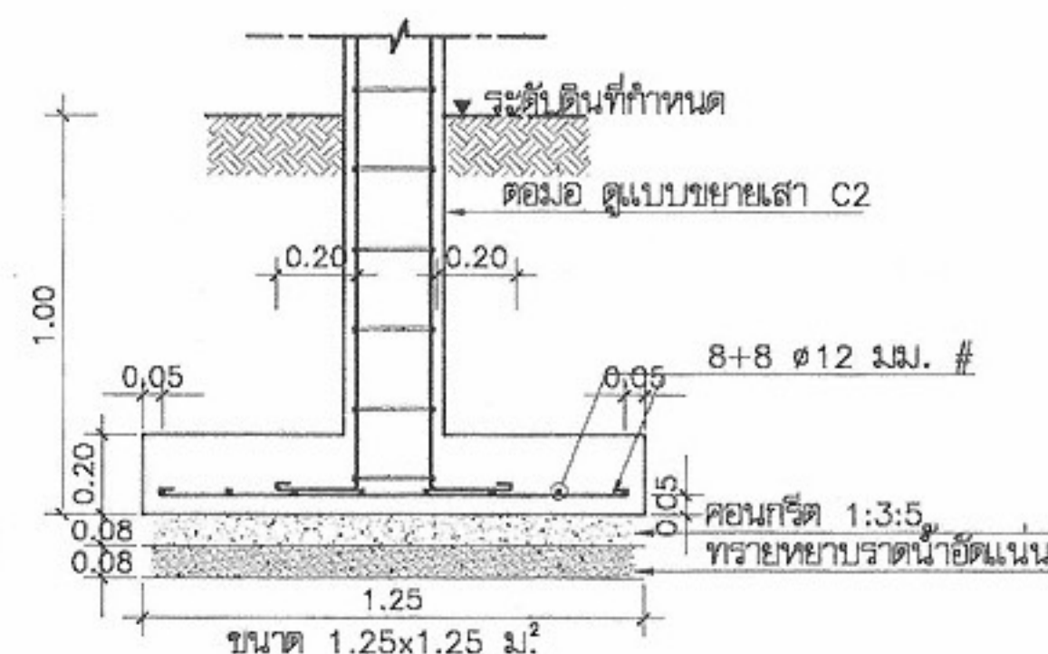
F4 1:25 (แบบฐานแผ่)
