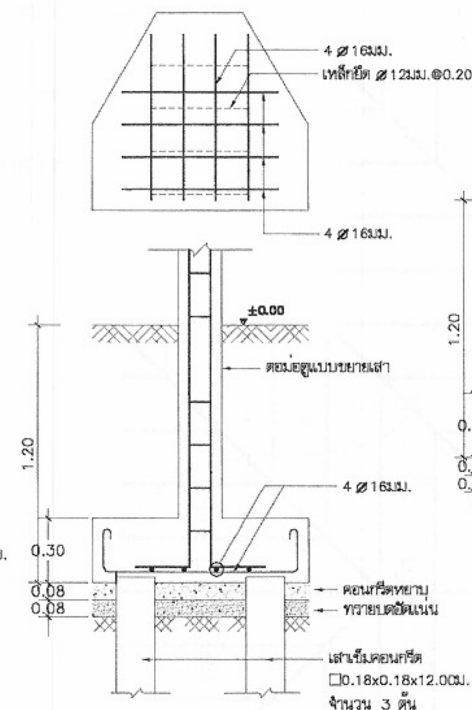
F 3 มาตราส่วน 1:25
