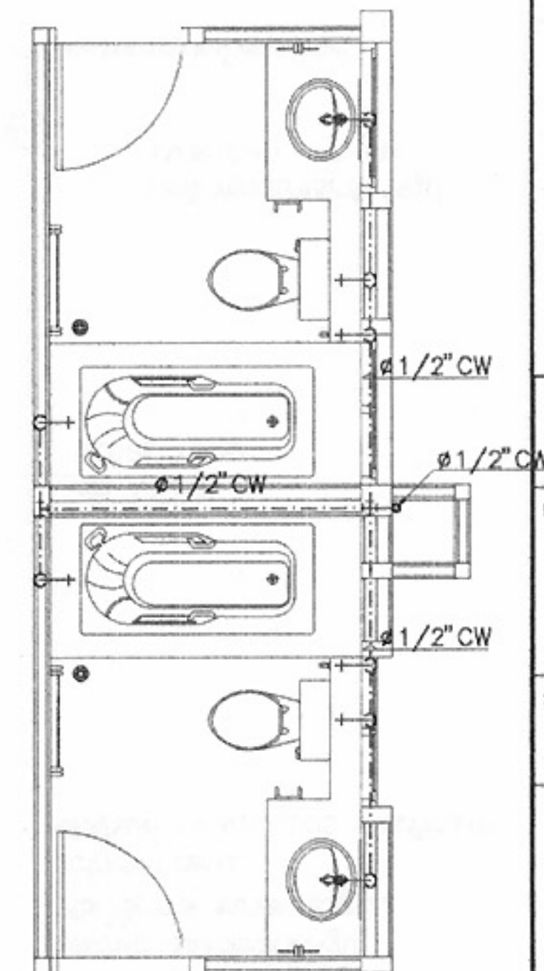
แปลนท่อน้ำดี มาตราส่วน 1:50
