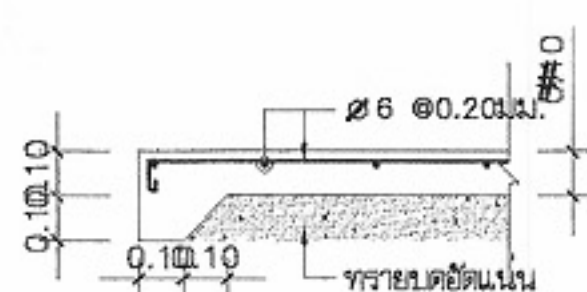
S0 มาตราส่วน 1:25
