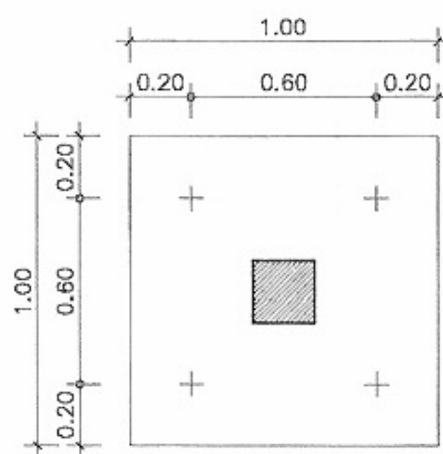
F 4 มาตราส่วน 1:25
