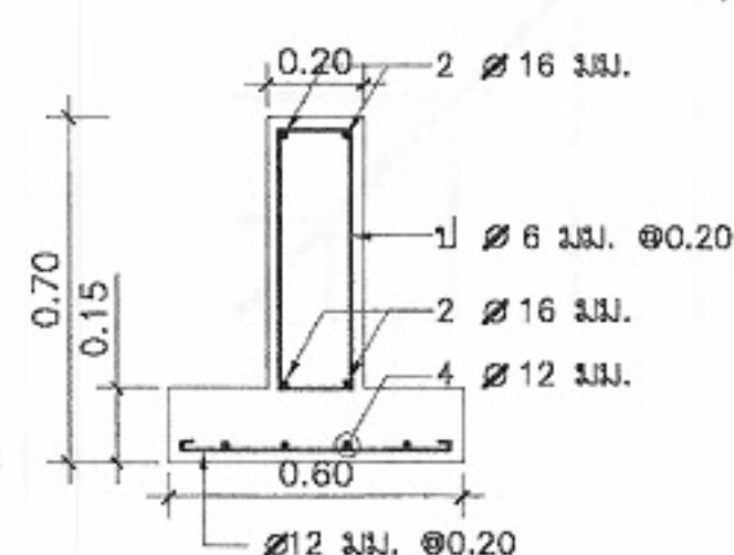
ขยายยกขอบ 1 : 25
