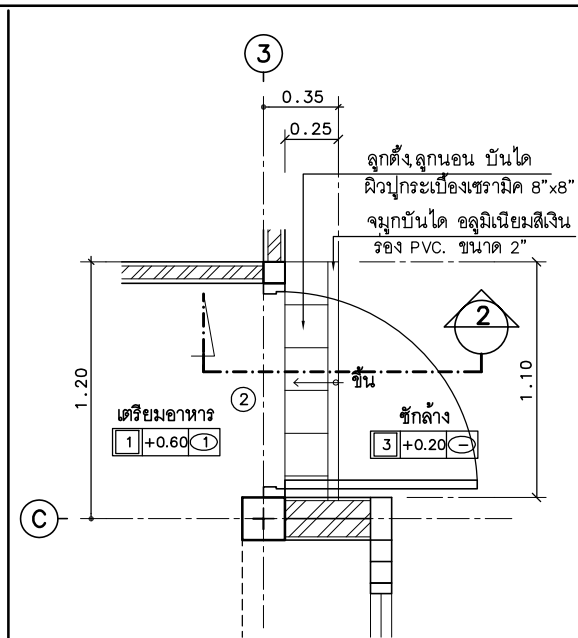
แปลนบ้าน ST.2
