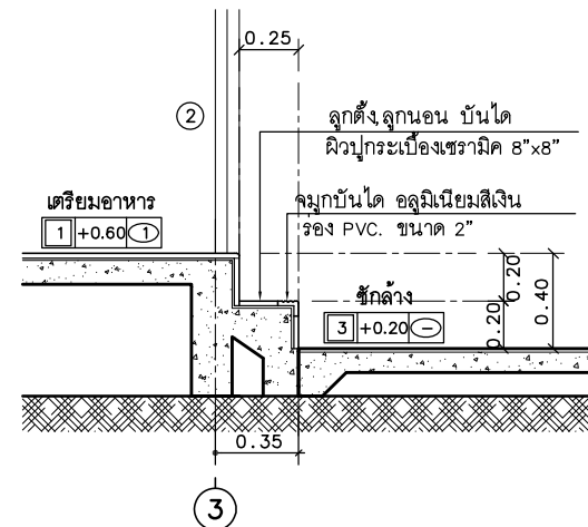
รูปตัดบ้าน ST.2
