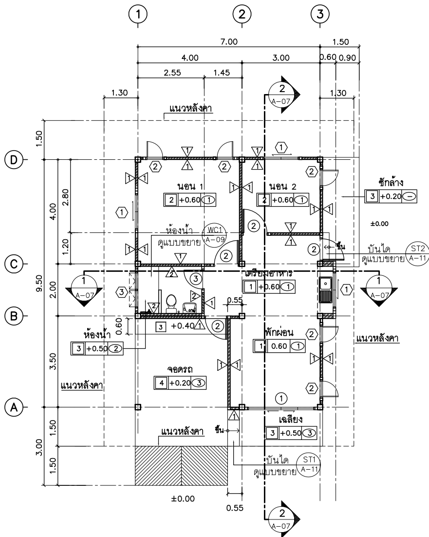
แปลนพื้นชั้น 1
