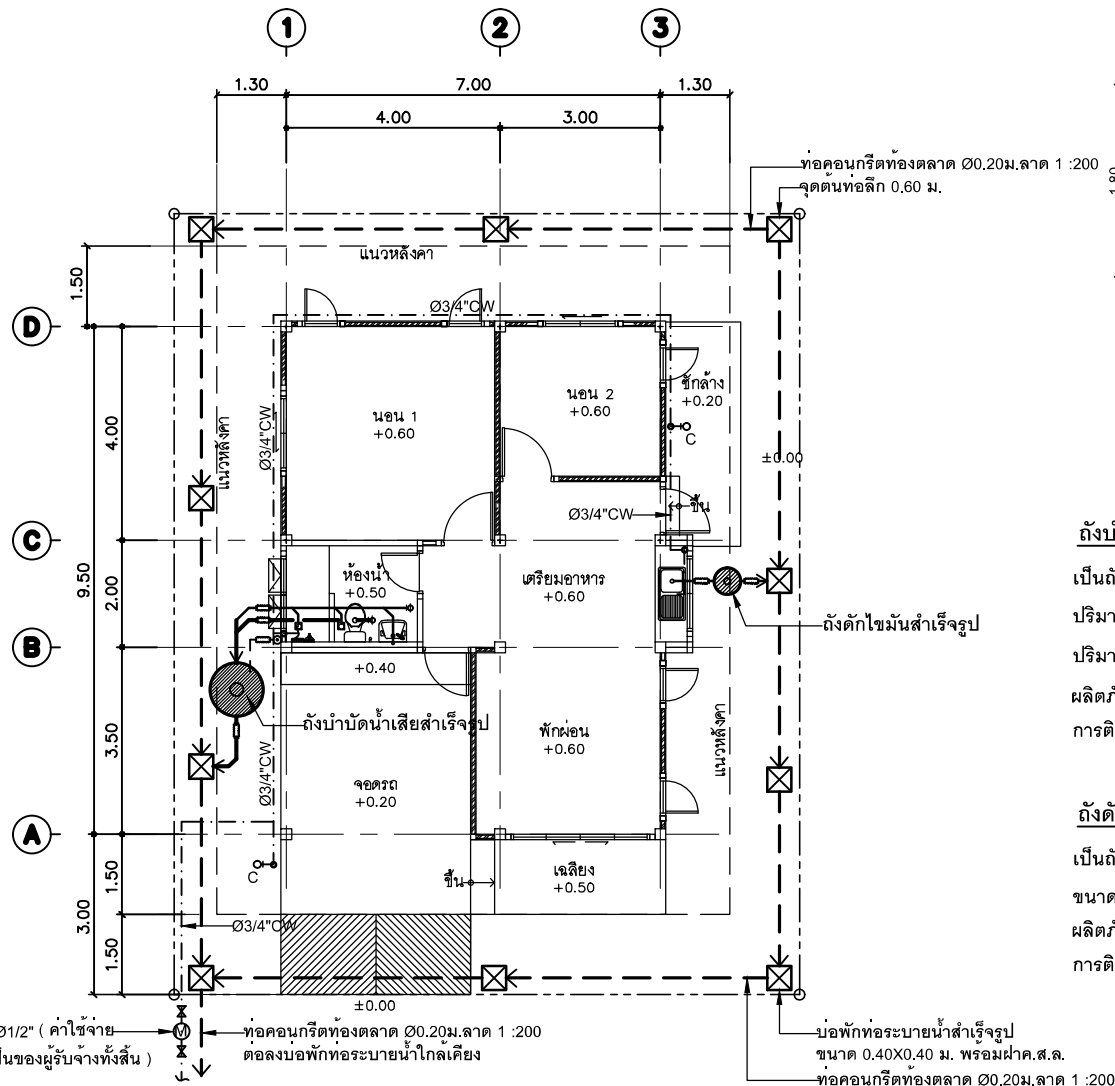
แปลนระบบสุขาภิบาลพื้น
