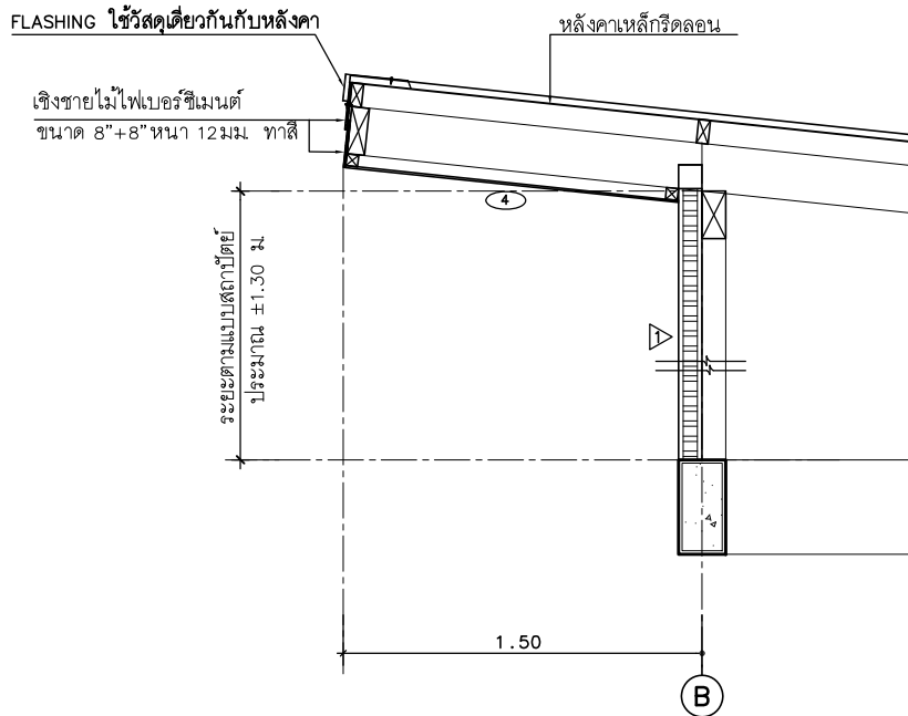
แบบขยาย เเชิงซ้าย 1
