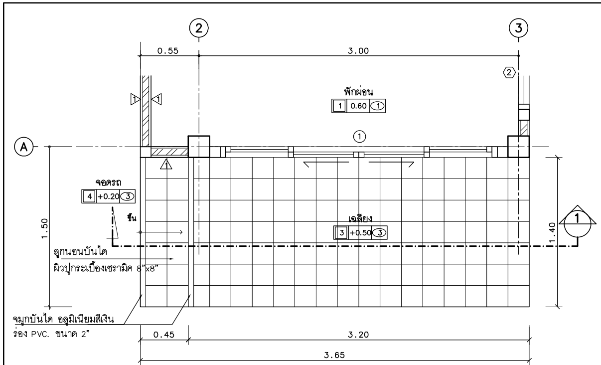
แปลนบ้าน ST.1
