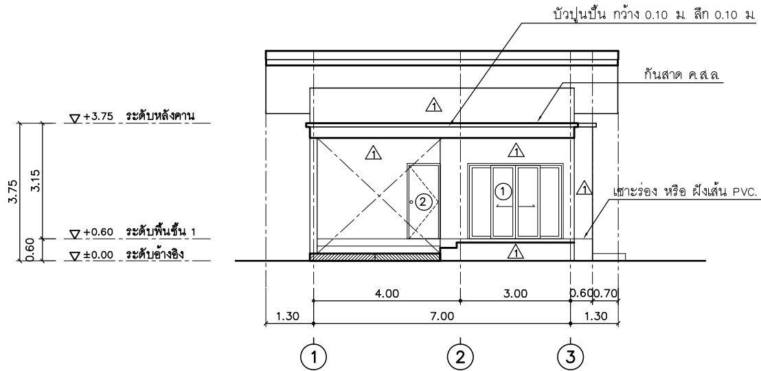
รูปด้าน 1
