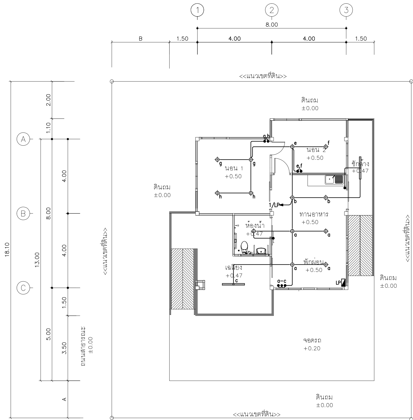
แผนผังไฟฟ้าแสงสว่าง 1:100
