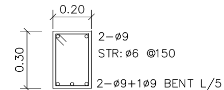
ขยายคานคอดิน
