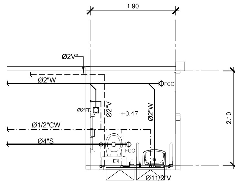
แปลนระบบสุขาภิบาลห้องน้ำ มาตราส่วน 1 : 50 ( ท่อประปาเดินใต้พื้น )
