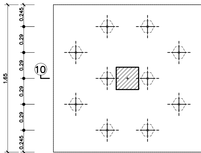
F10 1:25
