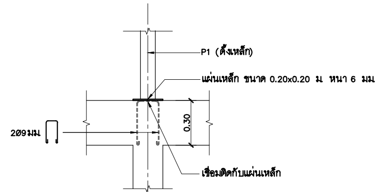
แบบขยายฐานรับตั้งเหล็ก (P1) 1:25
