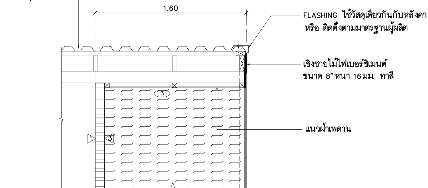
แบบขยายหลังคา มาตราส่วน 1 : 25 3 A-15
