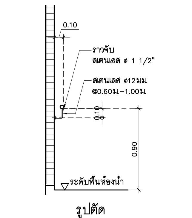
แบบขยายราวจับเพื่อนำไปสู่สุขภัณฑ์
