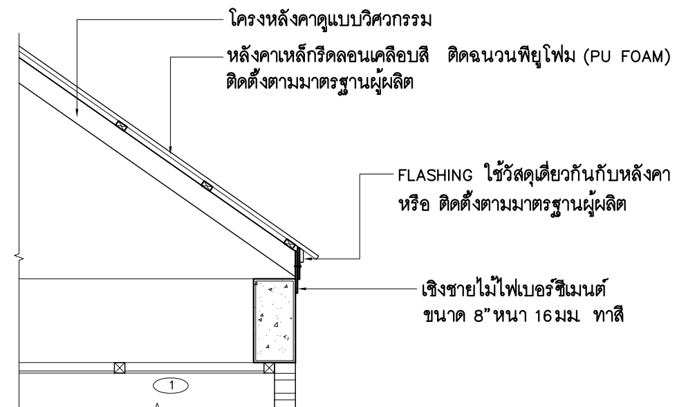
แบบขยายหลังคา มาตราส่วน 1 : 25 2 A-15
