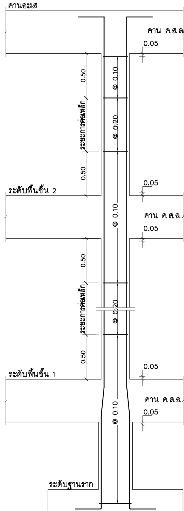
รายละเอียดการเสริมเหล็กปลอกในเสา
