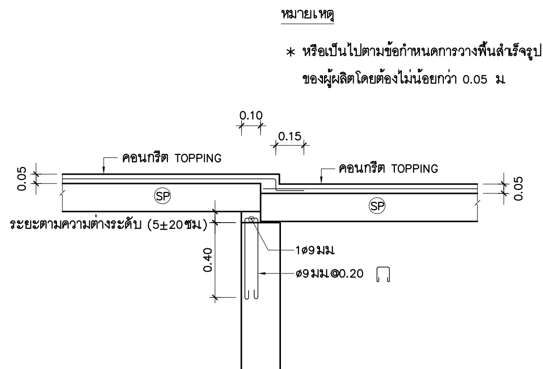
ลักษณะการหล่อพื้นเสริมกรณีสืบช่องว่างที่คานริม มาตราส่วน 1: 20
