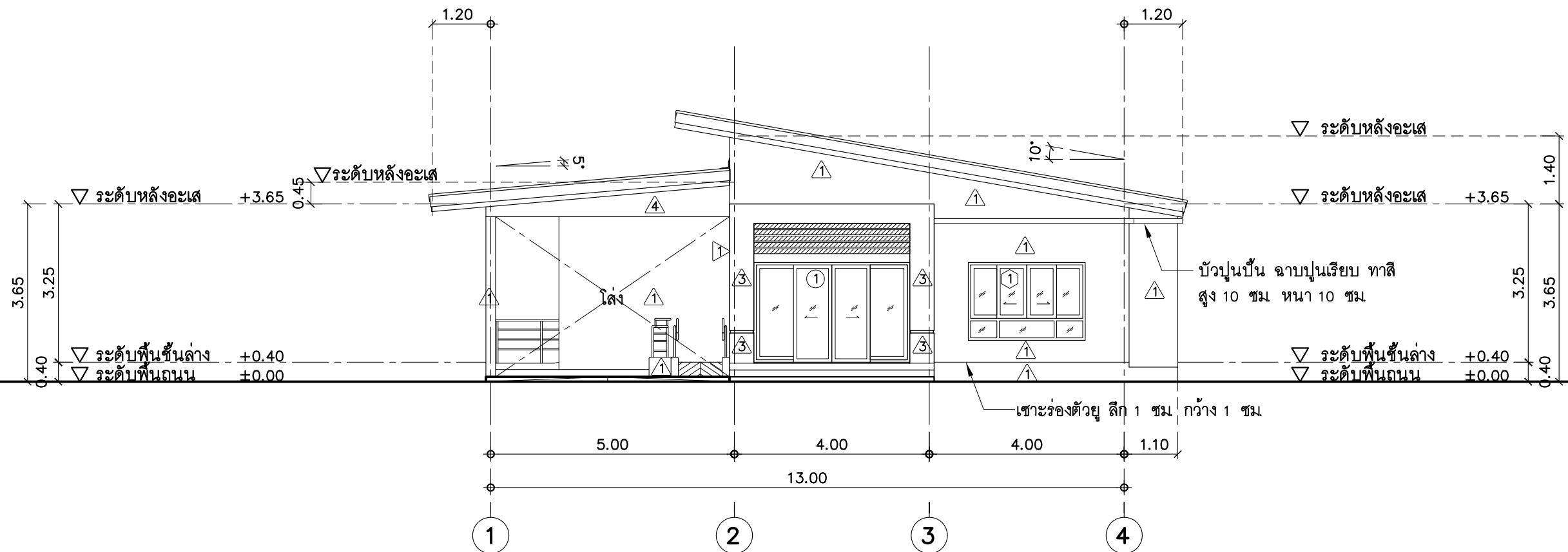
รูปด้าน
