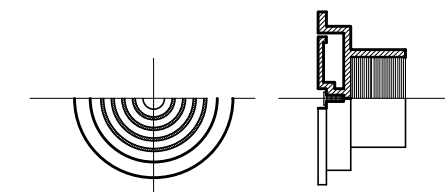
แบบขยายฝักบัวท่อระบายอากาศเหล็กหล่อชนิดออกด้านข้าง ( AVC )
