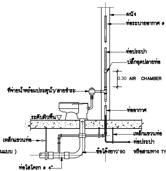
ส่วนชนิดประตูล้าง ( FLUSH VALVE )
