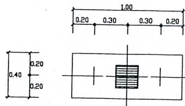
PLAN F2
