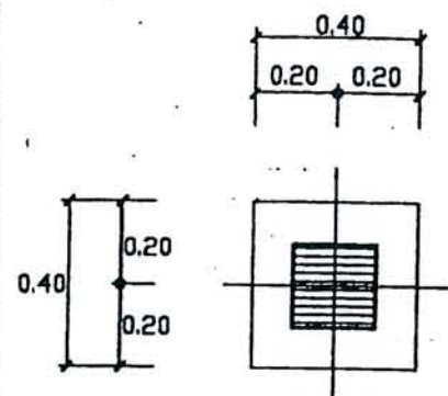
PLAN F1A
