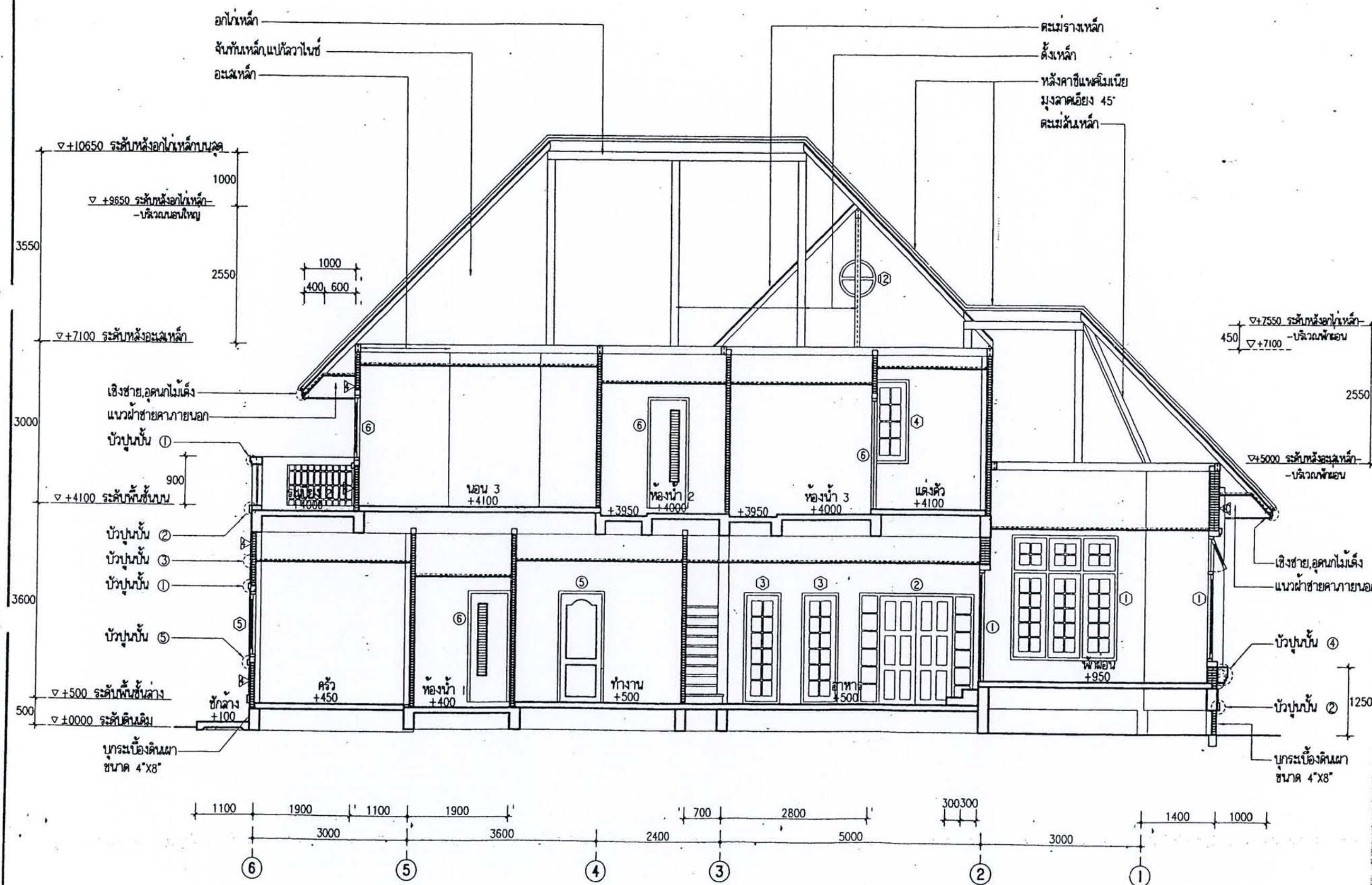
รูปตัด B-B มาตรฐาน 1:75
