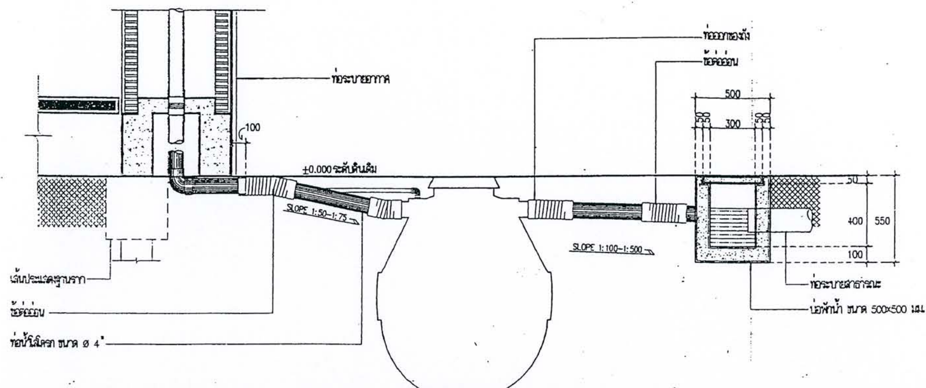
แบบขยายการวางท่อและตั้งระดับถังบำบัดลําเรือรูป มาตรฐาน 1 : 25
