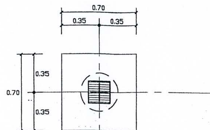
PLAN F1
