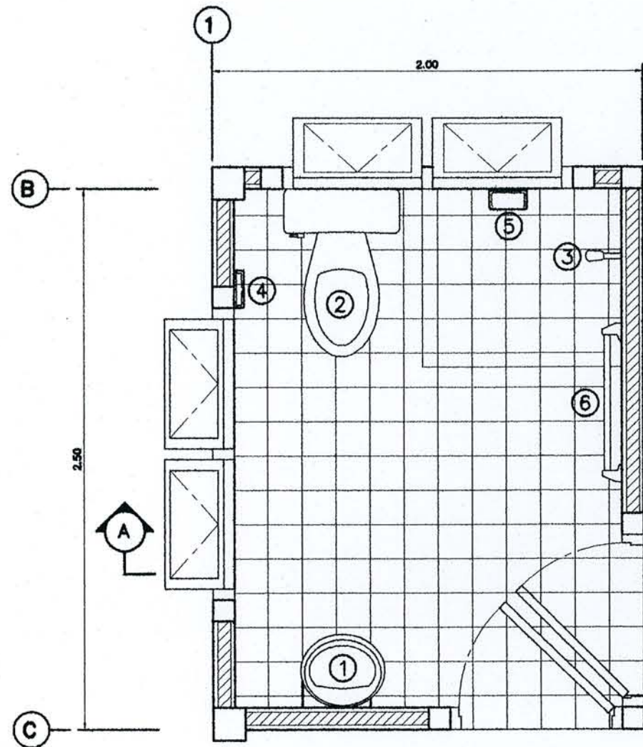
ขยายห้องน้ำ 1 มาตราส่วน 1 : 25
