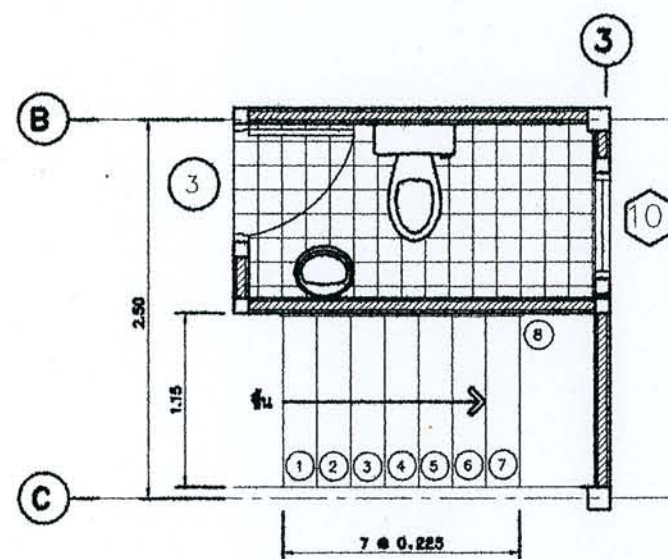
ขยายบันไดชั้นล่าง
