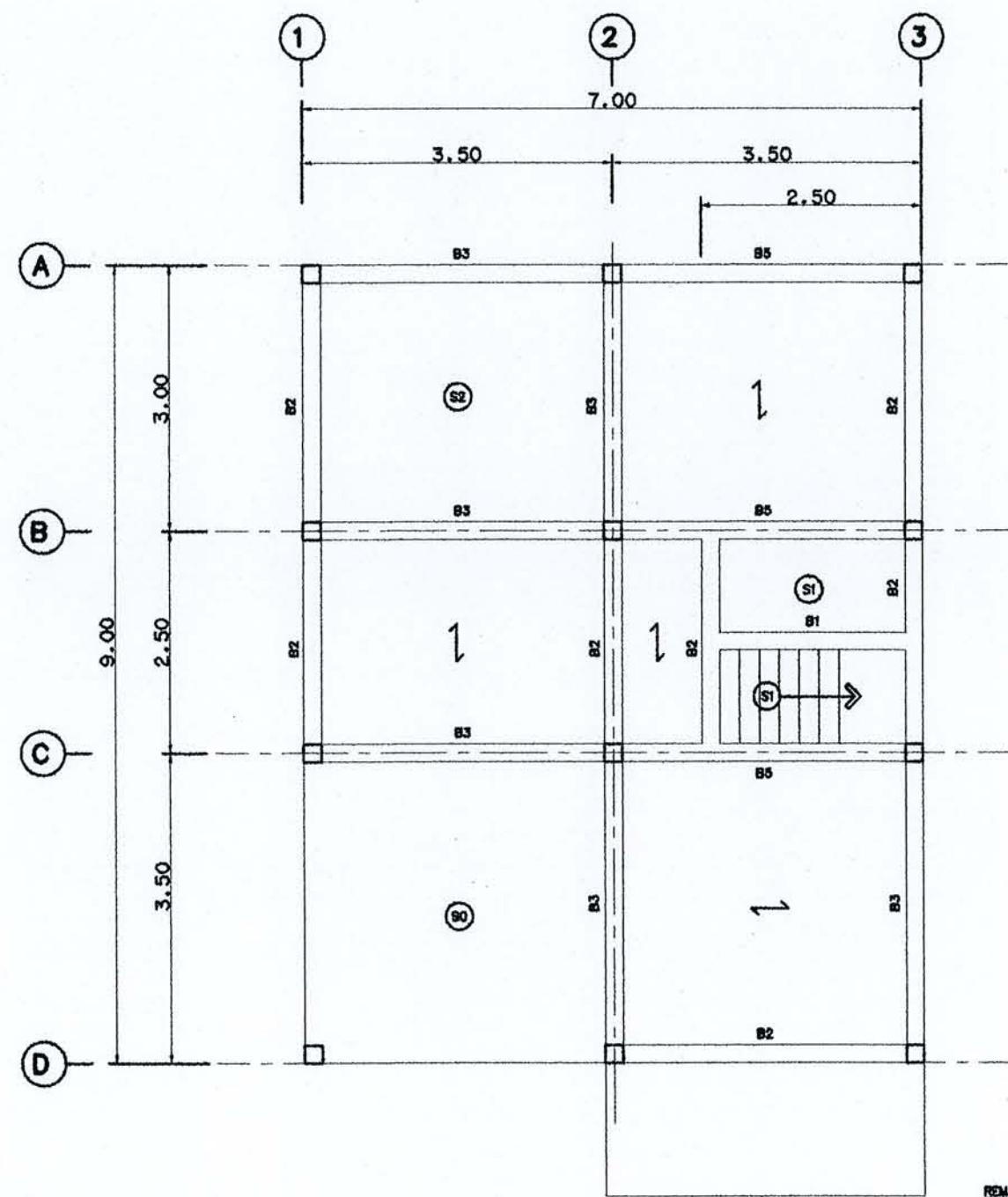
แปลนคานพื้นชั้นล่าง มาตราส่วน 1 : 75
