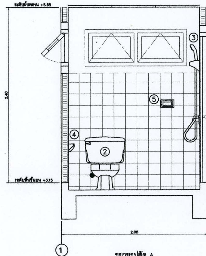
ขยายรูปตัด A มาตราส่วน 1 : 25
