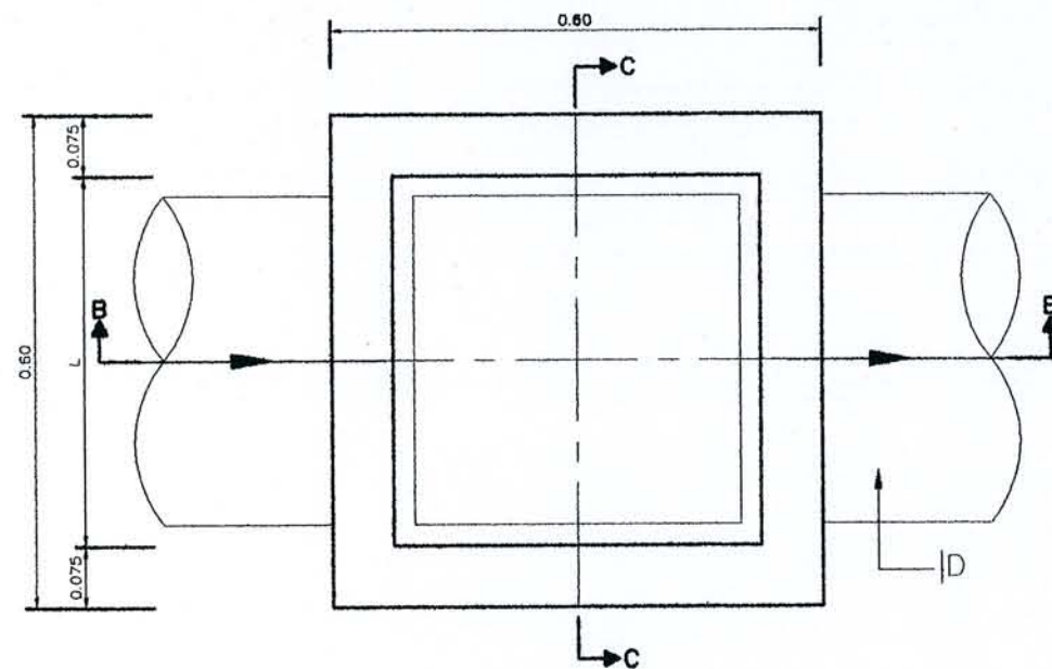
แบบขยายบ่อพักสำหรับรูปมาตรฐาน มาตราส่วน 1:10
