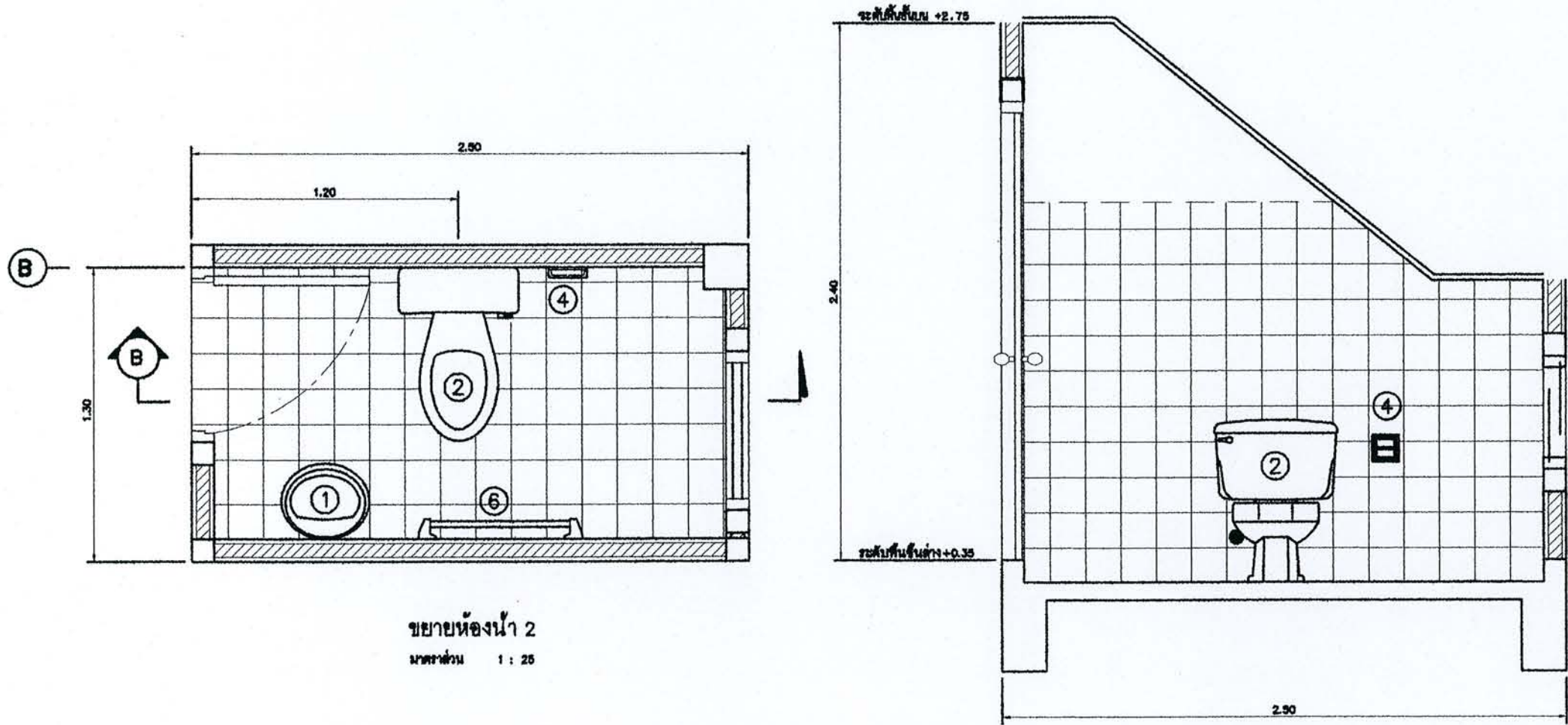
ขยายรูปตัด B มาตราส่วน 1 : 25
