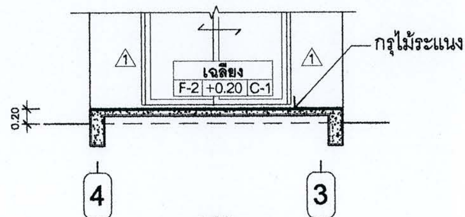
รูปตัด B
