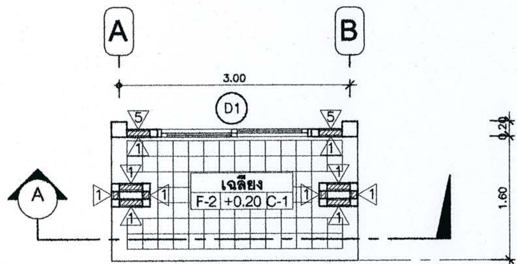
แบบขยายเจดียงหน้าบ้าน
