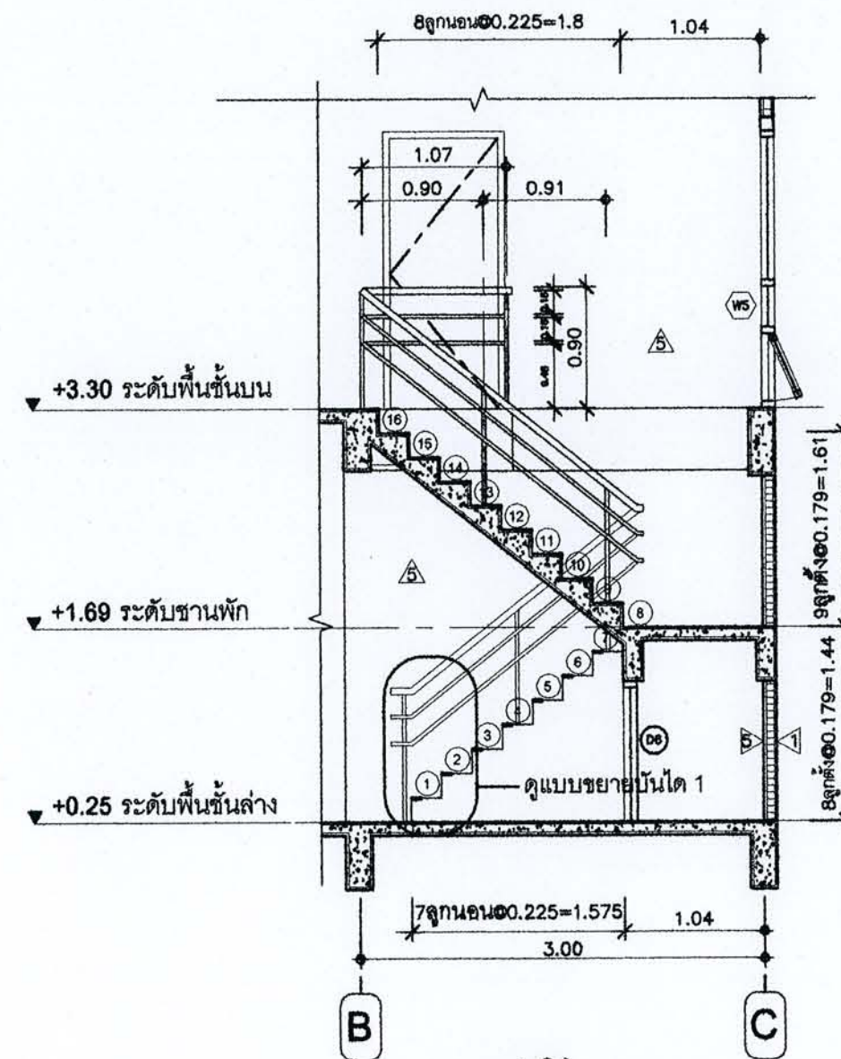
รูปตัด A
