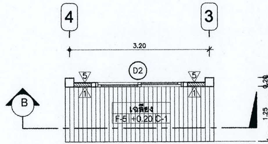
แบบขยายเจดียงห้องทานอาหาร
