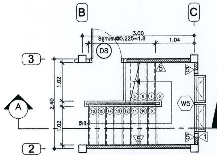
แบบขยายบันไดชั้นบน
