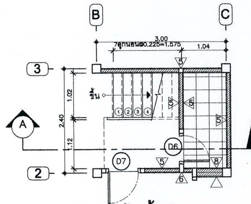
แบบขยายบันไดชั้นล่าง
