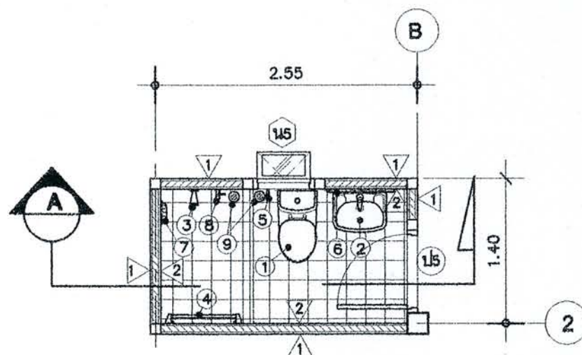
แปลนขยายห้องน้ำ ② มาตราส่วน 1 : 50
