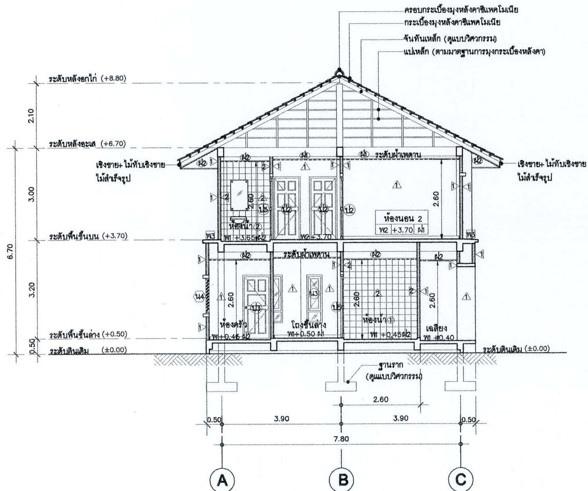
รูปตัด ก-ก มาตราส่วน 1 : 75
