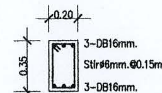
DETAIL B5
