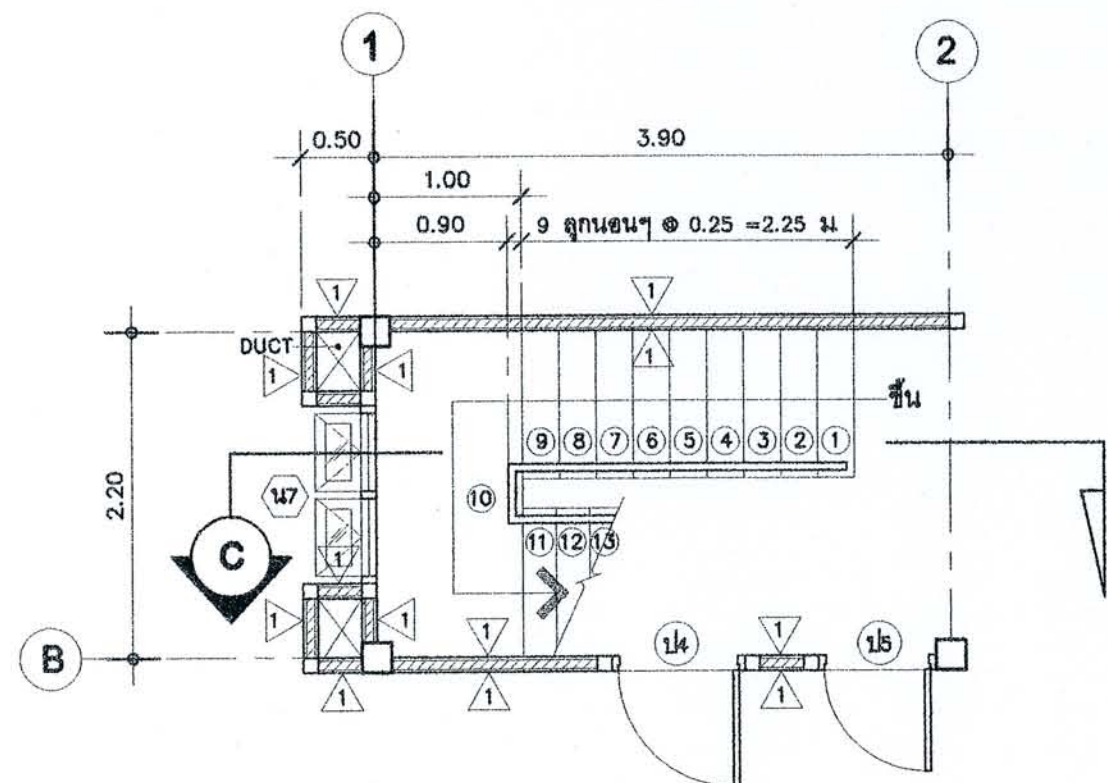
แปลนขยายบันไดชั้นล่าง
