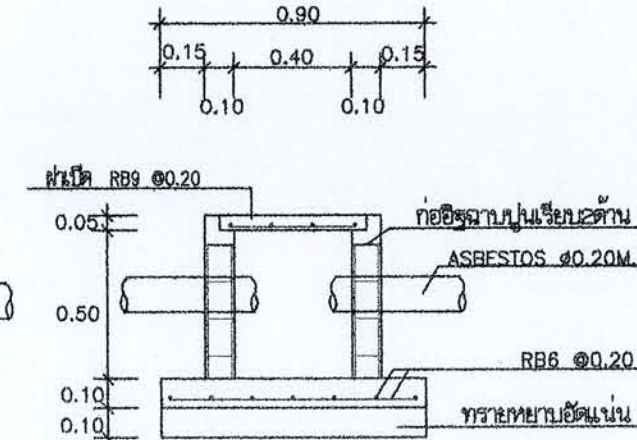
รูปตัดขยายบ่อพัก
