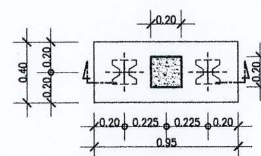
แบบขยาย F2
