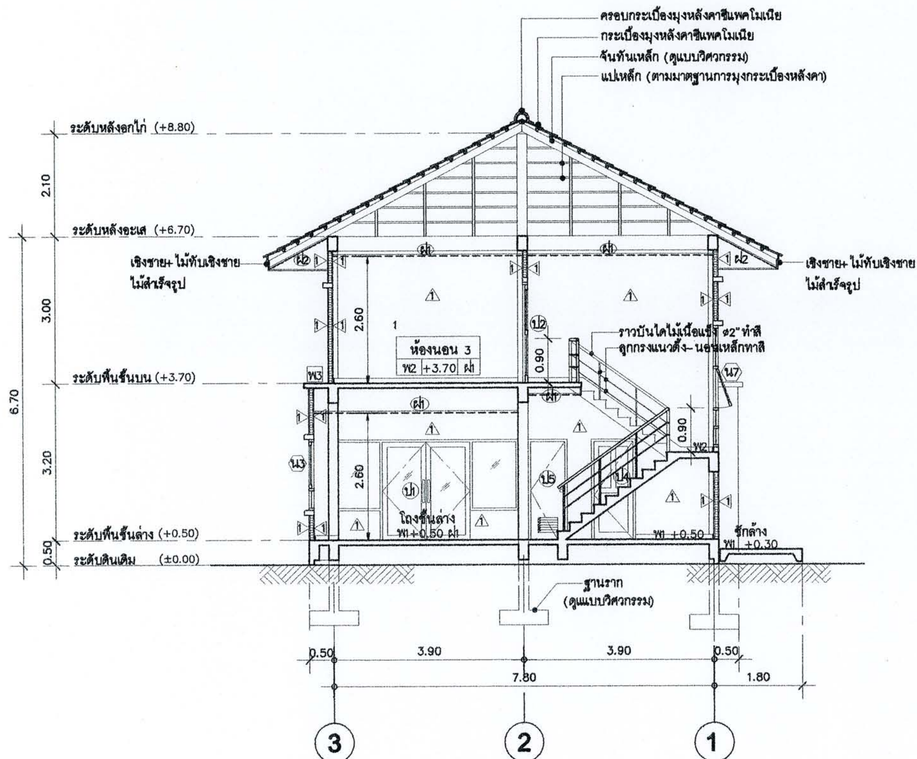
รูปตัด ข-ข มาตราส่วน 1 : 75
