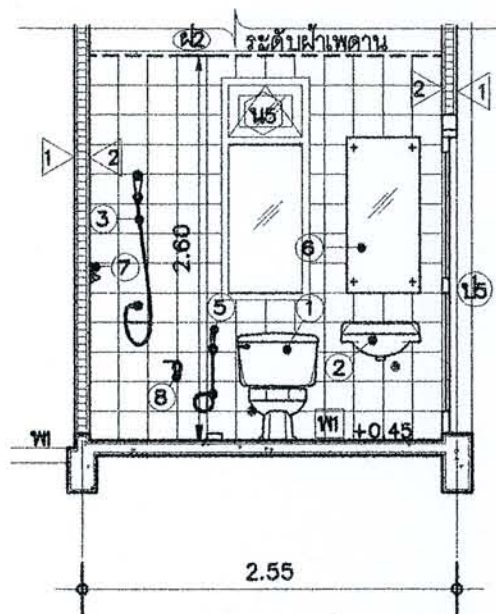
รูปตัด A - A มาตราส่วน 1 : 50
