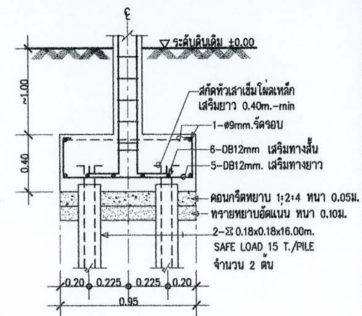
รูปตัด F2
