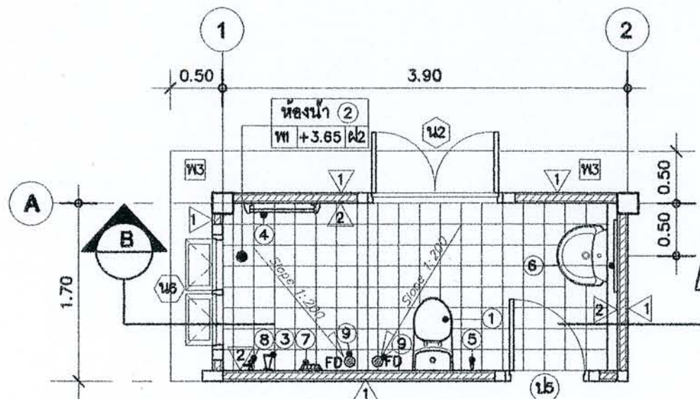
แบบขยายห้องน้ำ ① และ ② มาตราส่วน 1 : 50
