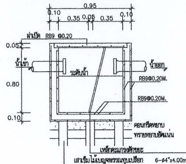
รูปตัดขยายบ่อพักขยะ
