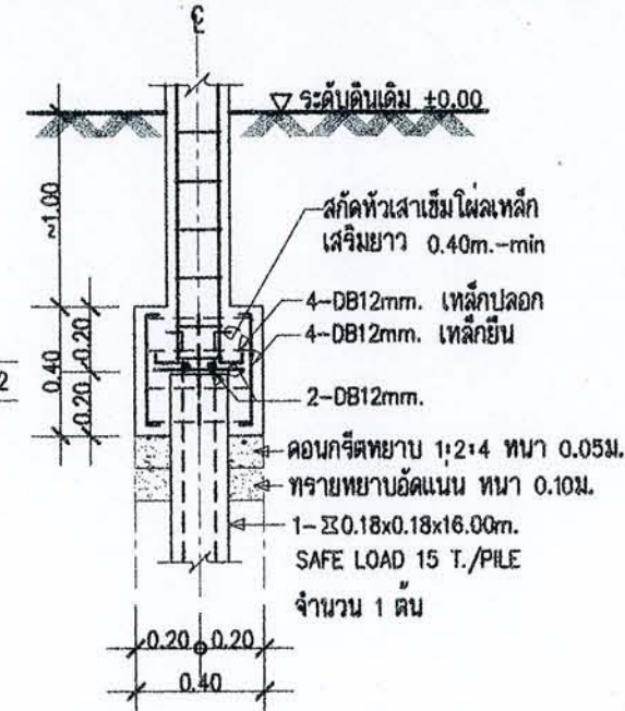
รูปตัด F1
