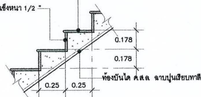
แบบขยายขึ้นบันได
