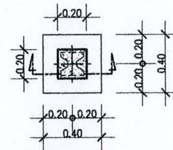
แบบขยาย F1
