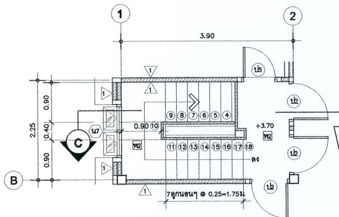
แปลนขยายบันไดชั้นบน
