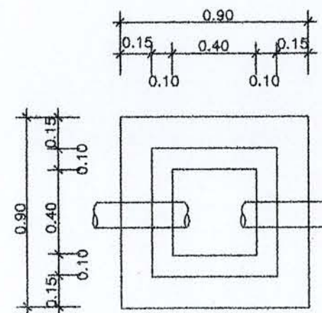
แปลนขยายบ่อพัก
