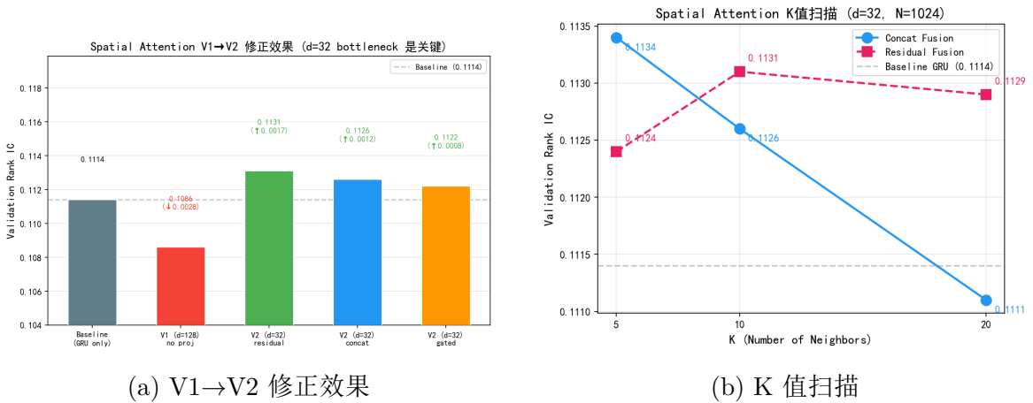
图 4: 空间注意力机制的设计迭代
