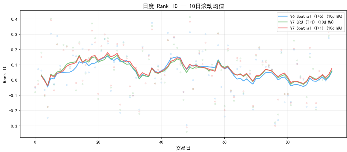
图 12: 路线 A 日度 Rank IC 时序（10 日滚动均线叠加）
