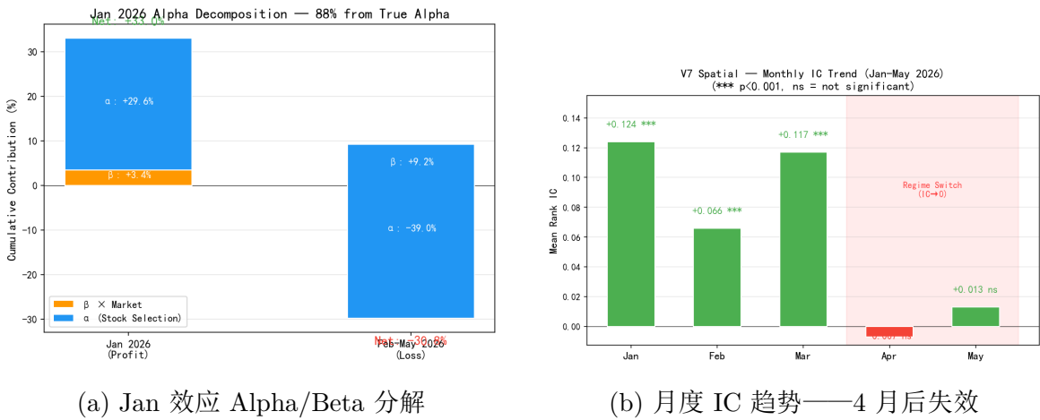
图 7: V9 效应诊断
