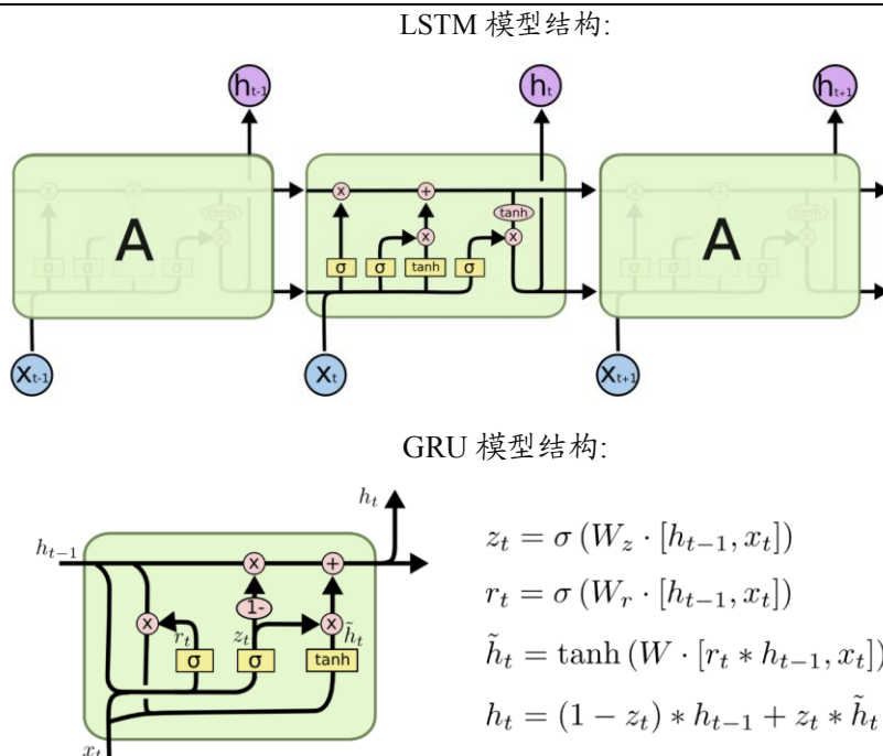
图 2: LSTM、GRU 模型结构
