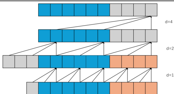
图 4: 扩张卷积
