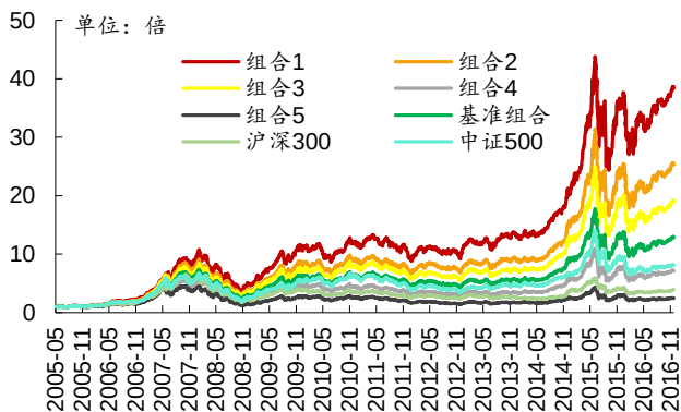
图表96: exp_wgt_return_6m 因子分层组合回测净值
