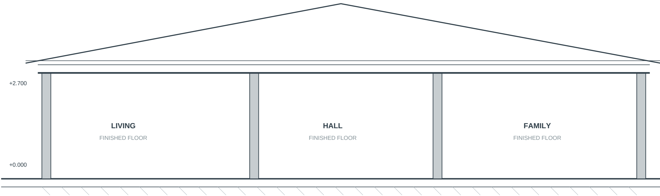
SECTION A-A
