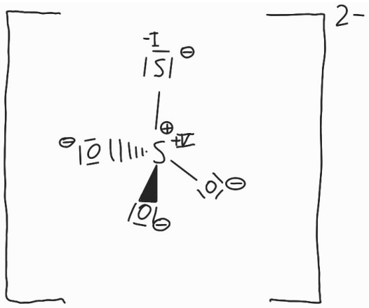
Abb. 1: Strukturformel des Thiosulfat-Ions
