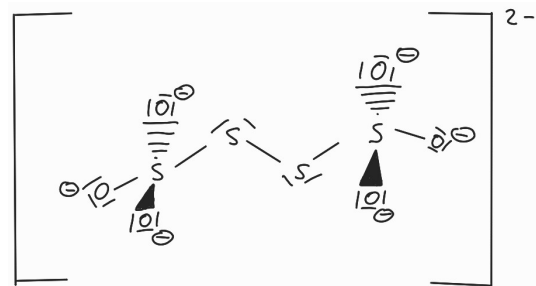
Abb. 2: Strukturformel des Tetrathionat-Ions
