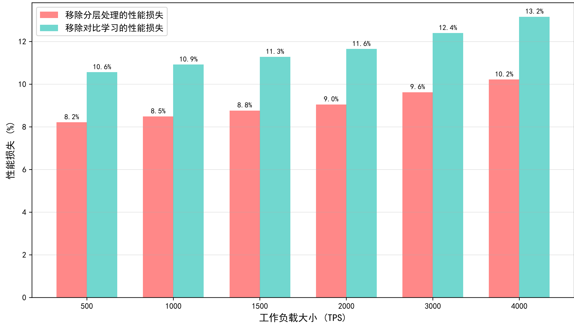
核心组件消融分析 - 性能损失量化
