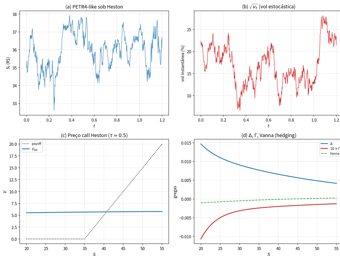
Figure 1: (a) S_t ; (b) vol; (c) preço; (d) gregas.
