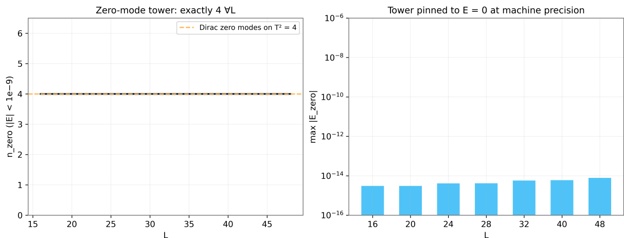
Рис. 2: Рис. 2. Тест D2. Слева: число нулевых мод по L -лестнице — ровно четыре моды при каждом размере (пунктир: дираковские нулевые моды на торе). Справа: максимальный |E| внутри башни — машинная точность (лог-шкала).
