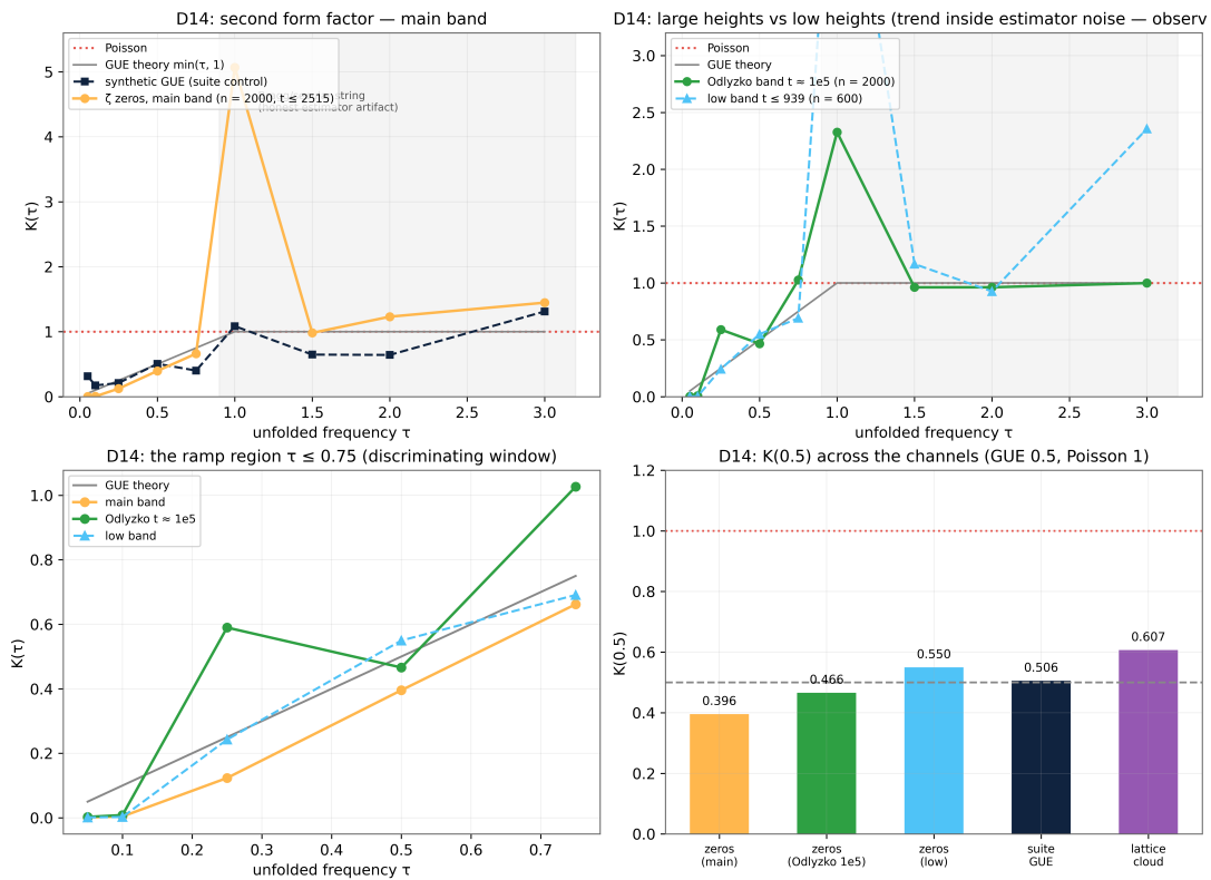
Рис. 14: Рисунок 14. Тест D14. Сверху слева: второй форм-фактор на основной полосе против GUE-теории, синтетического GUE-контроля сюта и пуассоновского уровня; струна оценщика при \tau = 1 затенена и аннотирована. Сверху справа: полоса Одлышко при t \sim 10^5 против низкой полосы — единичное плато уже точное на больших высотах. Снизу слева: рамповая область \tau \leq 0.75 по трём полосам. Снизу справа: K(0.5) по каналам — нули, синтетический GUE, решёточное облако.
