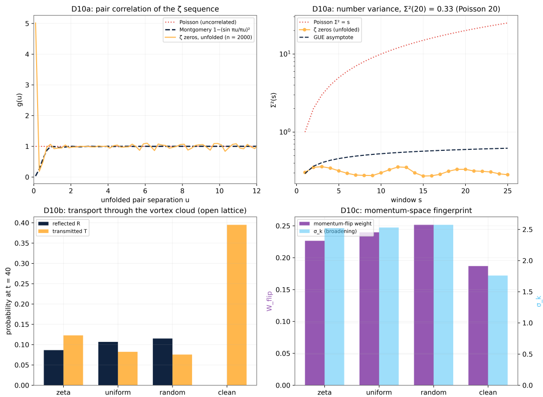
Рис. 10: Рис. 10. Тест D10. Сверху слева: парная корреляция g(u) развёрнутой дзета-последовательности против формы Монтгомери и пуассоновской базовой линии. Сверху справа: дисперсия числа \Sigma^2(s) — 0,33 при s = 20 против пуассоновских 20. Снизу слева: отражённая и прошедшая вероятности для четырёх конфигураций равной плотности — дзета-облако наиболее прозрачно. Снизу справа: импульсный отпечаток — вес переворота и уширение пакета, упорядоченные дзета < равномерное < Пуассон.
