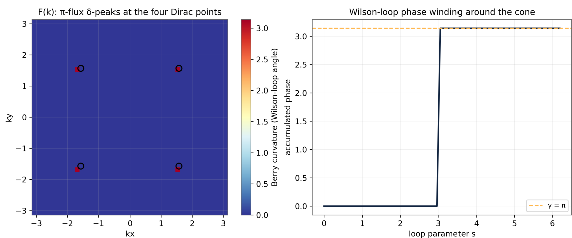
Рис. 3: Рис. 3. Тест D3. Слева: берриевская кривизна решётки из ячейечных петель Вильсона — четыре пи-флюкс пика в дираковских точках (обведены), полное число Черна нуль. Справа: накопленная фаза петли Вильсона по окружности r = 0.2 вокруг конуса — навивка достигает ровно \pi .
