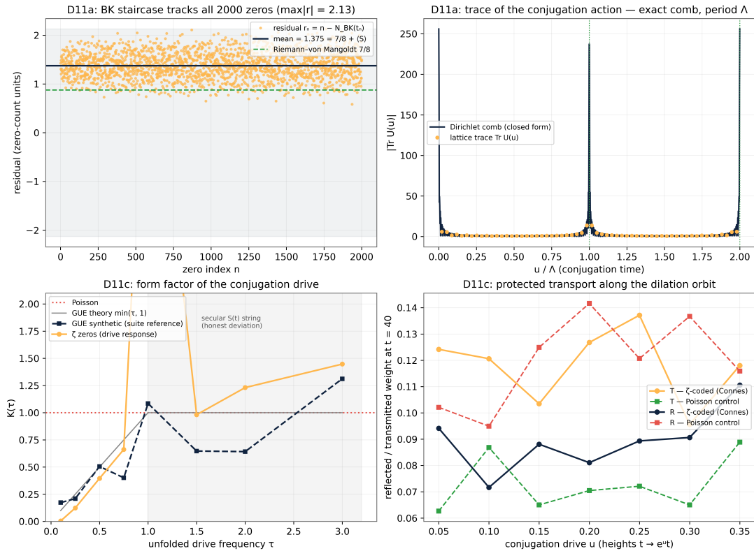
Рис. 11: Рисунок 11. Тест D11. Сверху слева: остаток лестницы Берри–Китинга r_n = n - (t_n/2\pi) \cdot \ln(t_n/2\pi e) по реальной лестнице нулей — среднее 1,3750 ( 7/8 + \langle S \rangle ), максимум 2,13. Сверху справа: след действия сопряжения против замкнутой гребёнки Дирихле, два точных периода \Lambda . Снизу слева: форм-фактор драйва K(\tau) — нули дзеты против синтетического GUE-справочника сюиты и пуассоновской прямой; заштрихованная область \tau \geq 1 несёт светскую струну S(t) (документировано). Снизу справа: транспорт под сопрягающим драйвом t \rightarrow e^u t — дзета-кодированное облако сохраняет защищённый класс вдоль всей орбиты.
