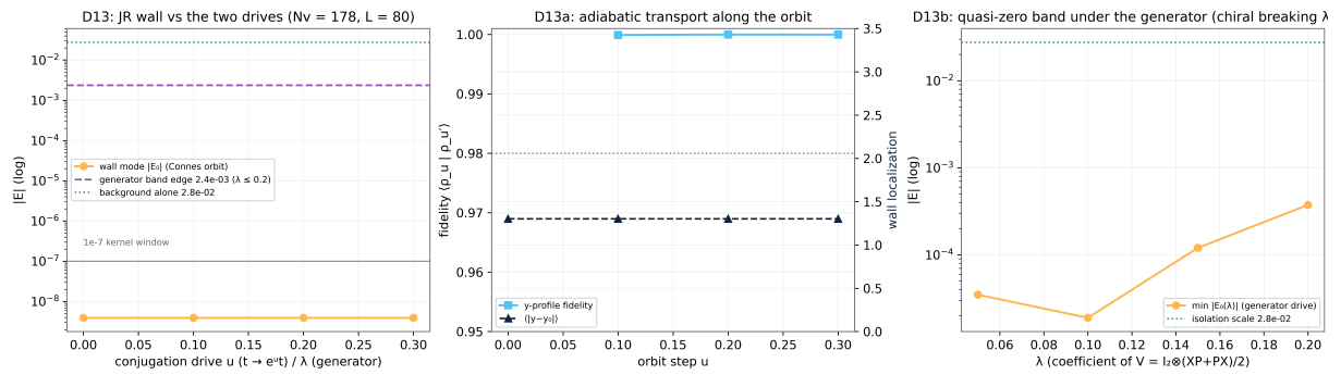
Рис. 13: Рисунок 13. Тест D13. Слева: энергия моды стенки под обоими драйверами — заякорена на 3,9 \cdot 10^{-9} вдоль коннесовской орбиты, приподнята лишь до \text{gar}/679 генератором при \lambda = 0.2 ; отмечены фоновый контроль и кернел-окно 10^{-7} . В центре: адиабатический транспорт вдоль орбиты (точность у-профиля и локализация на стенке). Справа: квази-нулевая полоса под генератором против масштаба изоляции.
