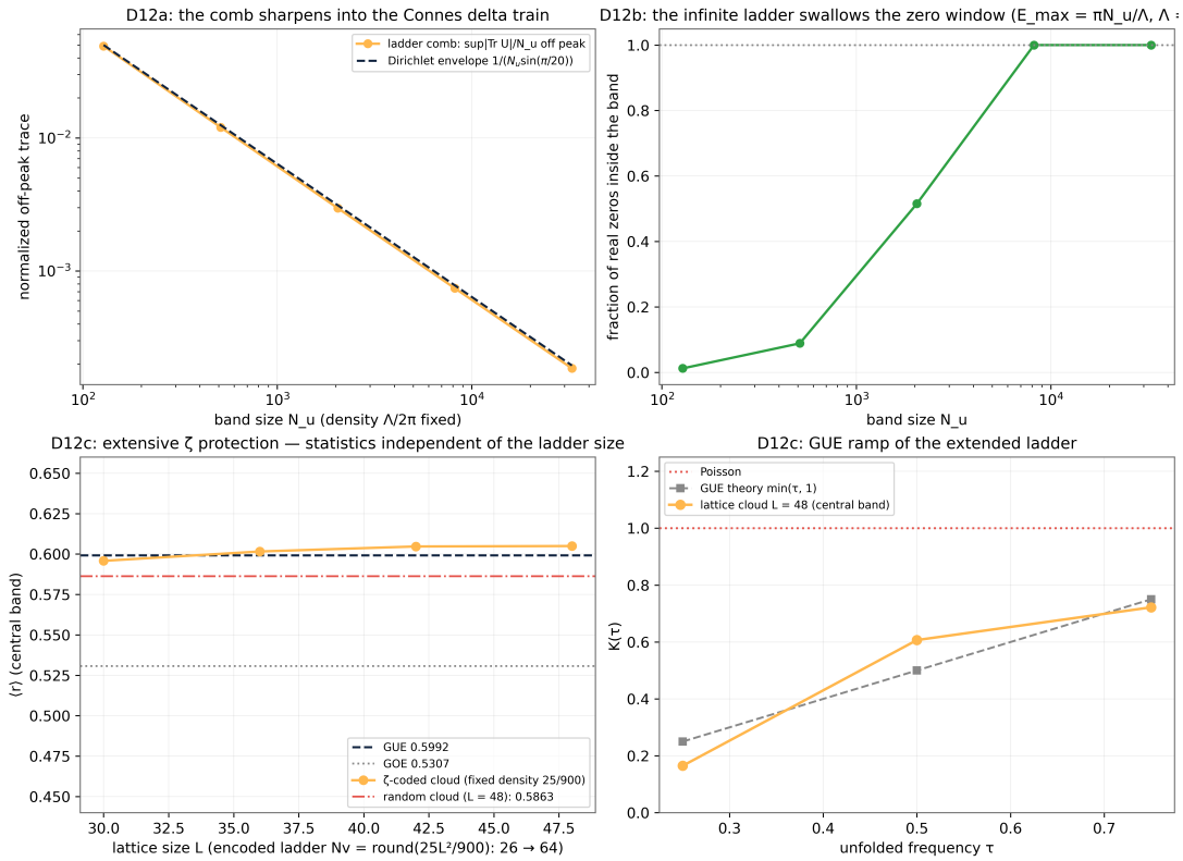
Рис. 12: Рисунок 12. Тест D12. Сверху слева: вне-пиковый след действия сопряжения следует дирихлевской огибающей 1/(N_u \cdot \sin(\pi/20)) через два порядка размера полосы — гребёнка заостряется в дельта-поезд Коннеса. Сверху справа: расширяющаяся полоса поглощает окно реальных нулей (покрытие = 1 при N_u = 8192 ). Снизу слева: GUE-статистика не зависит от L при фиксированной плотности вихрей, пока закодированная лестница растёт N_v = 25 \rightarrow 64 (показаны чистый и случайный базлайны). Снизу справа: GUE-рампа форм-фактора облака L = 48 .
