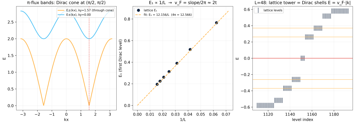
Рис. 1: Рис. 1. Тест D1. Слева: пи-флюкс зоны E_{\pm}(k) вдоль сечения через дираковскую точку (\pi/2, \pi/2) . В центре: финально-размерный скейлинг E_1 против 1/L с линейным фитом (наклон 12.156, R-квадрат 0.99989); континуальный прогноз — E_1 \times L = 2\pi v_F = 4\pi . Справа: низкоэнергетический спектр тора L = 48 против аналитических дираковских оболочек (горизонтальные линии) — башня решётки есть дираковский спектр уровня за уровнем.
