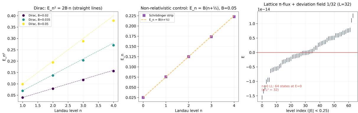
Рис. 4: Рис. 4. Тест D4. Слева: дираковские ландау-лестницы E_n -квадрат против n для трёх полей — прямые через начало координат с наклонами, совпадающими с 2 v_F -квадрат B . В центре: шрёдингеровская контрольная лестница E_n = B(n + 1/2) на том же стрипе. Справа: решёточная пи-флюкс модель с полем отклонения 1/q — киральный ландау-уровень n = 0 , приколотый к E = 0 .
