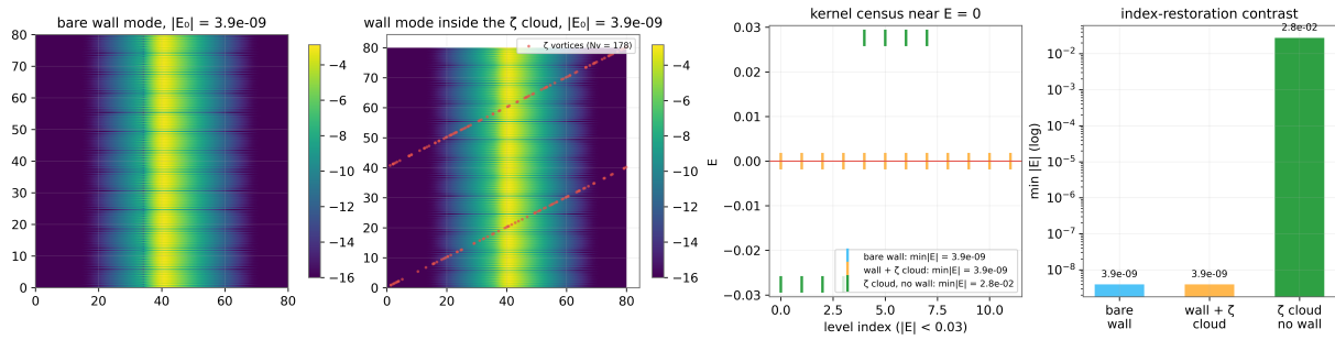
Рис. 9: Рис. 9. Тест D9. Слева: плотность моды стенки (лог-шкала) для чистой стенки Джекива–Рибби, |E_0| = 3,9 \cdot 10^{-9} . Слева в центре: та же мода в полном дзета-вихревом фоне ( N_v = 178 , красные точки) — без изменений. Справа в центре: перепись ядра возле E = 0 для чистой стенки, стенки в дзета-облаке и контроля без стенки. Справа: контраст восстановления в лог-шкале — стенка привлекает нулевую моду в 7 \cdot 10^6 раз ниже голого фонового сектора.
