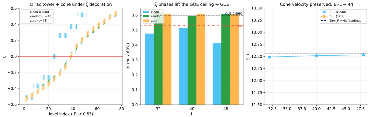
Рис. 7: Рис. 7. Тест D7. Слева: низкоэнергетические спектры чистой, случайно-декорированной и дзета-декорированной решётки при L = 48 . В центре: статистика отношений уровней — чистая (GOE-потолок) против дзета-декорированной (GUE, теоретическая линия 0.5992). Справа: масштаб конуса E_1 \times L против континуального значения 4\pi .
