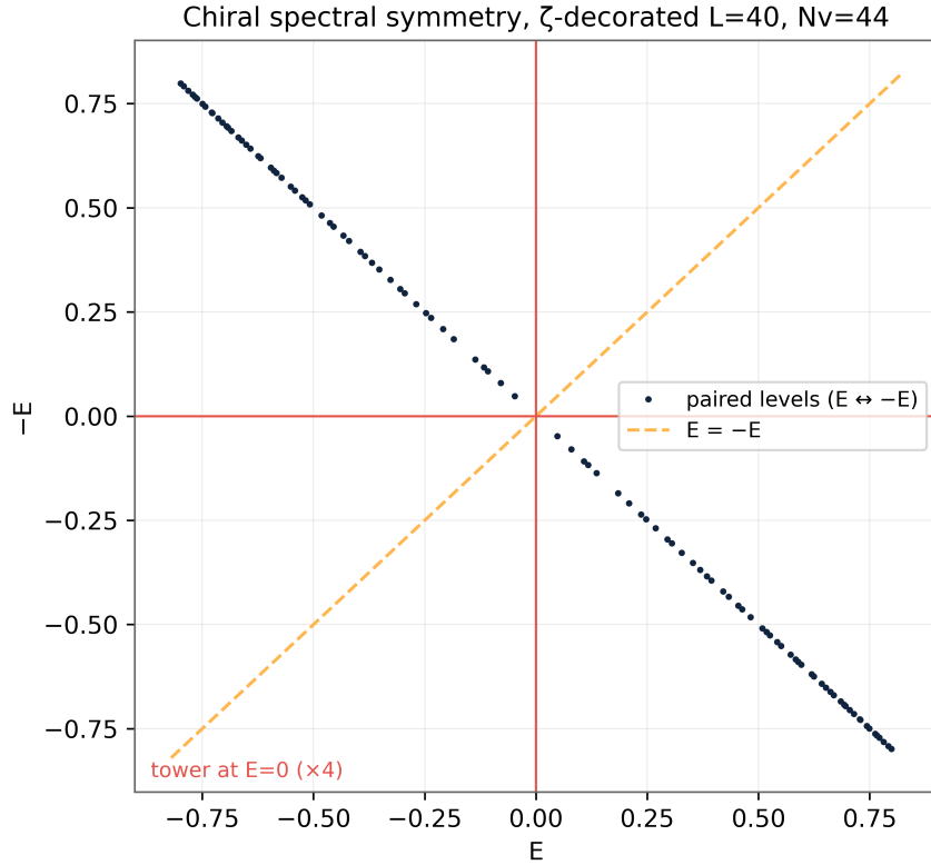
Рис. 8: Рис. 8. Тест D8. Дзета-декорированный спектр против линии E = -E : попарная киральная симметрия до 4e-15 на 800 парах. Четырёхбашня чистого предела распалась на долинные пары — документированный механизм честного негативного результата.
